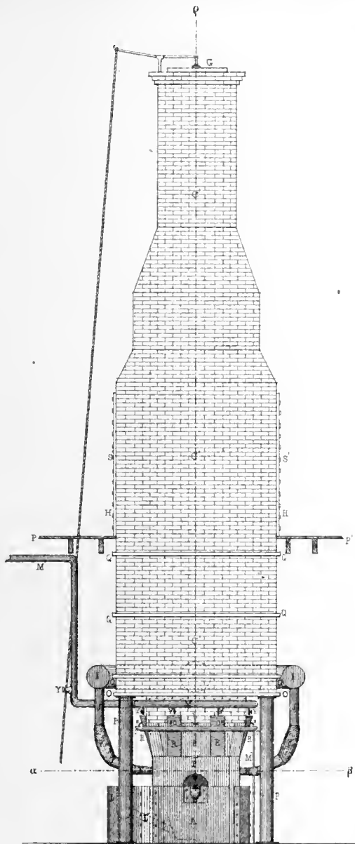
Fig. 1. ELEVATION
