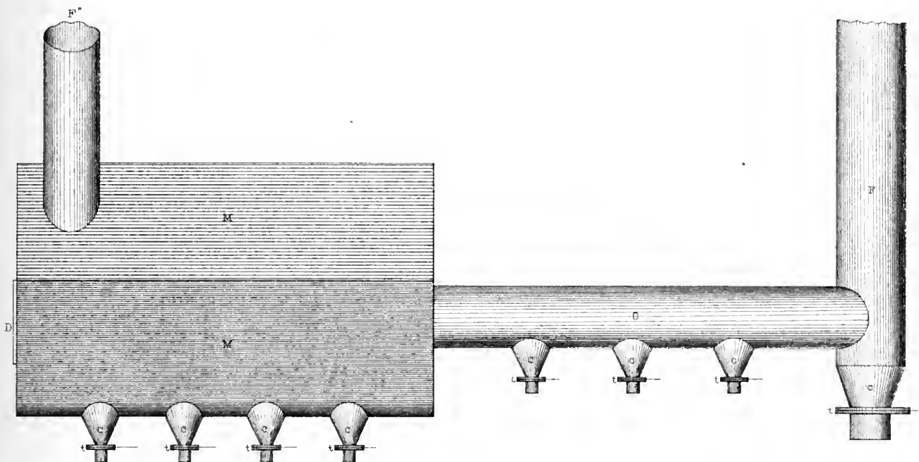
Fig. 1, SIDE ELEVATION
