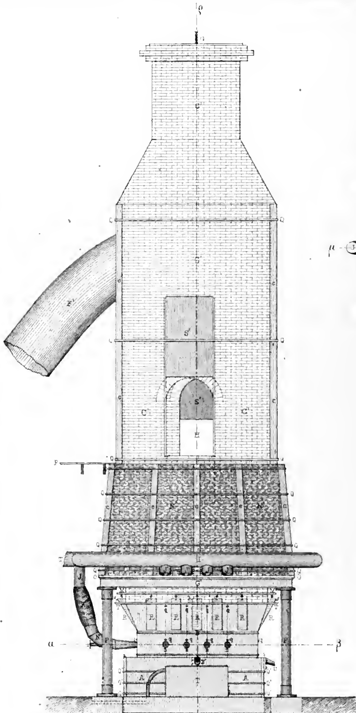
Fig. 1 ELEVATION
