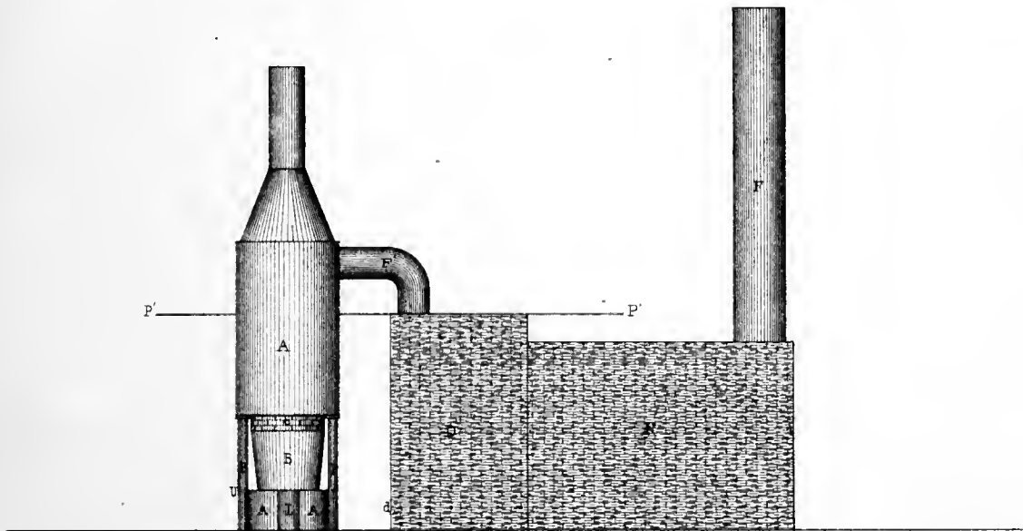
Fig. 1 SIDE ELEVATION
