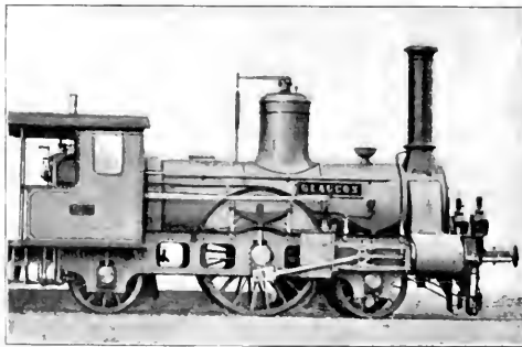
Abb. 300. Schnellzug-Locomotive der Nordbahn. [1874.]
