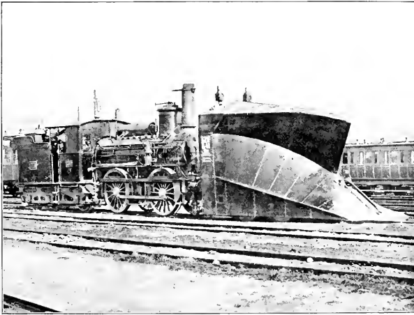
Abb. 399. Schneepflug [Nach einer Original-Aufnahme von A. Steimpl]
