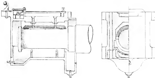
Abb. 319. Achsager der Kaiser Ferdinands-Nordbahn. [1854.]
