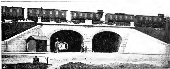
Abb. 134. Gewölbte Durchfahrt aus Stampfbeton auf dem Brüner Nordbahnhofe. [Kaiser Ferdinands-Nordbahn.]
