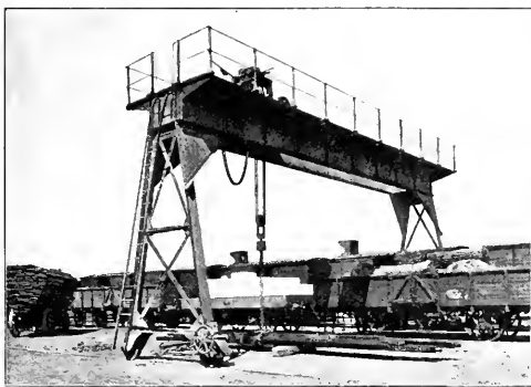
Abb. 201. Kran für schwere Lasten auf dem Frachtenbahnhof Matzleinsdorf.
