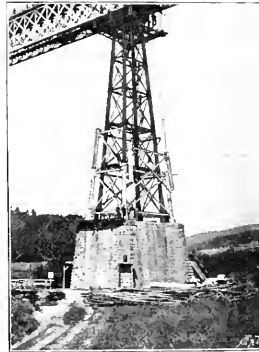
Abb. 109. Reconstruction der Iglawa-Brücke. [Auswechslung der Gusseisenpfeiler.]
