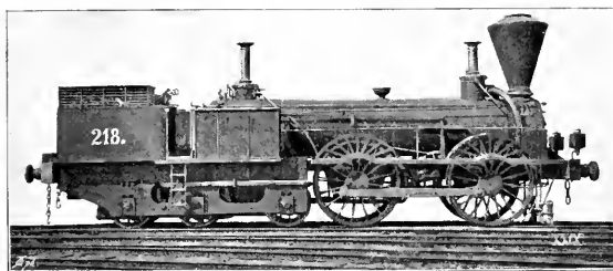
Abb. 285. Engerth-Locomotive der südlichen Staatsbahn. [1856.]
