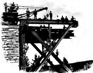
Abb. 159b. Montirung der Moldaubrücke bei Cervena.
