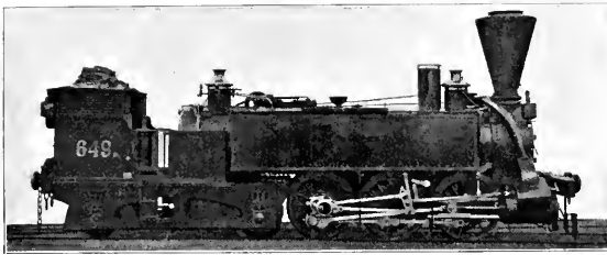
Abb. 283. Engerth-Locomotive der südlichen Staatsbahn. [1854.]
