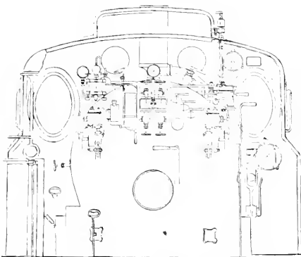
Abb. 308 Anordnung der Apparate bei einer Locomotive neuerer Type
