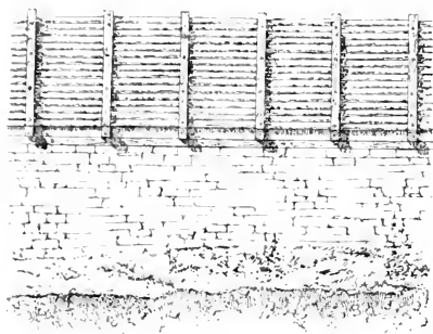
Abb. 51. Anlagen zum Schutze gegen kleinere Felsen- und Geröllstücke. Brennerbahn.
