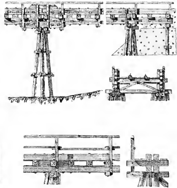
Abb. 130. Construction der Klötzeholzbrücken von Pressel.
