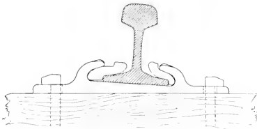
Abb. 122. Kremenplatte. [System Hohenegger.]
