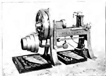
Abb. 188. Schraubenschneidmaschine. System Schellers.]
