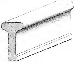
Abb. 104. Hochschiene (Raül). [Kaiser Ferdinands-Nordbahn, 1838.]
