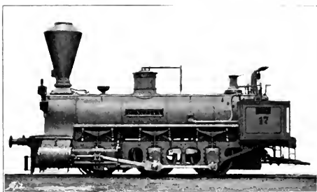
Abb. 202. Güterzug-Locomotive der Carl Ludwig-Bahn. [1859.]
