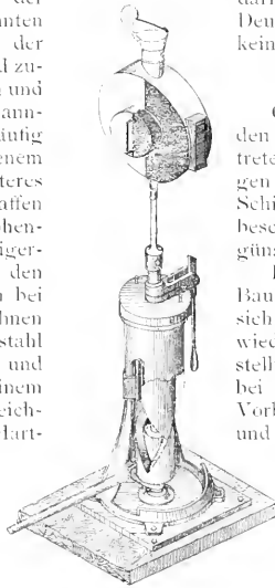
Abb. 121 b. Weichenconstruction der Semmeringbahn, 1851 [Wechselständer.]
