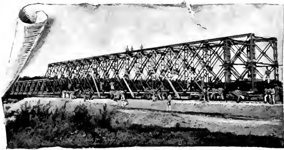
Abb. 30. Kohlenbrücke.
