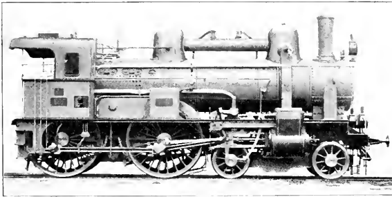
Abb. 308. Verbund-Schnellzug-Locomotive Serie 0 der k. k. Staatsbahnen. [1894.]
