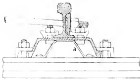
Abb. 113. Eisernes Oberbahnsystem. [System Hohenegger, 1879.]
