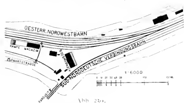
STATION ALT-PAKA DER OESTERR. NORDWESTBAHN UND SUD-NORDDEUTSCHEN VERBINDUNGSBAHN 1872.
