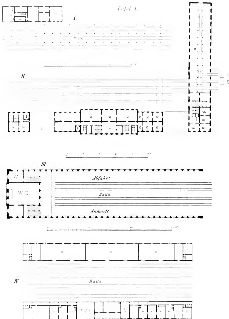
I. Station (1850). II. Aufnahmegebäude, Wien der Nordbahn (1850). III. Aufnahmegebäude, Wien-Gloggnitz (1852). IV. Aufnahmegebäude Olmütz der Nordbahn (1852).
