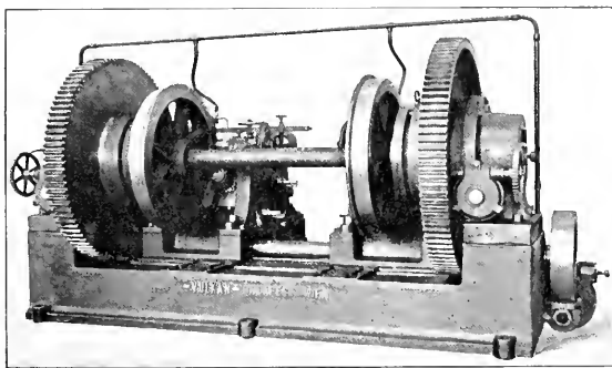
Abb. 313. Doppelte Tyres-Rollmaschine.
