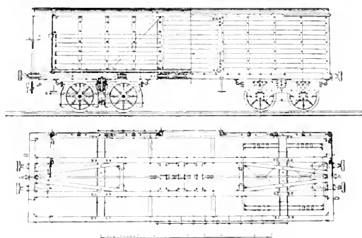
Abb. 305. Erster in der Fabrik von F. Ringhoffer gebauter Wagen. [1852.]
