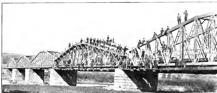
Abb. 148. Reconstruction der Dniesterbrücke bei Niznlów, [Stanislaw-Huslatyn.]
