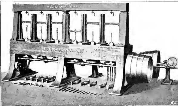
Abb. 387. Mutterschneidmaschine.
