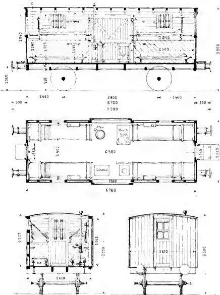
Abb. 350 Eisenbahn-Sanitätswagen [1877]
