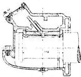
Abb. 320 Oellager der Kaiser Franz Josef-Bahn. [1872]
