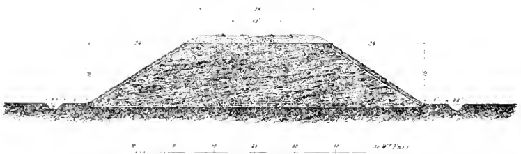
Abb. 63. Dämmprofil der Nordbahn [1857.]
