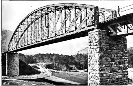
Abb. 152. Brücke über die Oetzthaler Aache. [Innsbruck-Landeck.] [Nach einer photographischen Aufnahme von C. A. Czichna, Innsbruck.]
