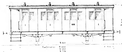
Abb. 332. Localzugwagen. (1875.)
