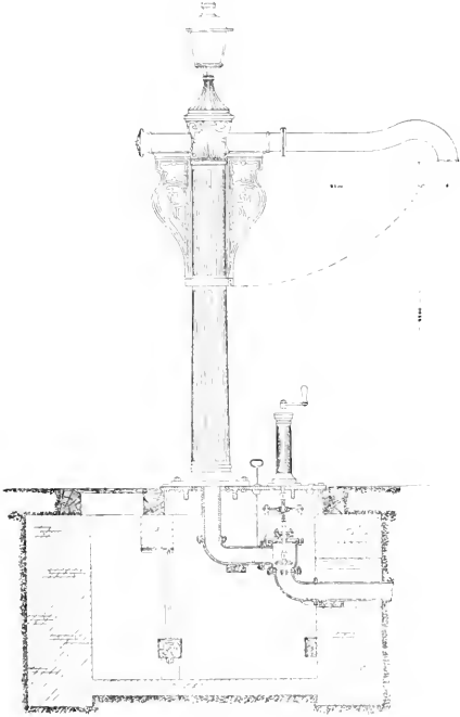
Abb. 397. Säulenkrahn älterer Typs.
