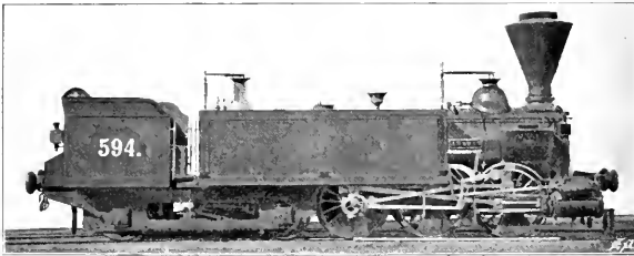
Abb. 284. Engerth-Loomotive der südlichen Staatsbahn. [1869.]
