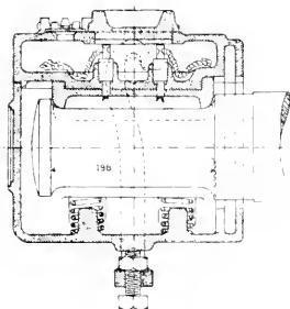
Abb. 322. Achslager der k. k. Staatsbahnen [1874]
