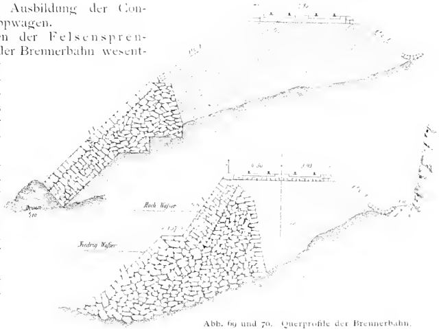
Abb. 69 und 70. Querprofile der Bremerbahn.
