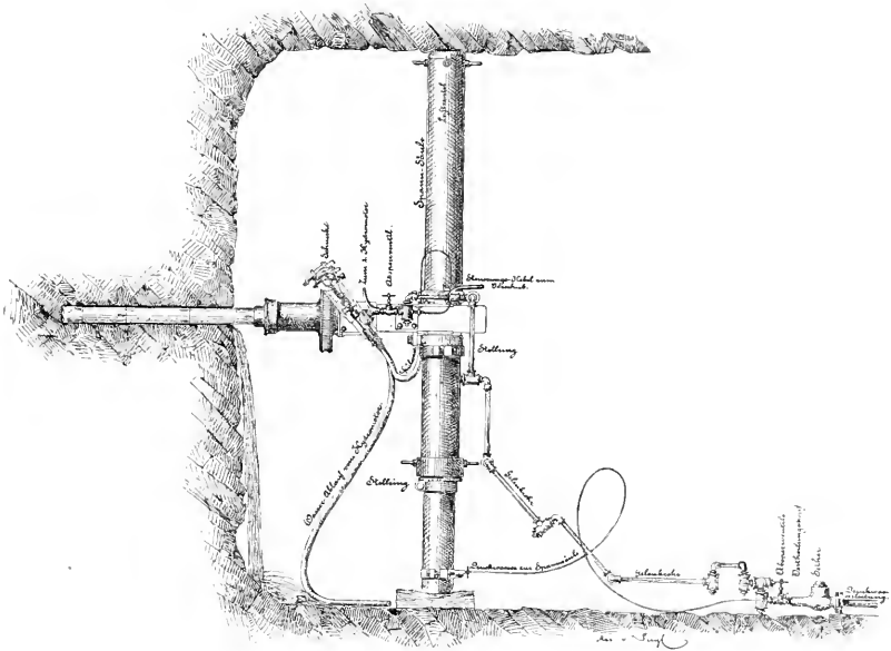
Abb. 07. Bohrmaschine nach Brandt's System.
