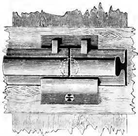
Abb. 105. Oberbau mit breitfüssigen Schienen [Wien-Gloggnitz, 1841.]
