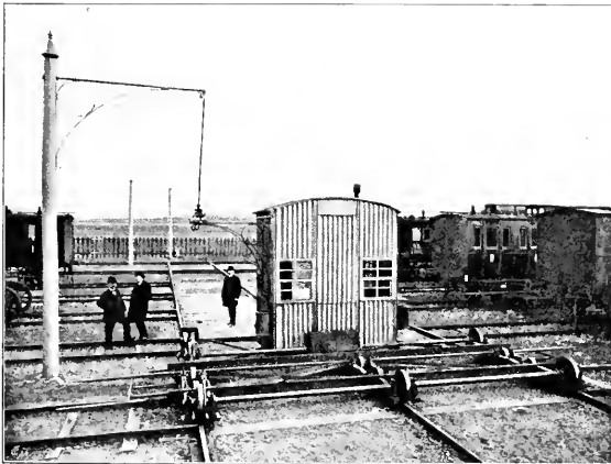
Abb. 353. Wagenschiebephöhne mit elektrischem Antrieb
