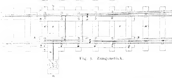
Abb. 124. Weichenconstruction der Semmeringbahn [1851]
