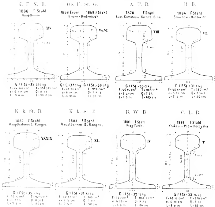
Abb. 1. Schnittprofile der österreichischen Eisenbahnen am 1. Januar 1888.
