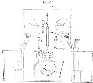
Abb. 301. Anordnung der Apparate bei einer Locomotive älterer Type.
