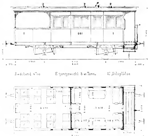
Abb. 318. Aussichtswagen der Kaiserin Elisabeth-Bahn.
