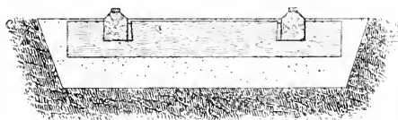
Fig. 3. Querschnitt. Abb. 102. Oberbau mit Flachschienen.
