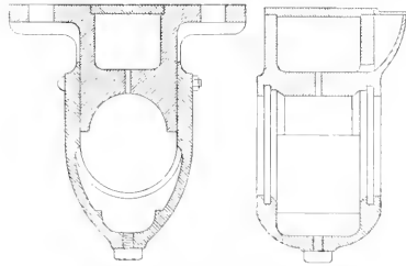
Abb. 317. Achslager der Pferdebahn Prag-Lana. [1880.]
