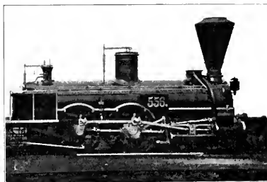
Abb. 296. Personenzug-Locomotive der Südbahn. [1891.]
