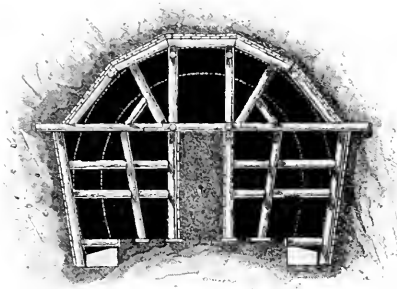
Abb. 89. Bau des Kerschbacher Tunnels [südl. Staatsbahn]
