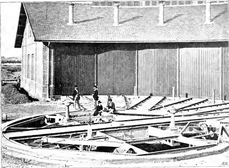
Abb. 100. Locomotiv-Drehscheibe auf dem Wiener Nordwestbahnhote.
