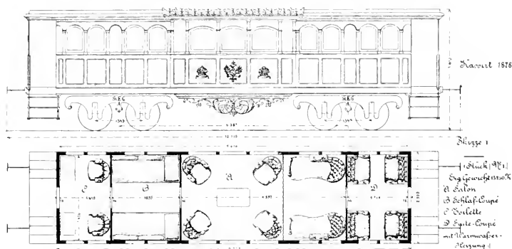
Abb. 349. Hofwagen der Staatsbahnen. [1876]
