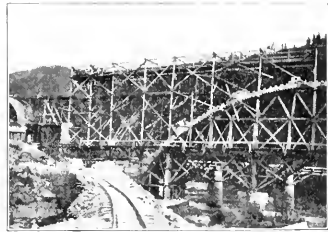
Abb. 133b. Pruthbrücke bei Jaremeze im Bau. [Erste Steinschar.]
