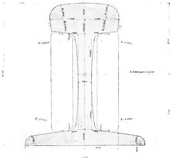
Abb. 110. Normalprofil des Oesterreichischen Ingenieur- und Architekten-Vereines [1895].
