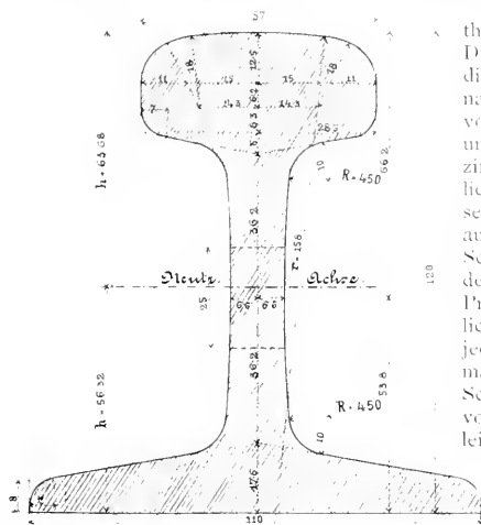
Abb. 108. Schienenprofil A der Nordbahn [eingeführt 1860]. Querschnittsfläche = 39 505 \text{mm}^2 , Gewicht pro 1 m in Schweiss- stahl = 30 810 kg, Gewicht pro 1 m in Flussstahl = 31 080 kg. Trägheitsmoment T = 706 080 für cm, Widerstandsmoment W = 120 302 für \text{cm}^3 .
