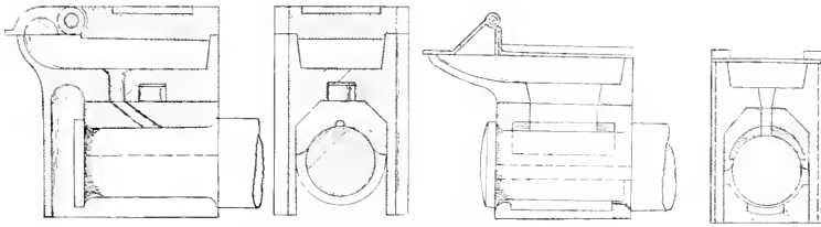
Abb. 318. Achsager der k. k. Staatsbahnen. [1844.]
