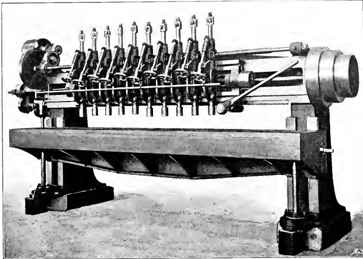
Abb. 356. Bohrmaschine mit zehn Bohrspindeln.
