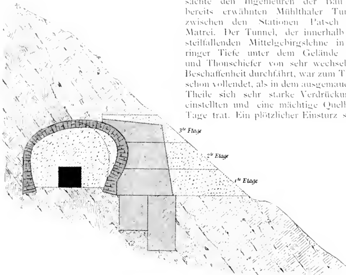
Abb. 91. Reconstruction des Mühlthaler Tunnels. [Brennerbahn.]
