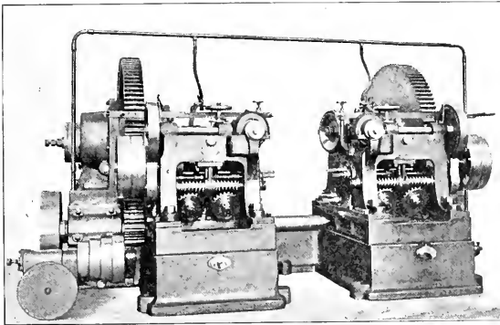
Abb. 392. Doppelte Tyres-Fräsmaschine.
