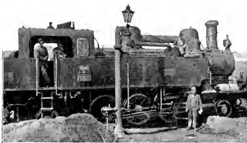
Abb. 399. Locomotive bei der Ausrüstung.
