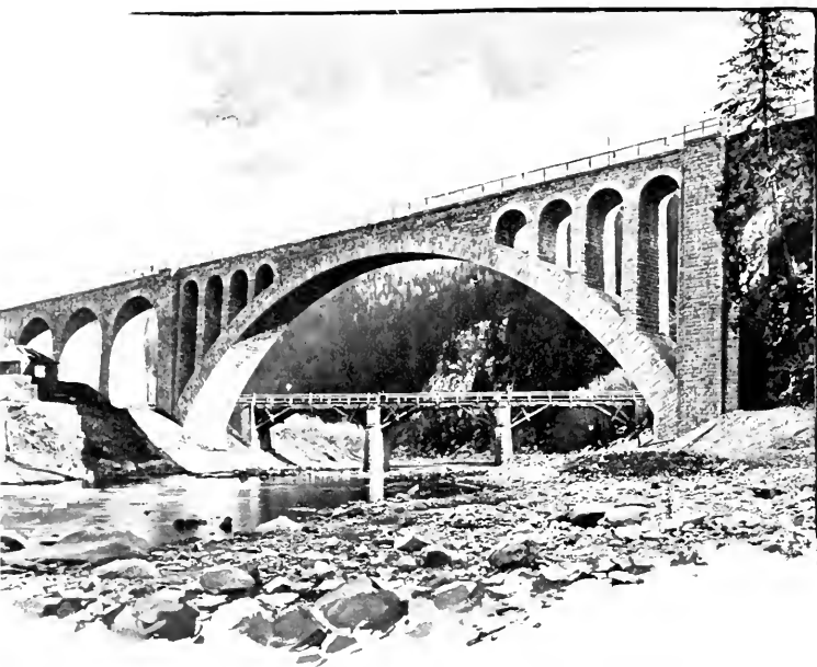
Abb. 133a. Brücke bei Jaremeze [K. k. Staatsbahn Stanislaw-Woronienka]
