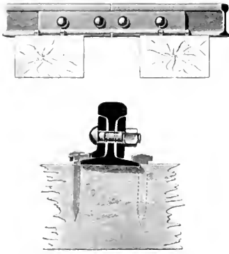
Abb. 110. Schwebender Stoss. Kaiser Ferdinands-Nordbahn 1870
