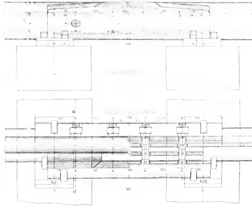
Stossverbindung mit Stossfangschiene 1:5
