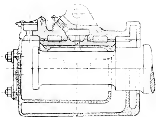
Abb. 321 Paget-Lager. [1858]
