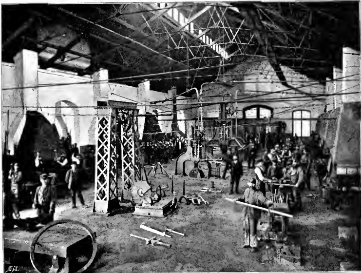
Abb. 378. Werkstätte Neu-Sandec der k. k. Oesterreichischen Staatsbahnen. [Schmiede-Werkstätte]
