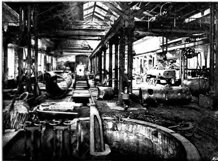
Abb. 308. Werkstätte Linz der k. k. österreichischen Staatsbahnen. [Kesselschmiede, im Vordergrund Seitenansicht der feststehenden hydraulischen Nietmaschine.]
