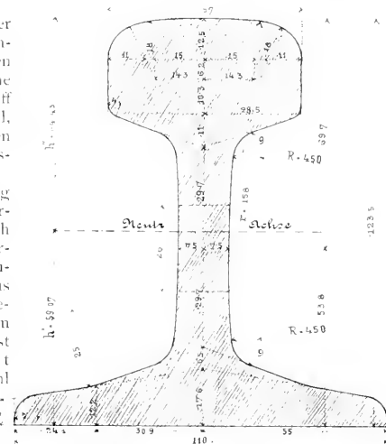
Abb. 109. Schienenprofil B der Nordbahn [eingeführt 1872]. Querschnittsfläche = 41 770 \text{mm}^2 , Gewicht pro 1 m in Schweiss- stahl = 31 090 kg, Gewicht pro 1 m in Flussstahl = 35 230 kg. Trägheitsmoment T = 877 490 für \text{cm}^3 , Widerstandsmoment W = 130 993 für \text{cm}^3 .
