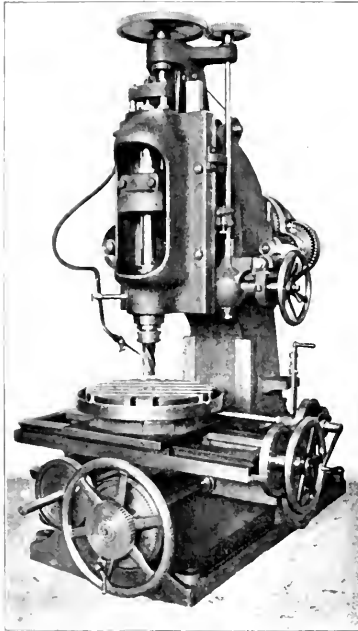
Abb. 390. Dampfbetriebene, selbstthätige Fräsmaschine.
