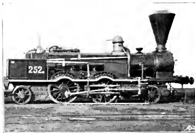
Abb. 280. Personenzug-Locomotive der südlichen Staatsbahn. [1857.]
