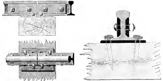
Abb. 117. Laschenverbindung beim Oberbau der Kaiserin Elisabeth-Bahn. [1885.]
