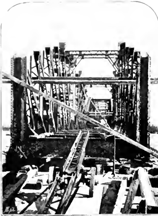
Abb. 153b Isuzo-Brücke, Montalcone-Cervignano.)
