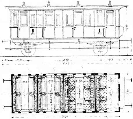
Abb. 320. Personenwagen mit Halb-Coupe und Schlafsitzen. [1870.]
