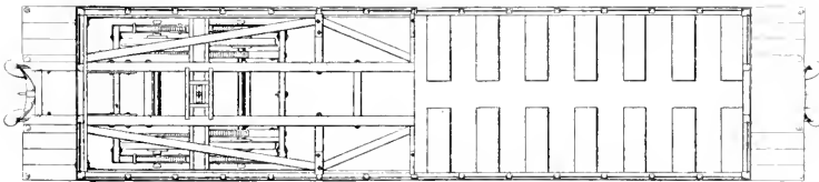
Abb. 325 c. Wagen III. Classe für 72 Personen.
