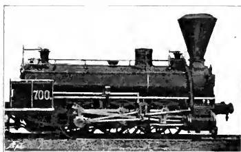
Abb. 298. Güterzug-Locomotive der südlichen Staatsbahn. [1890.]
