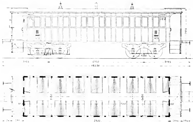
Abb. 330. Personenwagen III. Classe der nördlichen Staatsbahnen 1870.
