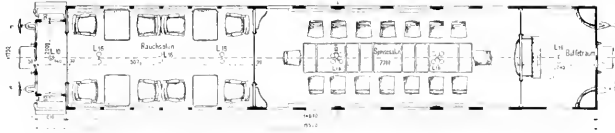
Abb. 348. Speisewagen des Kaiserzuges.
