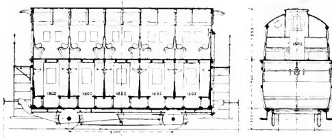
Abb. 351. Etagewagen. [1870.]
