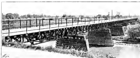
Abb. 107. Brücke über den Mitterbach [Schwechhat-Mannersdorf]
