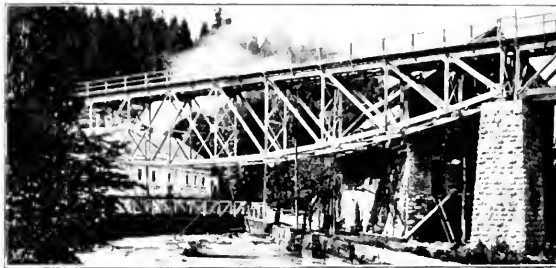
Abb. 157. Brücke bei Wardhofen. [Ybbsthal-Bahn]
