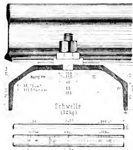
Abb. 116. Eiserner Querschwellen-Oberbau. [System Heindl, 1882.]
