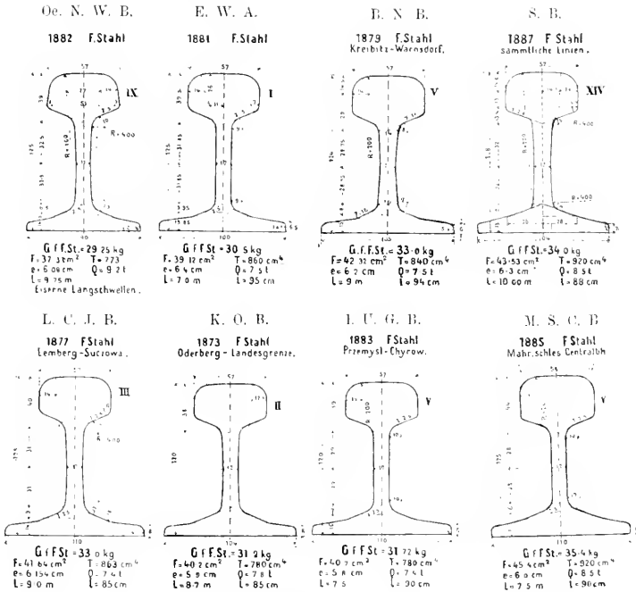
Abb. 111b. Schienenprofile der österreichischen Eisenbahnen (aus J. Lamm 1888).
