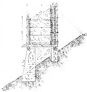
Abb. 51. Anlagen zum Schutze gegen kleinere Felsen- und Geröllstücke. Brennerbahn.
