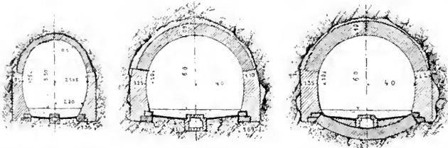
Abb. 101. Tunnelprofil der Arlbergbahn.
