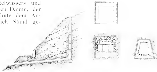
Abb. 71. Entwässerungs-Anlage auf der Brennerbahn. [Querschnitt und Einzeltheile.]
