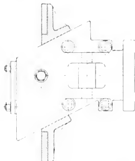
Abb. 312. Achsbüchse von Adams. [1851.]
