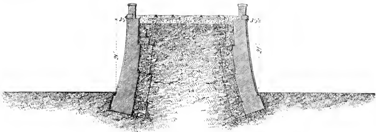
Abb. 64. Profil mit Stützmauern. [Nordbahn, 1857.]
