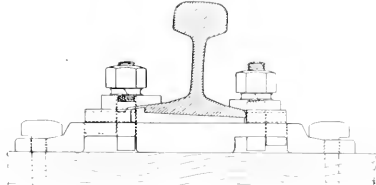
Abb. 123. Stuhlplatte. [System Heindl.]
