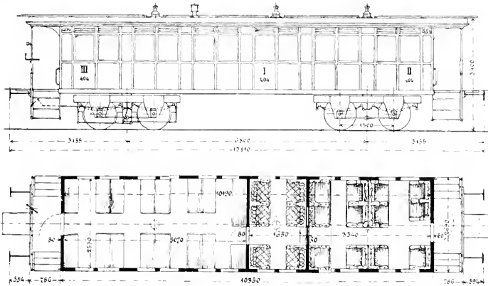
Abb. 331. Personenwagen I., II., und III. Classe der nördlichen Staatsbahnen [1870]
