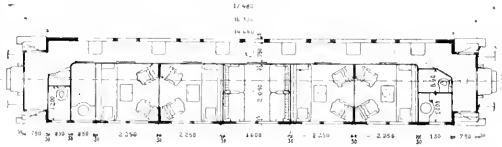
Abb. 342. Luxuszug-Wagen. [1895.]
