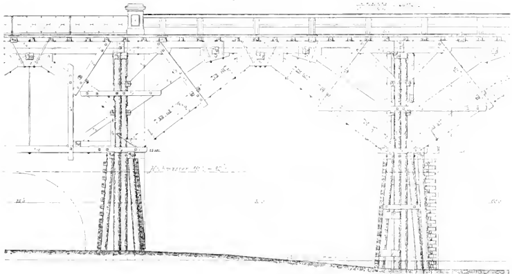
Abb. 143. Holzprovisorium der Inundationsbrücke bei Stadlau.
