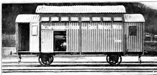
Abb. 391. Imprägnierungswagen.
