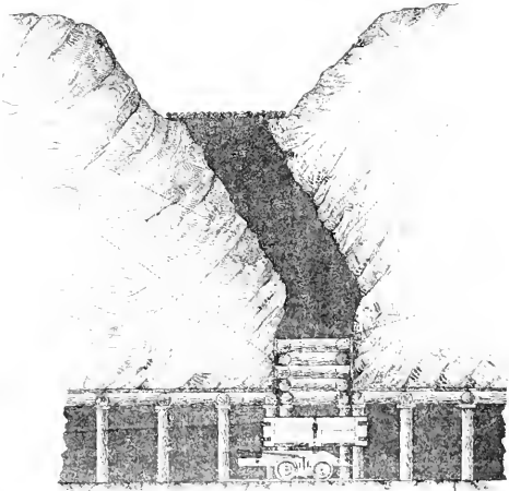
Abb. 75. Englischer Einschnittbetrieb.
