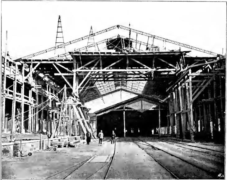
Abb. 297. Die Halle des Wiener Südbahnhotes in Unbau begriffen. [1870.]
