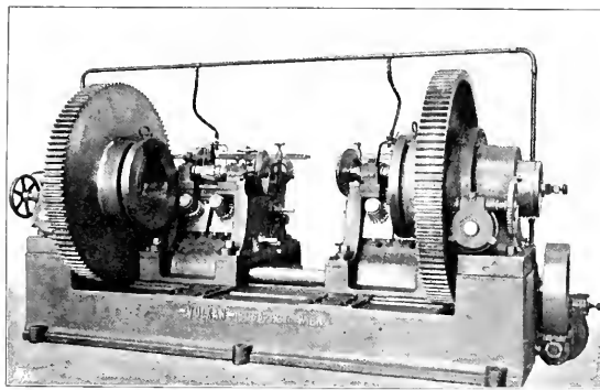
Abb. 301. Doppelte Tyres-Fräsmaschine.
