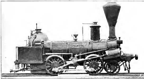
Abb. 282. Güterzug-Locomotive der Nordbahn. [1844.]
