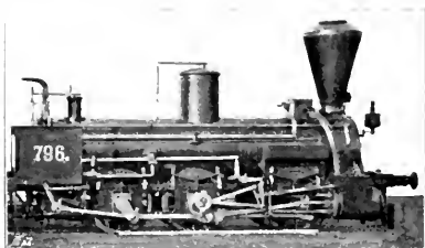
Abb. 298. Güterzug-Locomotive der Kaiser Franz Josef-Orient-Bahn. [1869.]
