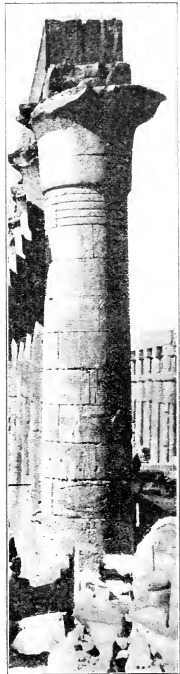
Abb. 39: Offene Papyrusdolden-Einzelsäule. Zeit Amenophis' III. (Luxor).
