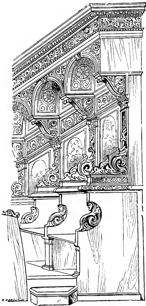
Abb. 303. Chorstühle aus S. Giovanni in Parma. (Nohl.)
