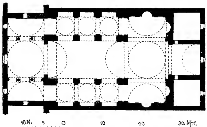
Abb. 161. Annunziata zu Arezzo. Grundriß. (Gnauth.)
