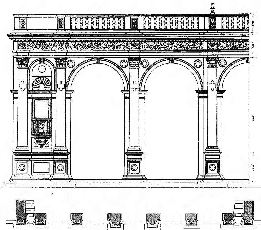
Abb. 130. Von der Vorhalle des Domes zu Spoleto. (Nach Bühlmann.)
