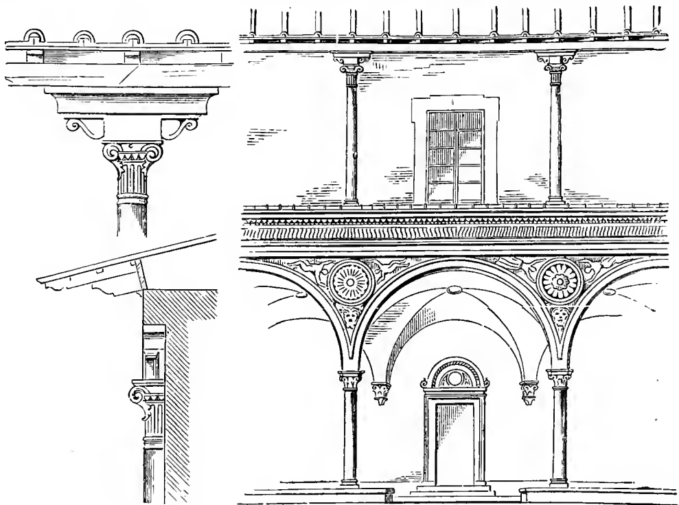
Abb. 14. Hof bei S. Croce zu Florenz.
