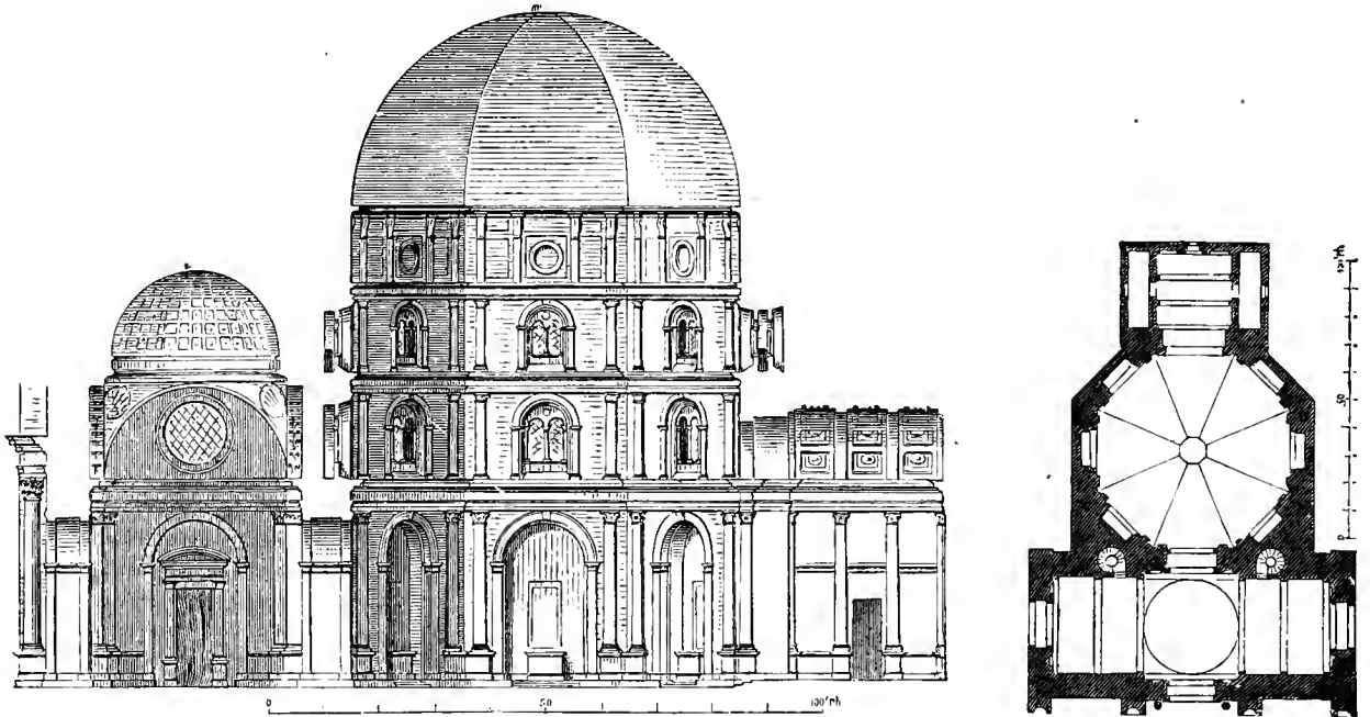
Abb. 94 und 95. Madonna dell' Umiltà zu Pistoja. Durchschnitt. (J. Stadler.) Grundriß.
