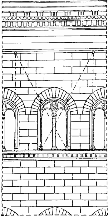
Abb. 77. Vom Pal. Strozzi zu Florenz. (Nach A. Thiersch im Handb. d. Archit.)
