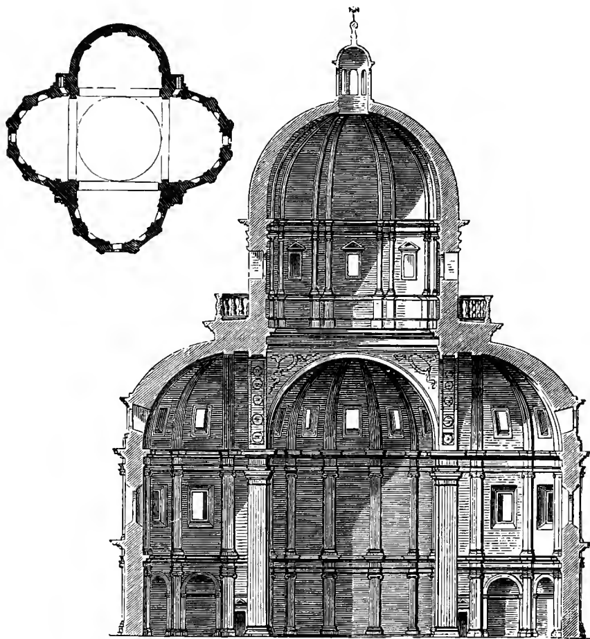
Abb. 109 und 110. Consolazione zu Todi.
