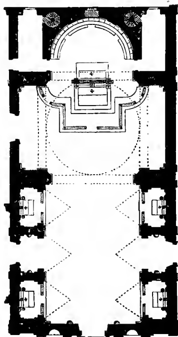
Abb. 155. S. Maria de' Monti. (Nach Letarouilly.)
