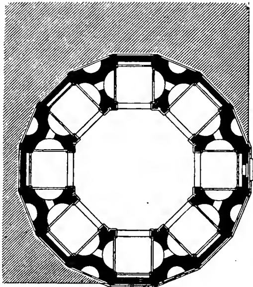
Abb. 86. S. Maria degli Angeli zu Florenz.
