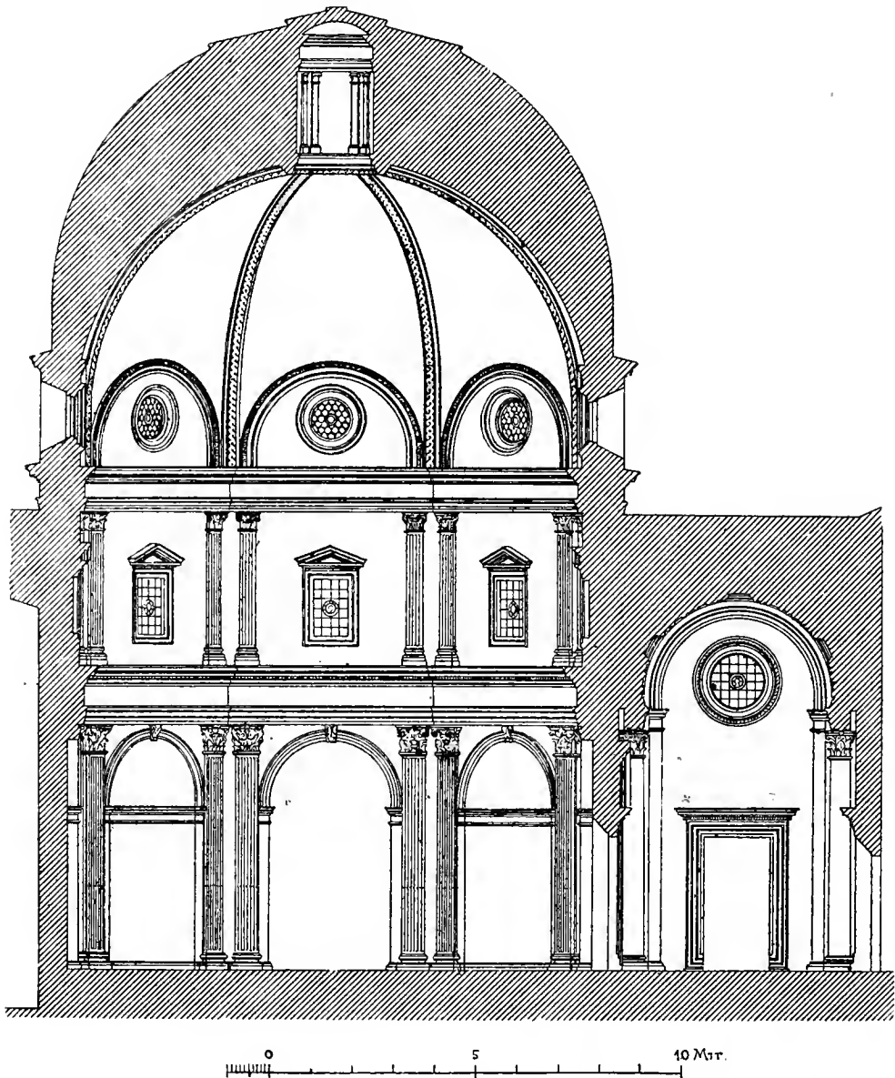
Abb. 175. Sakristei von S. Spirito zu Florenz. Durchschnitt. (Nach Mayreder.)
