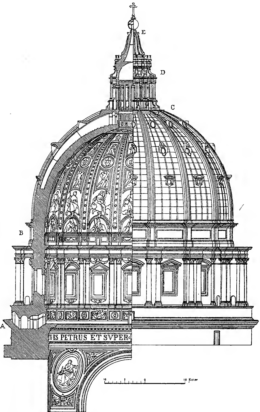
Abb. 108. Kuppel von St. Peter zu Rom. (Nach Bühlmann.)
