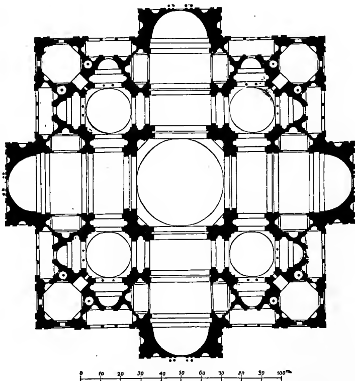
Abb. 104. St. Peter. Bramantes erster Grundriß.
