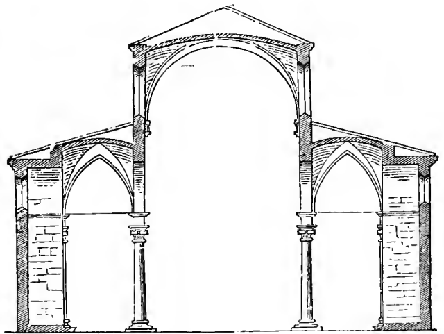
Abb. 143. Servi zu Siena. Querschnitt. (L.)
