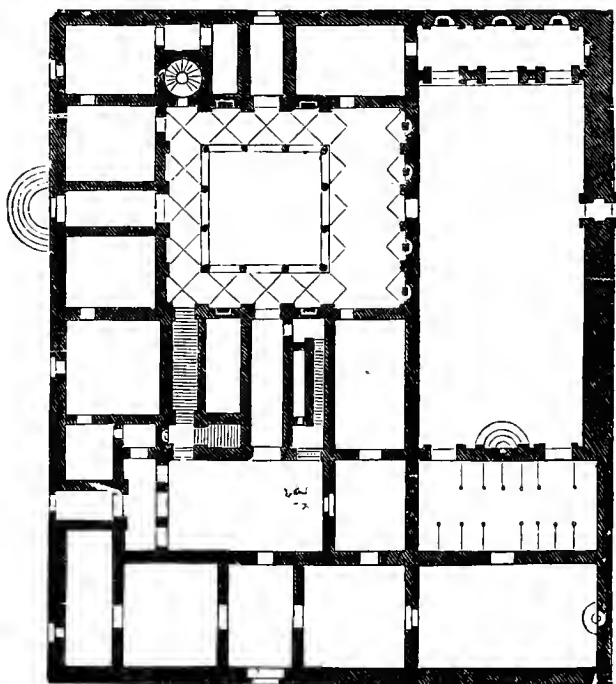
Abb. 192. Pal. Riccardi zu Florenz. Grundriß.
