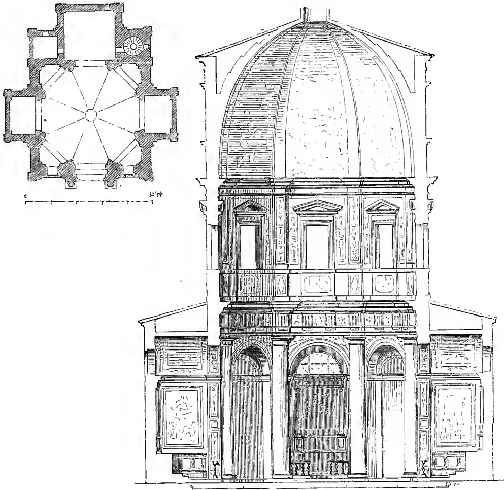
Abb. 117 und 118. S. Croce bei Riva.
