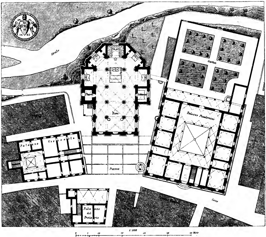
Abb. 193. Dom und Paläste zu Pienza. Grundriß. (Nach Mayreder.)
