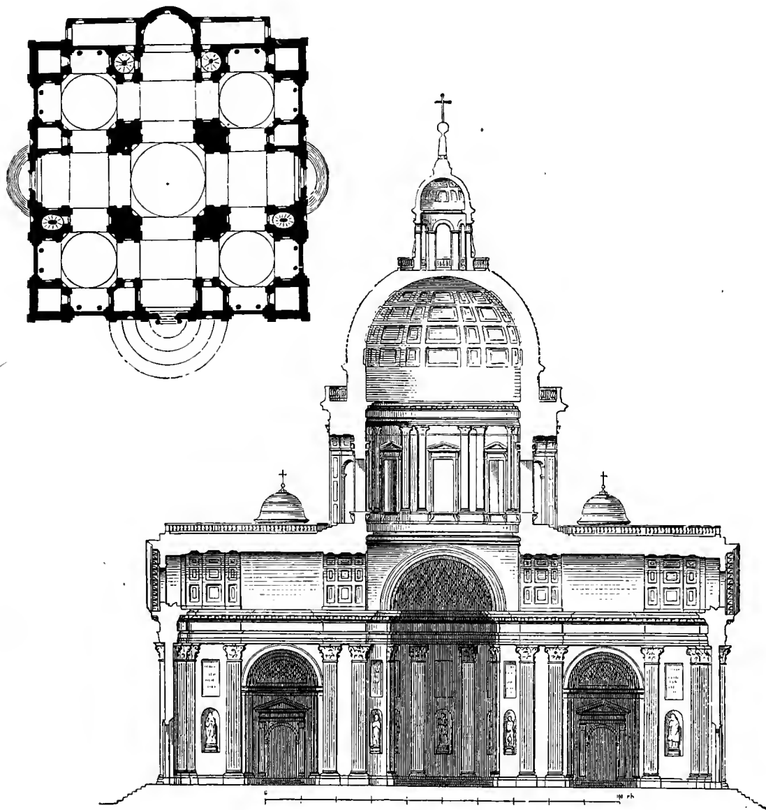
Abb. 119 und 120. Madonna di Carignano zu Genua.
