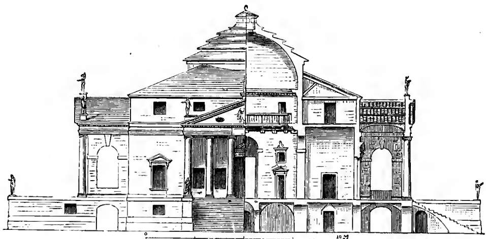
Abb. 262. La Rotonda bei Vicenza.
