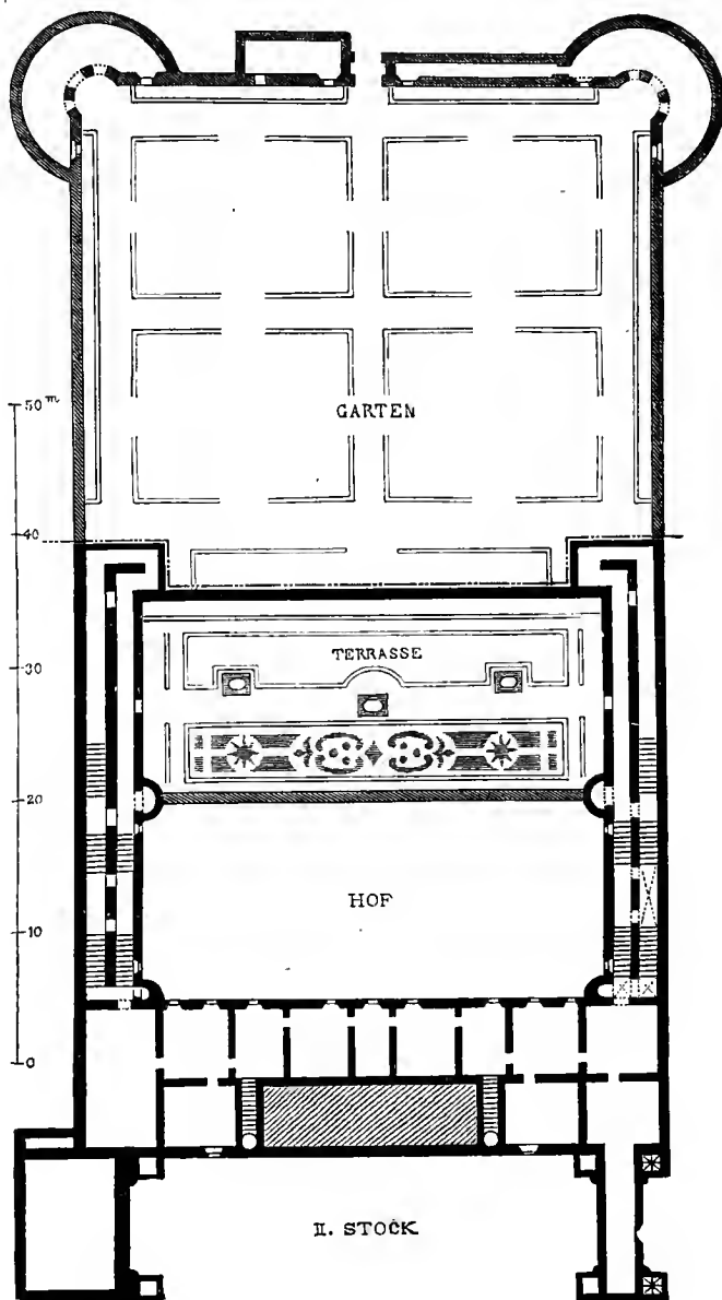
Abb. 255. Monte Imperiale bei Pesaro.
