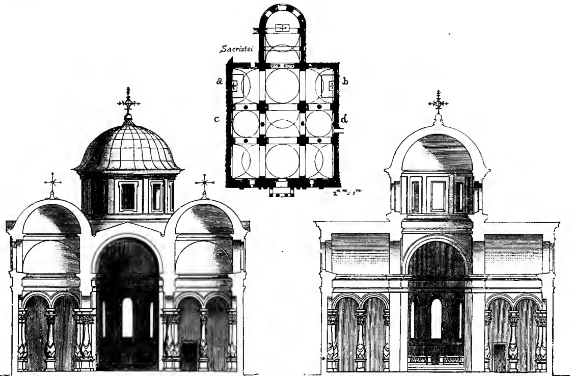
Abb. 98—100. S. Maria de' Miracoli zu Brescia. (Nach Herdtle.)
