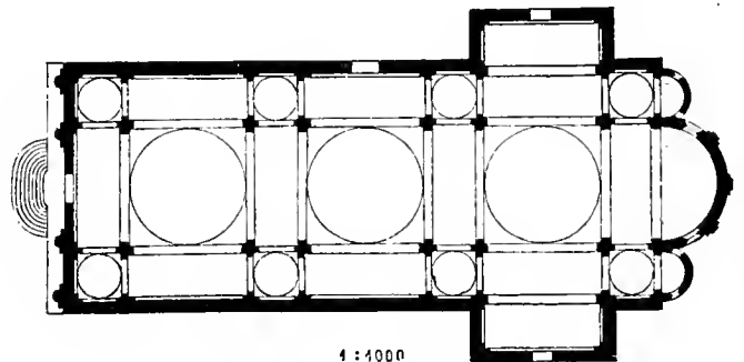
Abb. 167. S. Salvatore zu Venedig. Grundriß.
