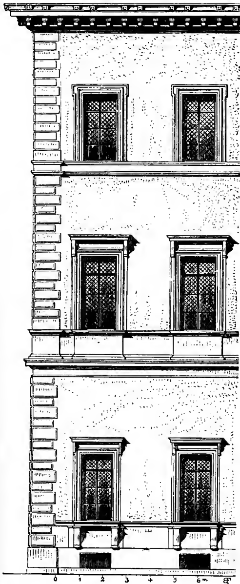
Abb. 206. Pal. Sciarra zu Rom.
