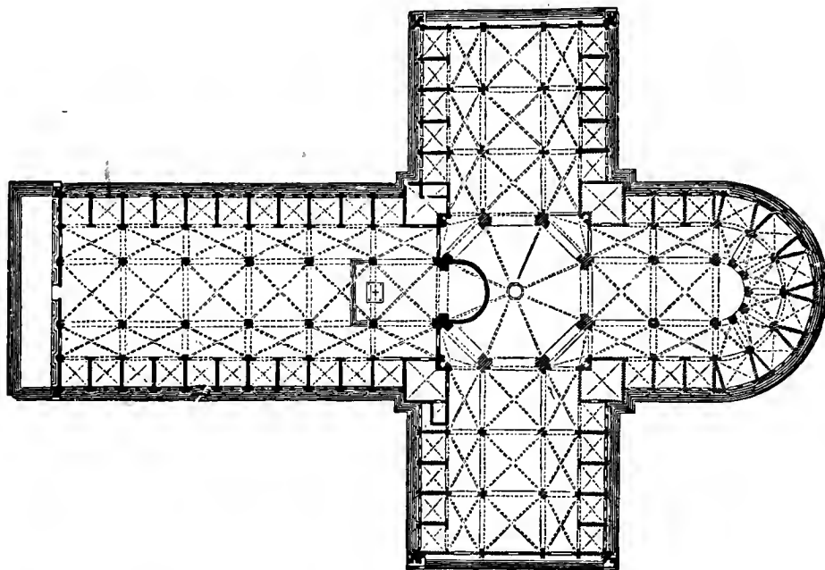
Abb. 9. Grundriß von S. Petronio zu Bologna.
