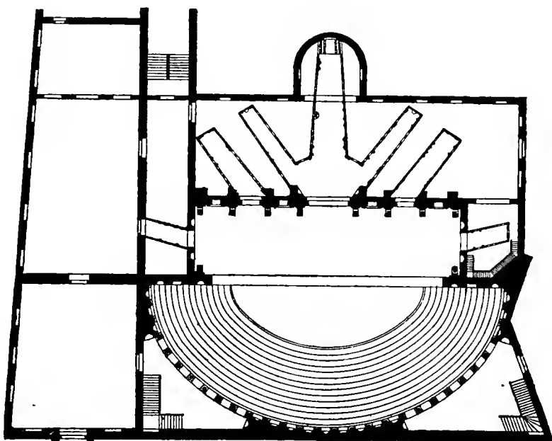
Abb. 334. Palladios Teatro olimpico zu Vicenza. Grundriß. (Nach Gurlitt.)
