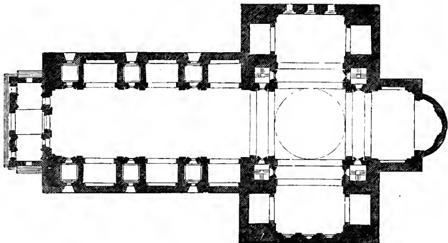
Abb. 146. S. Andrea zu Mantua. Grundriß.
