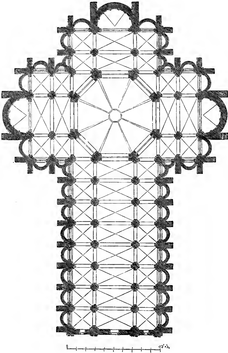
Abb. 156. Dom zu Pavia.
