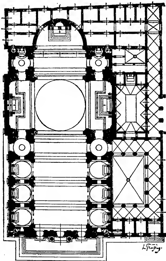
Abb. 153. Il Gesù zu Rom. (Nach Gurlitt.)
