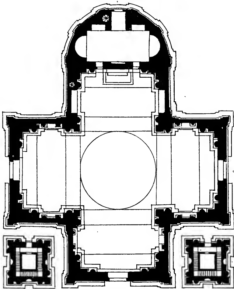
Abb. 92. Madonna di Biagio zu Montepulciano. Grundriß. (Nach Laspeyres.)
