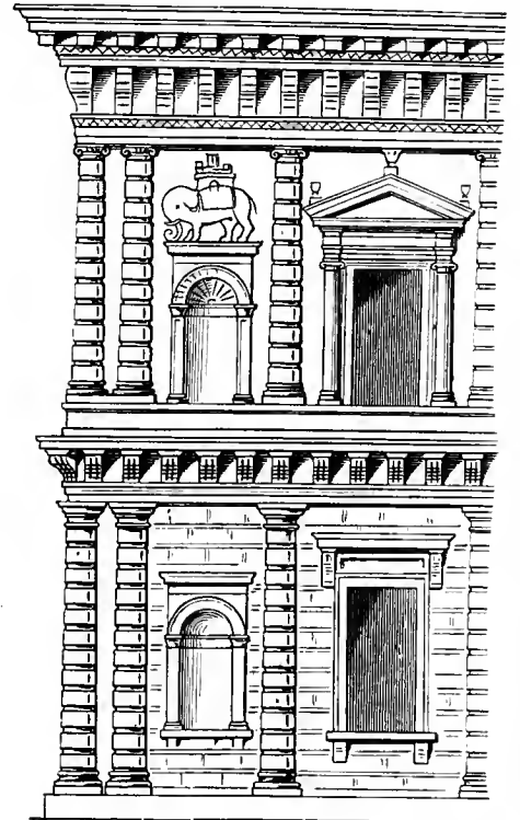
Abb. 235. Pal. Fantuzzi zu Bologna. (Nohl.)
