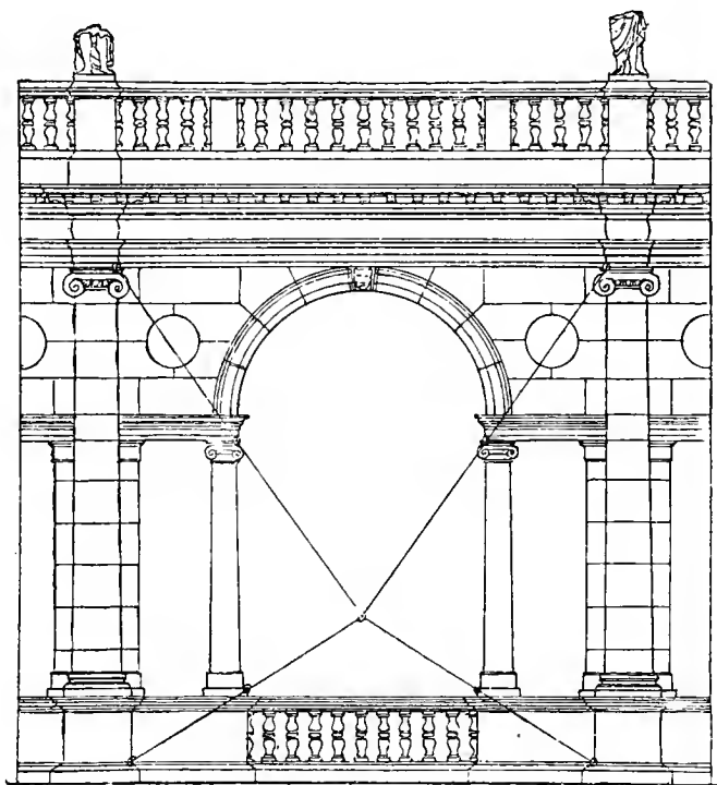
Abb. 81. Von der Basilica zu Vicenza. (Nach A. Thiersch im Handb. d. Archit.)
