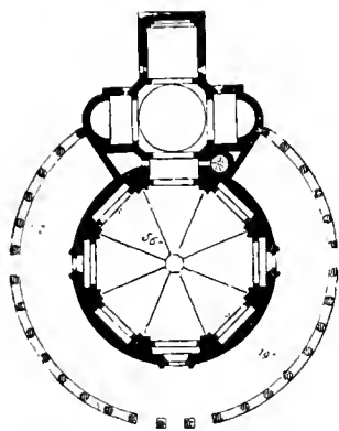
Abb. 114. Madonna di Campagna bei Verona. (L.)
