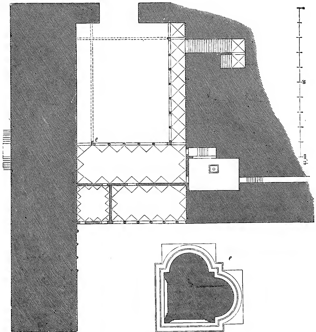
Abb. 201. Pal. Scrofa zu Ferrara. (L.)
