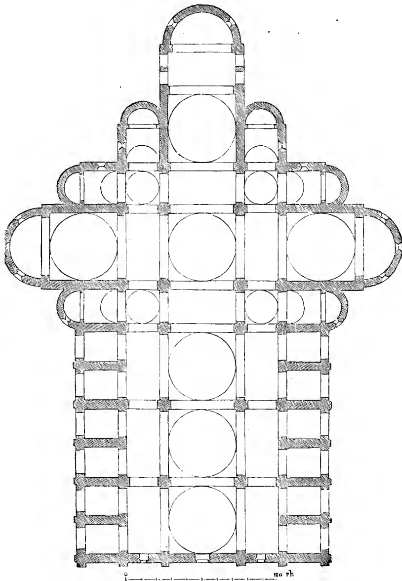
Abb. 165. S. Giustina zu Padua. (L.)
