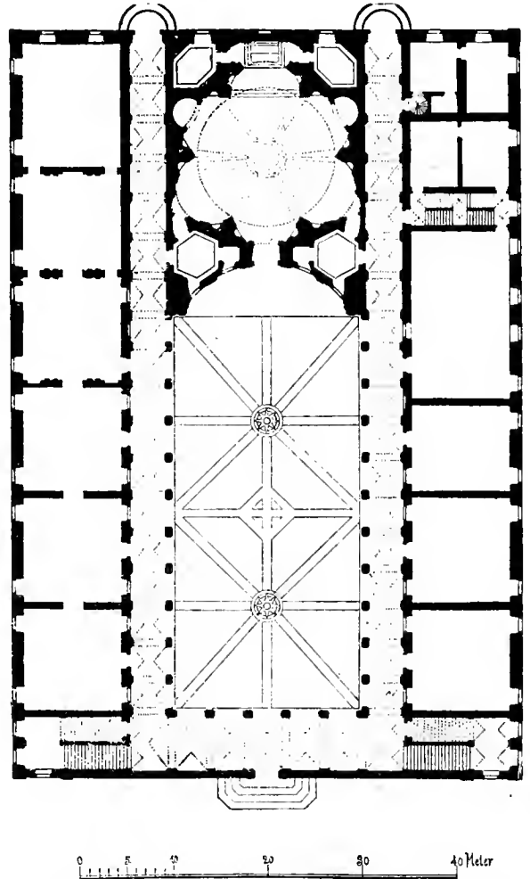
Abb. 186. Sapienza zu Rom. Grundriß. (Nach Gurlitt.)
