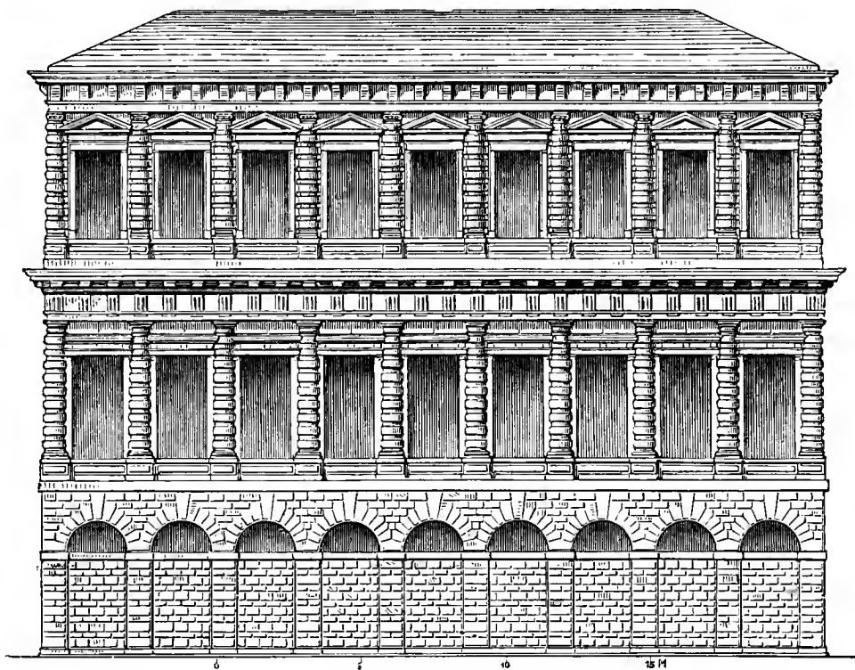
Abb. 59. Zecca zu Venedig.
