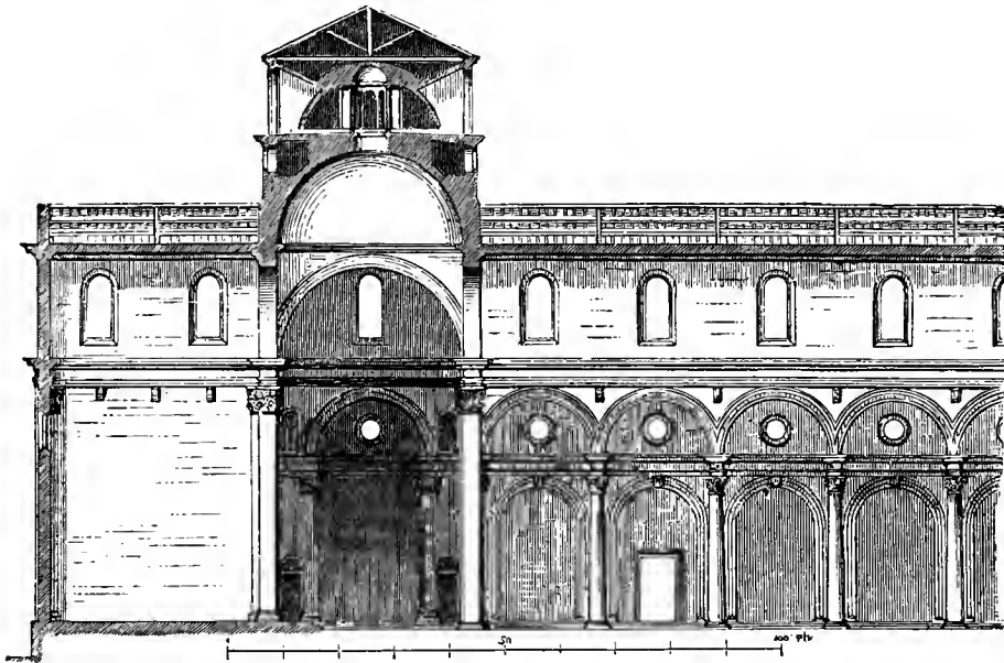
Abb. 137. S. Lorenzo zu Florenz. Längenschnitt.
