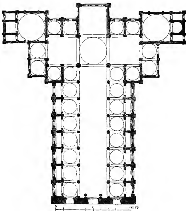
Abb. 138. S. Lorenzo zu Florenz. Grundriß.
