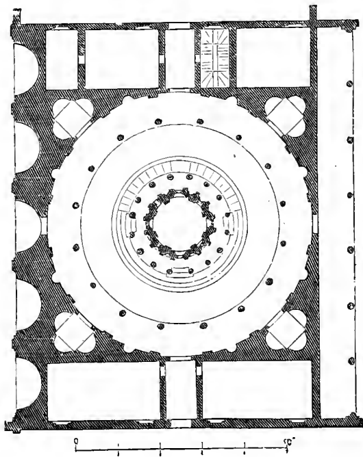
Abb. 103. Tempietto bei S. Pietro in Montorio zu Rom.
