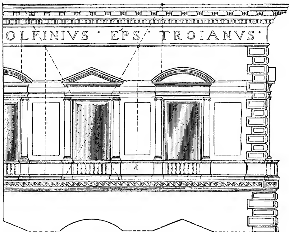
Abb. 72. Vom Pal. Pandolfini zu Florenz. (Nach A. Thiersch im Handb. d. Archit.)
