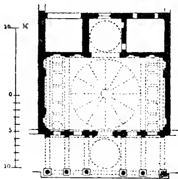
Abb. 87. Capp. Pazzi zu Florenz. Grundriß. (Nach Paulus.)
