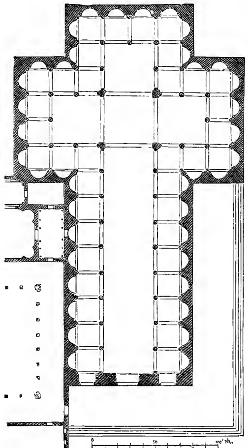
Abb. 140. S. Spirito zu Florenz. Grundriß.
