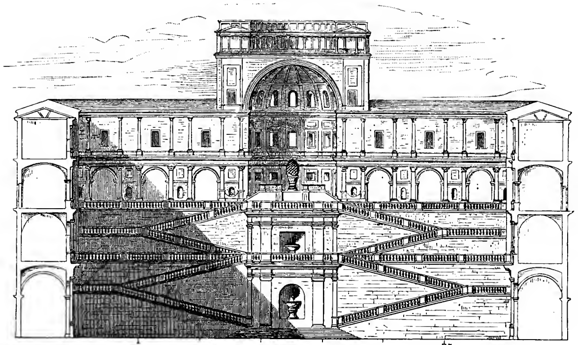
Abb. 215. Querschnitt durch den großen Hof des Vatikans in seinem ursprünglichen Zustande; oben der Giardino della Pigna.
