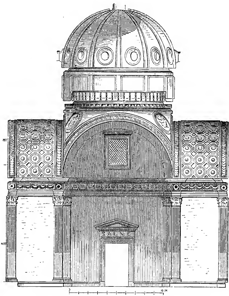
Abb. 91. Madonna delle Carceri zu Prato. (J. Stadler.)
