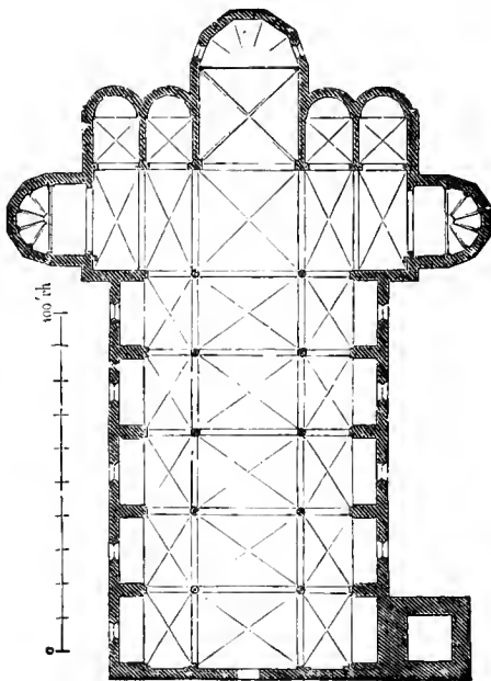
Abb. 142. Servi zu Siena. Grundriß. (L.)
