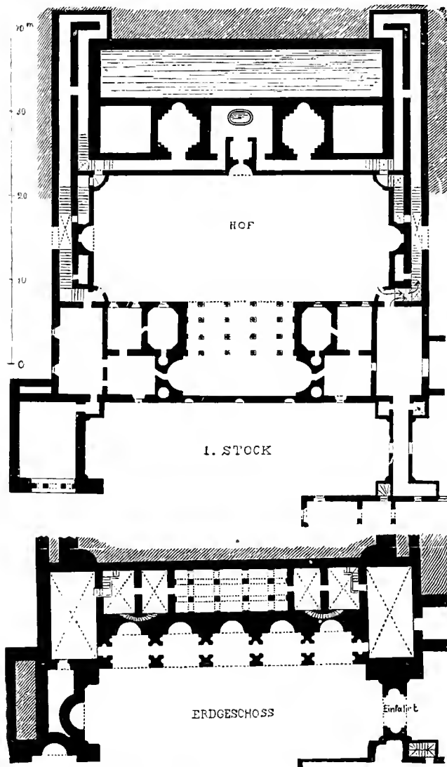
Abb. 256. Monte Imperiale bei Pesaro.
