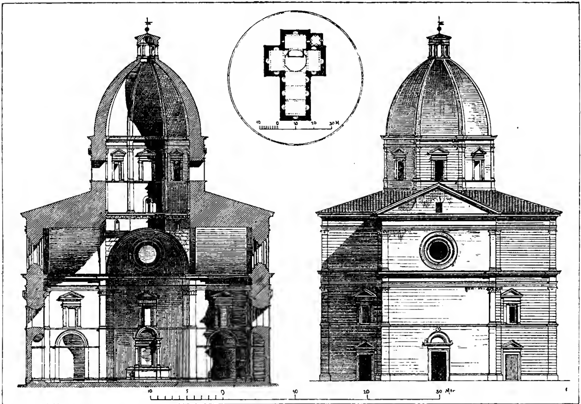
Abb. 147—149. Madonna del Calcinajo bei Cortona. (Nach Gnauth.)
