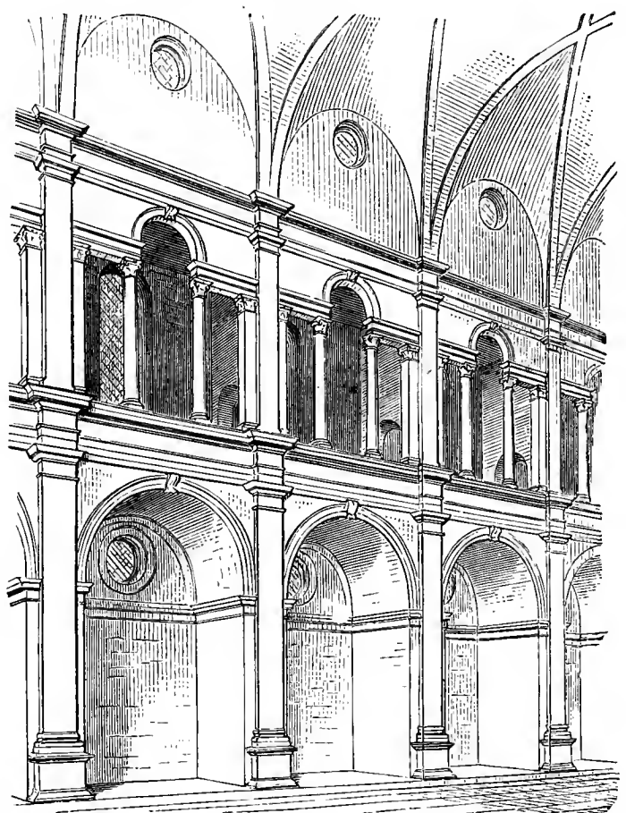
Abb. 150. S. Maurizio (monastero maggiore) zu Mailand. (Lasius.)
