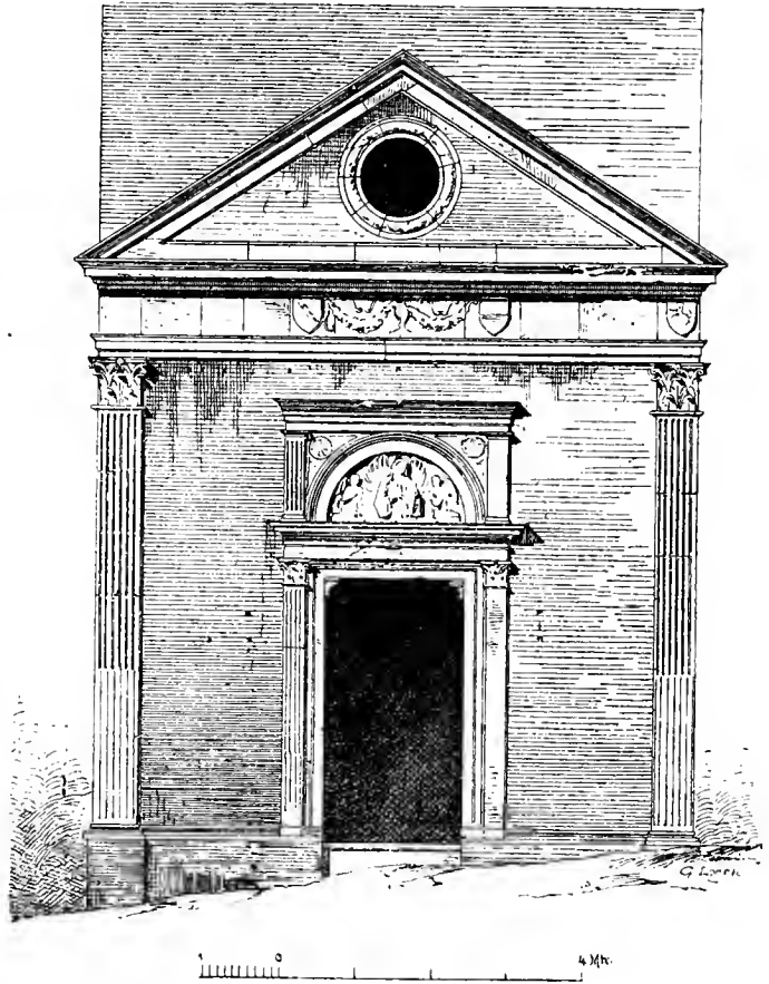
Abb. 127. S. Caterina zu Siena. (Gnauth.)
