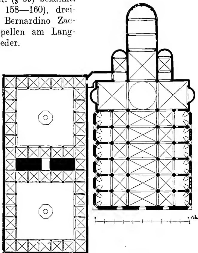
Abb. 158. S. Giovanni zu Parma. (L.)
