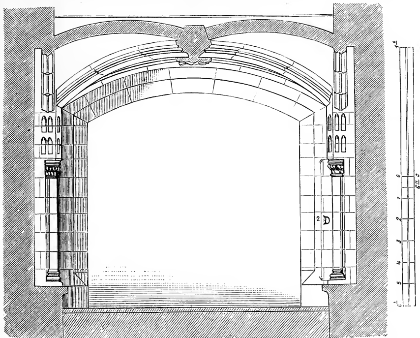
60. Querdurchschnitt der Thorhalle des Presburger Rathhauses.
