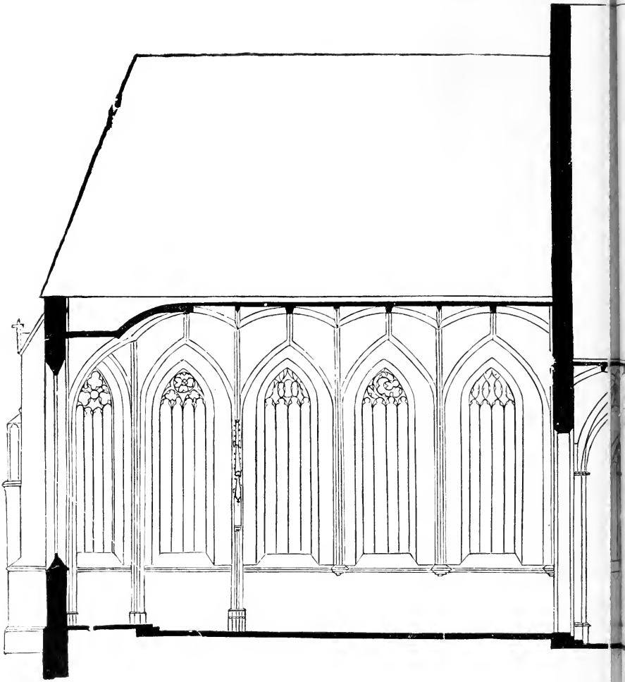
Längenschnitt
