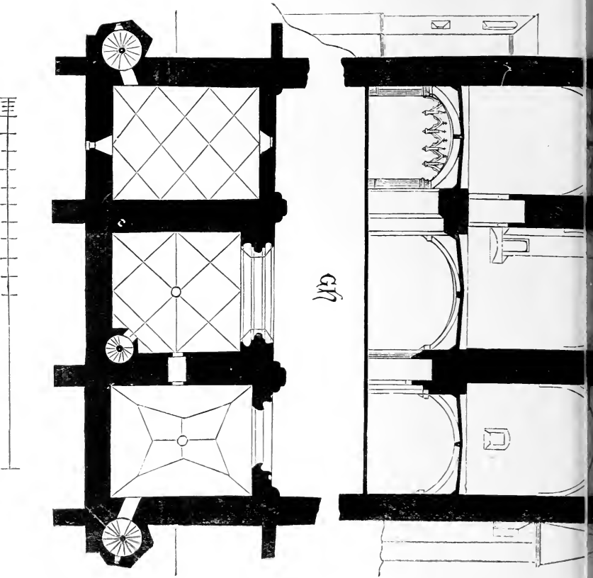
Querschnitt des Pöschinger Domstufwerkes und der Sacrifici.
