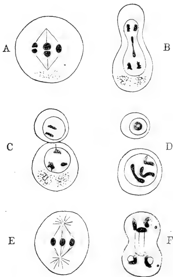
Sl. 3. Spermatogenesisa kod Aphis saliceti . Po v. Baehr-u iz Haeckera.
