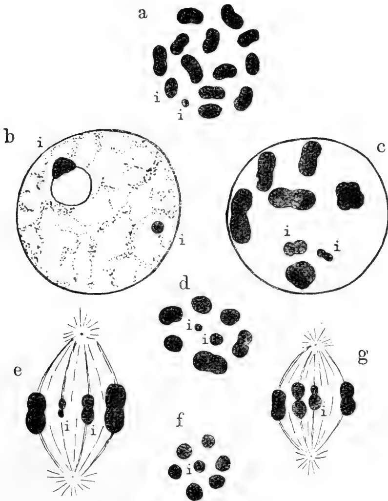
Sl. 2. Spermatogenesisa od Lygaeus turcicus Po Wilsonu iz Haeckera.
