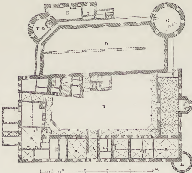
Abb. 227 Grundriß des Alten Schlosses zu Stuttgart
