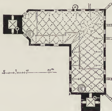
Abb. 223 Oberer Grundriß der Kirche zu Freudenstadt
