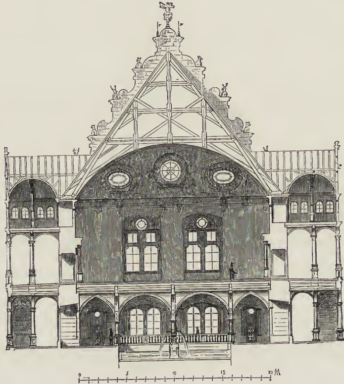
Abb. 231 Querschnitt des ehemaligen Lusthauses zu Stuttgart
