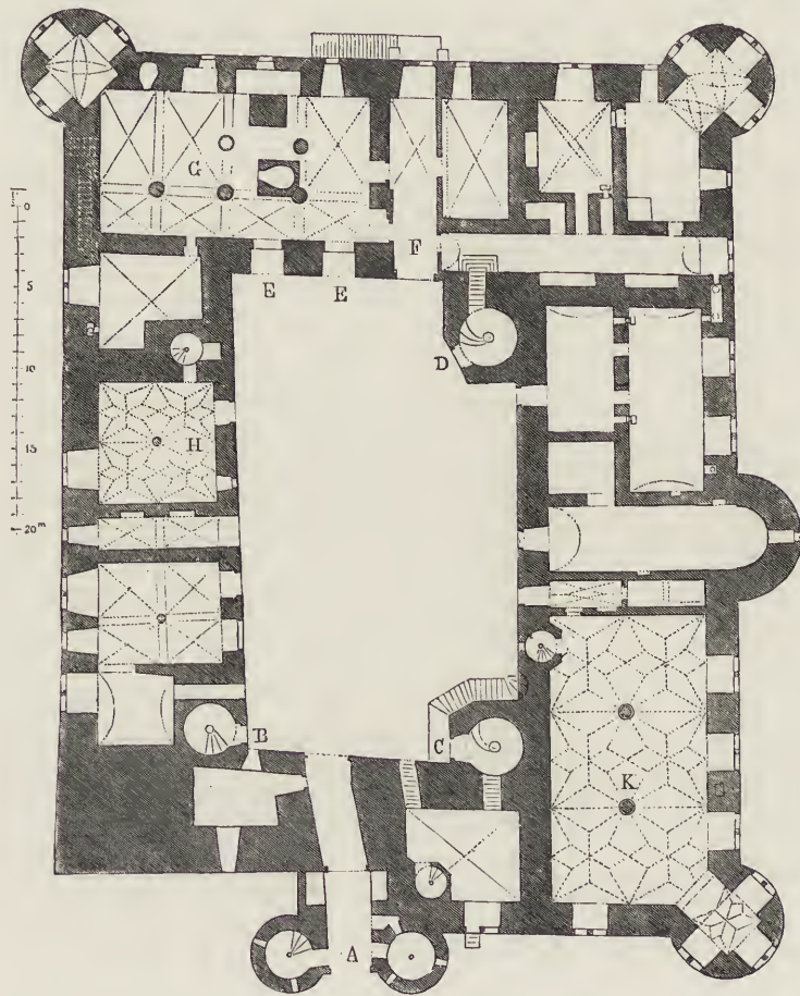
Abb. 295 Grundriß des Schlosses Neuenstein
