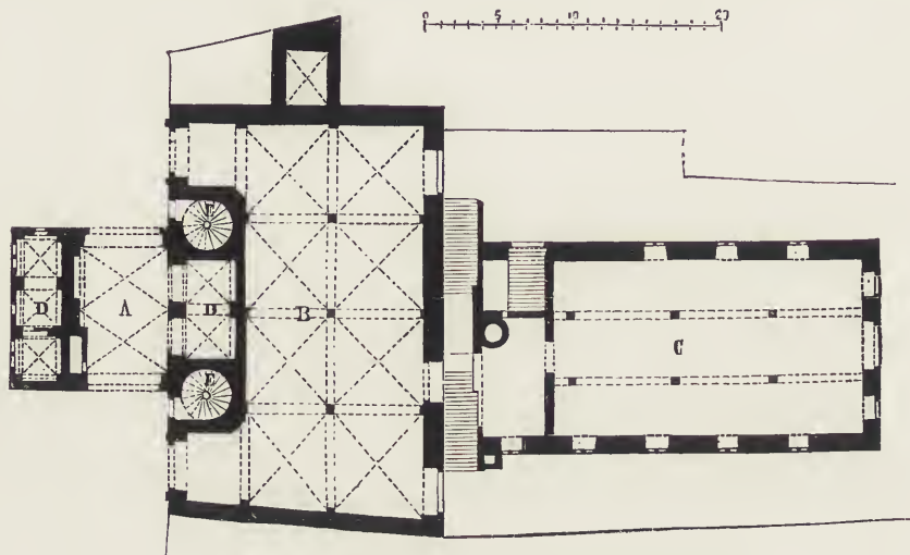
Abb. 292 Erdgeschoßgrundriß des Rathauses zu Schweinfurt
