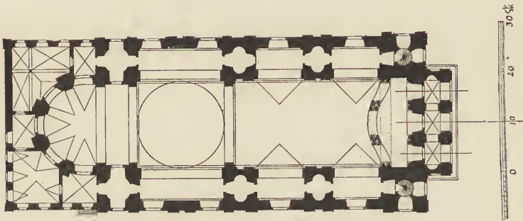
Fig. 52. Jesuitenkirche zu Mannheim. Grundriss.
