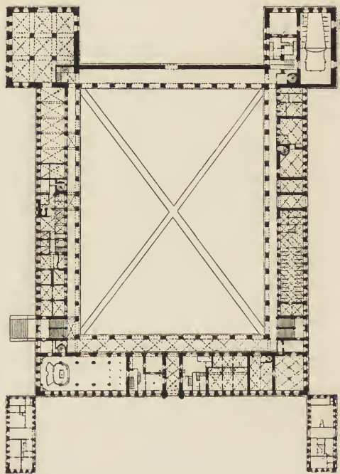
Fig. 14. Schloss Friedenstein zu Gotha. Grundriss.
