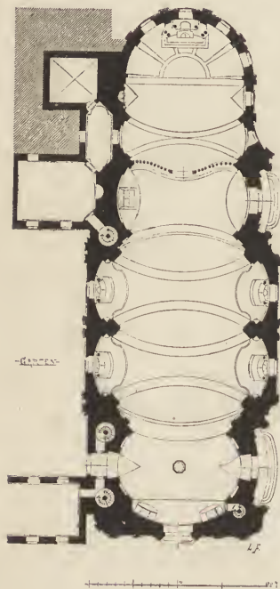
Fig. 57. St. Margareth in Břevnov. Grundriss.
