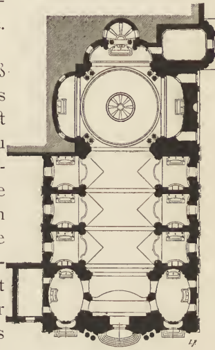
Fig. 59. St. Nikolauskirche zu Prag (Kleinfeite). Grundriß.
