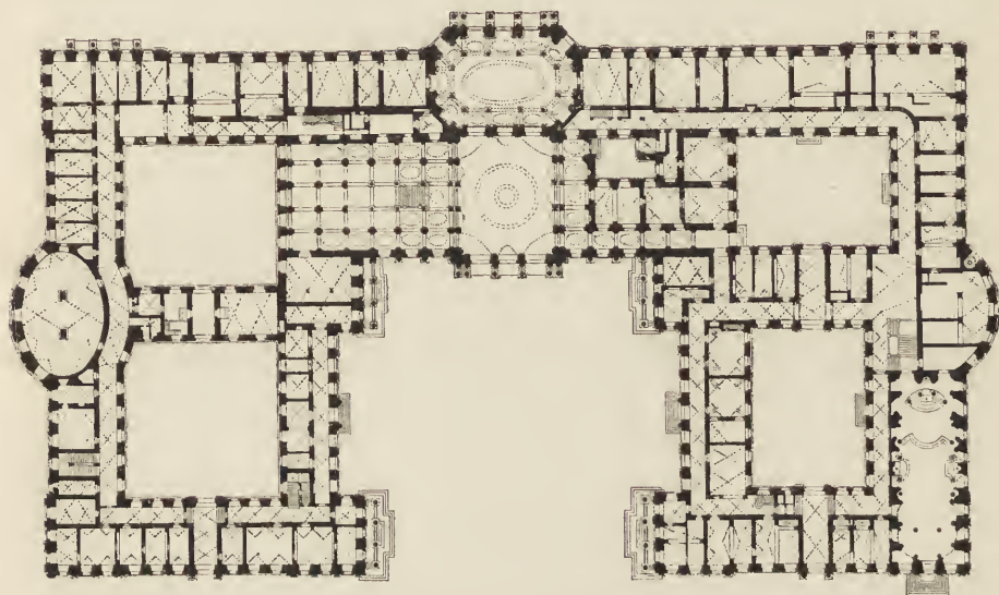
Fig. 107. Residenz zu Würzburg. Grundriß des Erdgeschosses.
