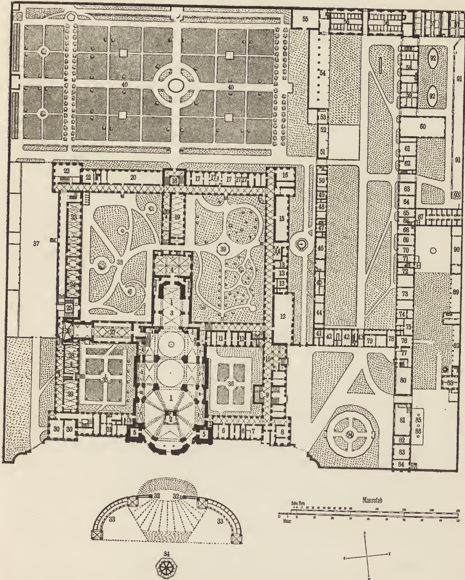
Fig. 90. Kloster Maria-Einfeldeln. Grundriss.
