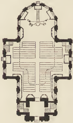
Fig. 146. Dreifaltigkeitskirche zu St. Georg-Hamburg. Grundriss.
