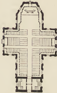
Fig. 147. Hauptkirche zu Altona. Grundriss.
