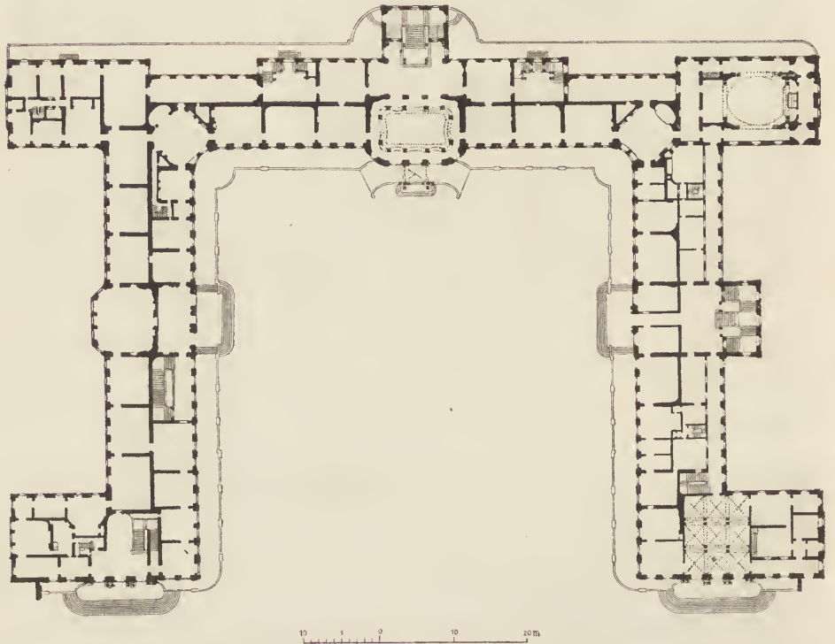
Fig. 156. Residenzschloss zu Stuttgart. Grundriss.
