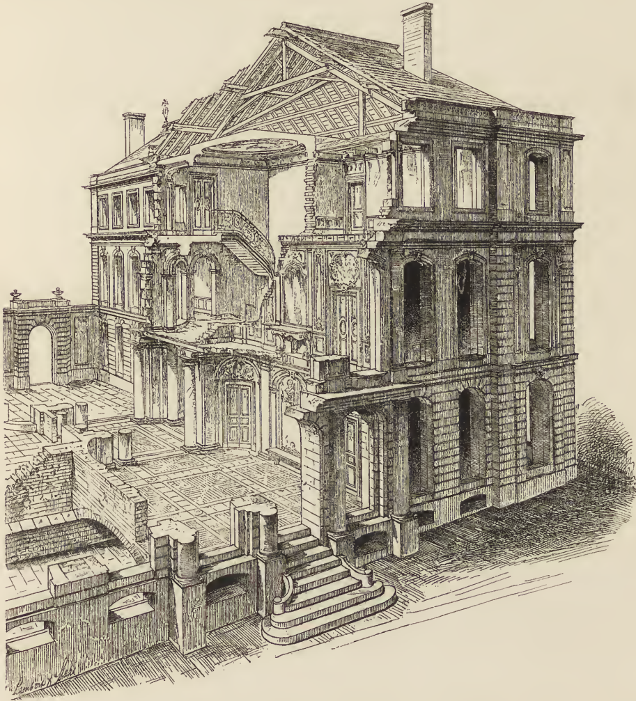
Fig. 167. Hôtel Mallet zu Genf. Perspektivischer Querschnitt.
