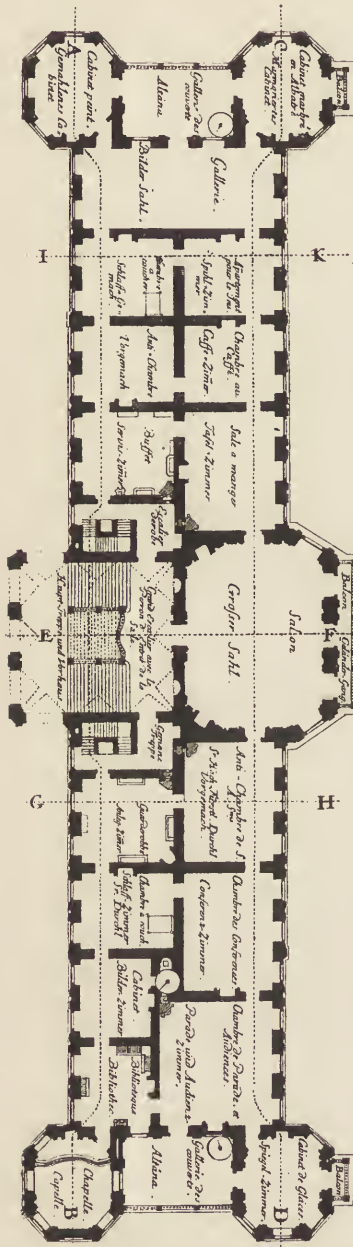
Fig. 67. Schloss Belvedere zu Wien, Hauptgeschoss.
