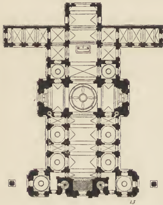
Fig. 105. Dom zu Fulda. Grundriss.
