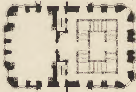
Fig. 163. Schloß Pommersfelden, Grundriß des Mittelbaues.
