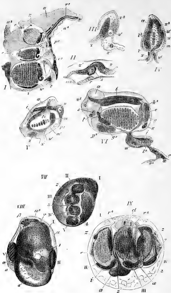
Fig. 170. — Pyrosoma giganteum .
