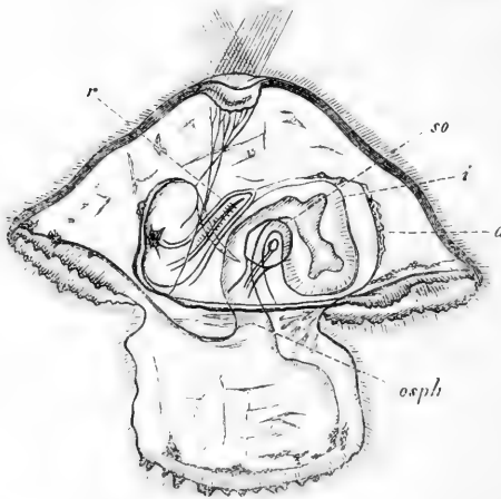
Fig. 35-37. Pilidium gyrans .
