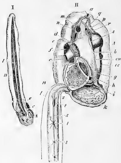
Fig. 167. — Appendicularia flabellum .
