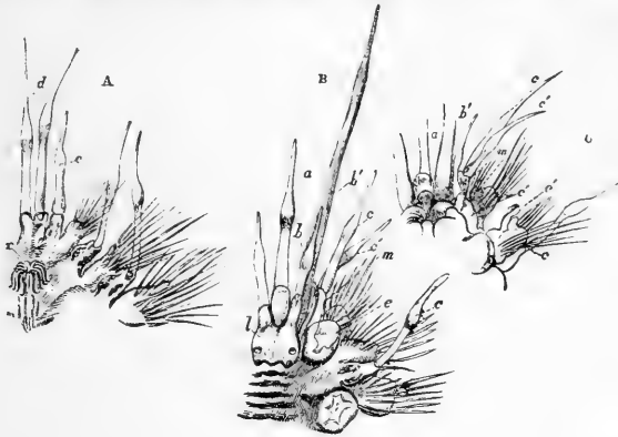
Fig. 56. — Polynoë squamata .
