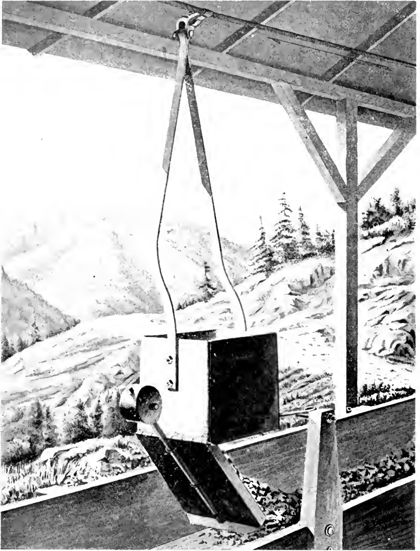
FIG. 29. AUTOMATIC BOTTOM DUMP BUCKET.
