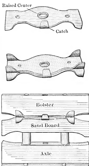
FIG. 144.—Bolster plates.
