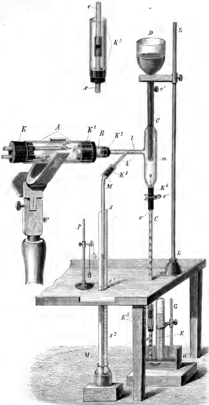
FIG. 205. Apparat für das Studium der Diffusionserscheinungen atmosphärischer Gase von Pflanzenmembranen. D SPRENGEL'SCHE Pumpe mit Quecksilber getrieben. Die Gase, welche auf dem Weg K1 B1 in die Pumpe gelangen, werden in dem Abförpionsrohr E aufgefangen. s1 s2 Manometer, welcher den Druck in der Pumpe anzeigt. In der Erweiterung von B ist ein Gypsstopf, auf welchem die Membran liegt. In A werden die Gase durch a'' ein, durch b'' ausgelaufen. In P eine Sekundenuhr, welche gleichzeitig mit dem Spiegel des Manometers s abgelesen werden kann.
