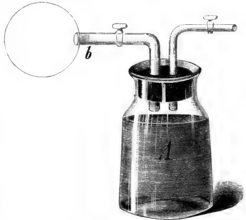
FIG. 2. Wenn man den Behälter A, Fig. 2, mit \text{CO}_2 füllt und in b eine Seifenblase mit diesem Gas füllt, dann den Hahn schließt, so kann man beobachten, wie die Gasblase allmählich zusammen sinkt, bis sie verschwindet. Stellt man aber eine Wasserstoffblase her, so wächst diese, bis sie platzt.
