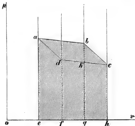
FIG. 429. Schema des umkehrbaren Kreisprozesses. Die Ordinate o nach p stellt den Druck, die Abscisse o nach v das Volum dar.
