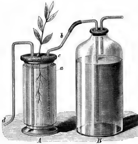
FIG. 394. Apparat für Wasserculturen. A der Behälter, in welchem die Pflanze wächst, c eine durchlöchernte Korkplatte, b das Zuleitungs-, d das Ableitungsrohr für die Nährstofflösung aus dem Reservoir B, a eine undurchsichtige Hülle von Pappe.
