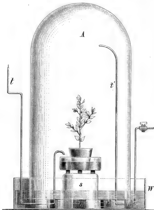
FIG. 395. Die Glasglocke A ruht auf drei Porzellan- oder Glasfüßen in der Wanne W , auf dem umgestülpten Glas s steht eine zweite Schale, in welcher der Blumentopf steht. Dieselbe wird durch die Röhre t mit Wasser gefüllt, so daß der Blumentopf dieses imbibiren kann. Die Wanne W wird bis zur Sperrung der Glocke A mit verdünnter Schwefelsäure gefüllt. Das zweite Rohr führt Kohlenstoffdioxid, welche auf das sorgfältigste gereinigt ist, in die Glocke A . BOUSSINGAULT'S Nachweis, daß das N der Atmosphäre nicht assimiliert wird. Ann. d. sc. nat. Bot. IV. Sér., I. Bd. 1854. Recherches sur la végétation etc.
