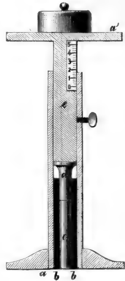
FIG. 402. Das Tischchen, welches zum Auspressen des Wassers aus dem Holze benutzt wurde. Die Metallhülfe b , welche den Bohrschnitt c aufnimmt, kann von dem Fuß aus in das Tischchen eingefchoben werden.
