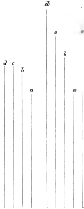
FIG. 191. Aus zwei gleich langen Cylinderabschnitten wachsender Sonnenrosenfähne wurde das Mark herausgeschnitten, in Wasser gelegt und nach 3 Stunden b , nach 14 Stunden c , nach 21 Stunden d gemessen.
