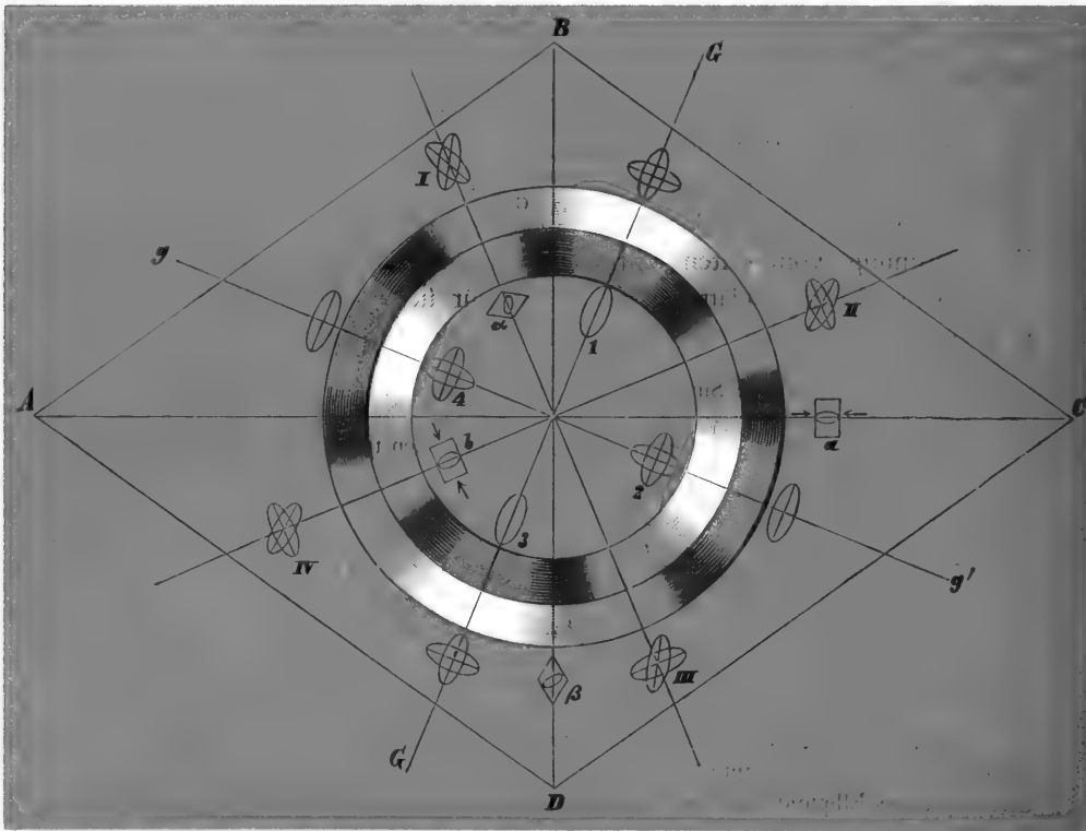
FIG. 140. ABCD ist ein Gypsplättchen von Roth I. G ist die Richtung der größten, g die Richtung der kleinsten Elastizität. Im inneren Farbenring rotirt ein Gypsplättchen Bläulichweiß erster Ordnung \alpha oder ein in Richtung der Pfeile comprimirtes Glaswürfelchen b . Im äußeren Farbenring rotirt ein gleiches Gypsplättchen \beta oder ein Glaswürfelchen, welches in Richtung der Pfeile a comprimirt ist. 1, 2, 3, 4 die Lage der Elastizitätsellipsen im festliegenden Gypsplättchen zu denjenigen des rotirenden. Im äußeren Ring haben diese die umgekehrte Lage, in allen diesen Quadranten aber schneiden sich die ungleichnamigen Elastizitätsachsen unter rechtem Winkel oder sie fallen zusammen, 1, 3 innen, 2, 4 außen. In den mit I, II, III, IV bezeichneten Stellen schneiden sich die Elastizitätsellipsen unter Winkeln von 45^\circ .
