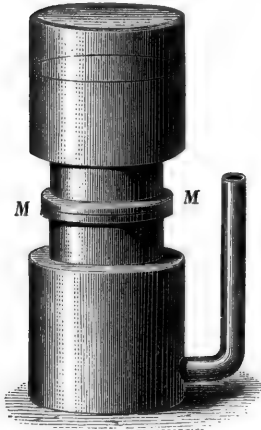
FIG. 397. Recipient für osmotische Versuche. In der Berührungsfäche M M der beiden Gasgefäße wird die Membran befestigt. Die Ränder der Gläser können durch Klammern aneinandergepreßt werden.
