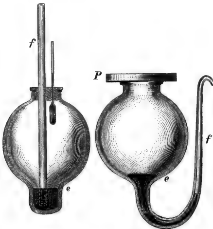
FIG. 116. Quellungsmeßer.
