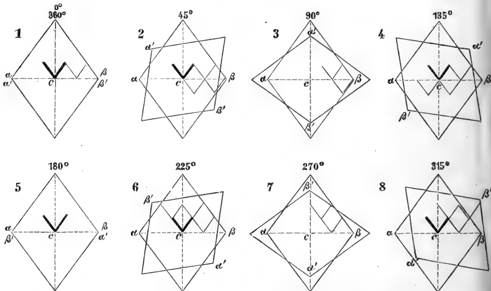
FIG. 129 A. Zur Analyse der hier einschlägigen Phänomene kann man zunächst die Rotation eines Kalkspates um einen Strahl als Axe, sodann aber auch die Rotation eines solchen Kryftalles \alpha' \beta' um einen gleich dicken \alpha \beta , welcher bezogen auf den Strahl \sphericalangle festliegt, anwenden. Bei dieser Drehung nach \overline{12} ( 45^\circ ) findet eine Uebertragung beider in dem festliegenden gebrochenen Strahle in den zweiten Kryftall statt. Bei einer Drehung um \overline{13} ( 90^\circ ) wird nur der extraordinäre in \alpha' \beta' durchgelassen. Bei einer Drehung um 180^\circ (1 nach 5) wird hingegen nur der ordinäre Strahl durchgelassen. Man nennt den gewöhnlichen Strahl im Hauptschnitt \alpha \beta , den außergewöhnlichen senkrecht zum Hauptschnitt polarisiert. Das Schema zeigt dann die Brechung und den Durchgang von \sphericalangle und \sphericalangle' , und da sich \sphericalangle und \sphericalangle' leicht, bezogen auf den Ort c , orientiren lassen, die Lage der Brechungsebenen für \sphericalangle und \sphericalangle' .
