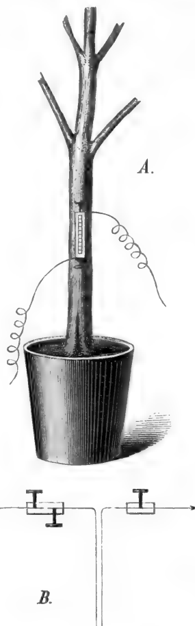
FIG. 474. A. Eine Thermofaule, am Stamm einer Daturapflanze eingelassen. B. Eine Nadel, welche aus einem Antimon- und Wismuthstreifen zusammengelöthet ist, in Richtung der Pfeile mit dem Multiplikator verbunden.
