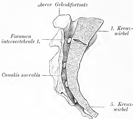
Fig. 41. Kreuzbein, Medianschnitt.
