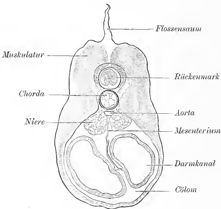
Fig. 1. Tritonlarve, Querschnitt.
