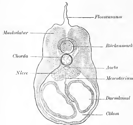
Fig. 7. Tritonlarve, Querschnitt.
