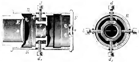
Fig. 409 V. s. Hünig: Geometr. Instrumente
