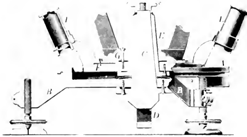
Fig. 323. Aus Hünac's, Geometr. Instrumente
