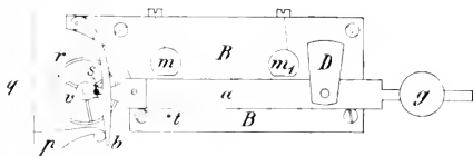
Fig. 196a. (Nach Tobler, Elektr. Uhren.)
