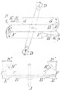
Fig. 285 (Nach Caspari, Nautische Instr.)
