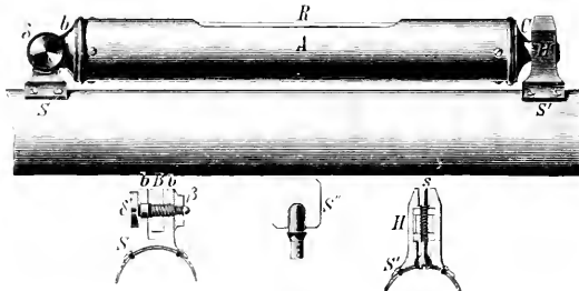
Fig. 74. Nach Hünneke, Geometr. Instrumente)
