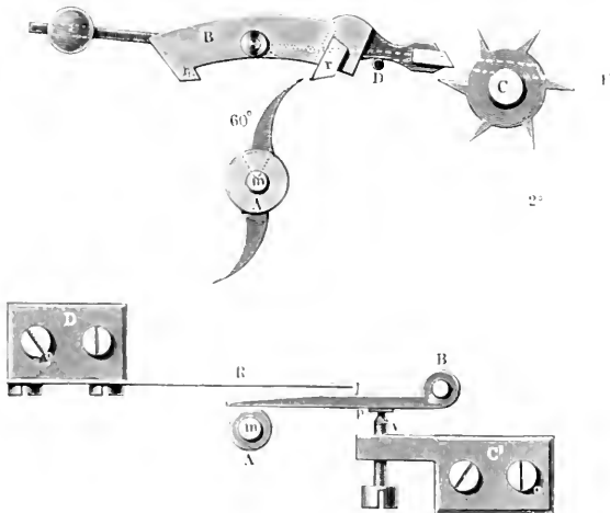
Fig. 297 Ank. kontak' v. Anordnung
