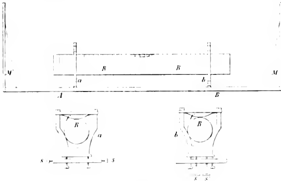
Fig. 83. Nach Carl Preussner's Konstruktion.
