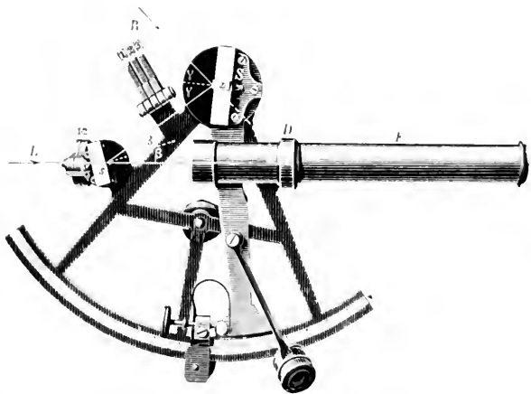
Fig. 136 Aus Jordan, Zeit- u. Ortbestimmungen
