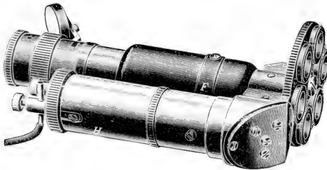
Fig. 564. Taschenspektroskop mit Skala.
