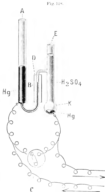
Kapillarelektrometer (ohne Stativ).
