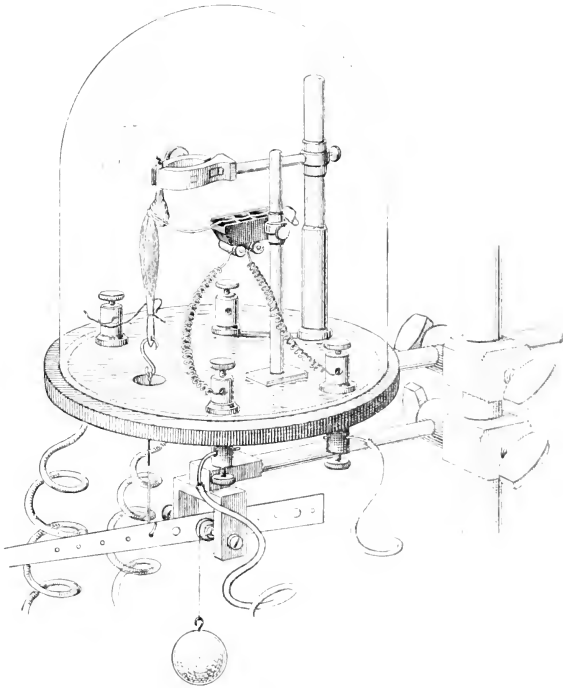
Feuchte-Kammer mit Nervemuskelpräparat
