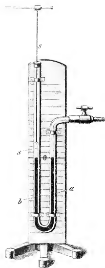
Registrierende Quecksilbermanometer. 15.
