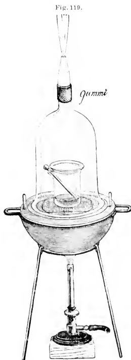
Dampfbad. \frac{1}{2} nat. Gr.
