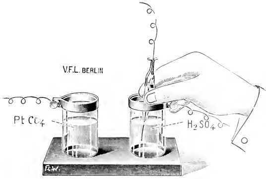
Platinierungs- und Reduktionsgefäß.
