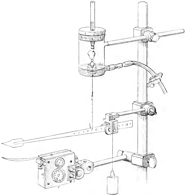
Isoliertes Frosterz in Herzkammer über Ringerlösung Sauerstoffdurchleitung. Jaquet'sche Zeitmarkenrühr.
