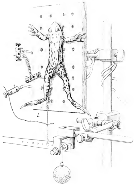
Rana esculenta . Versuchsordnung zur elektrischen Reizung des Musculus gastrocnemius .
