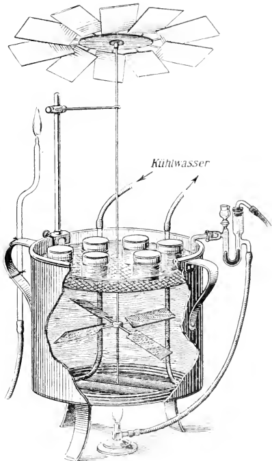
Thermostat nach Wilh. Ostwald , (Nach Peck .)
