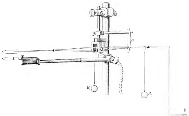
Schreibhebel zur Tropfenregistrierung nach Steud.
