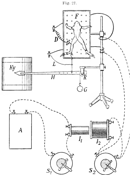
Versuchsanordnung zur Abbildung der Öffnungs- oder Schließungsinduktionsschläge.
