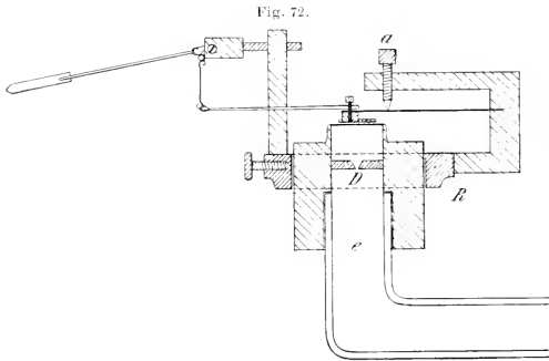
Kopf des Federmanometers (nach Fronk und Petter ).
