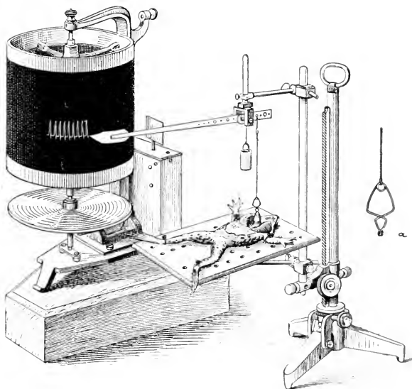
Graphische Registrierung der Herzstätigkeit. a Herzklammer.
