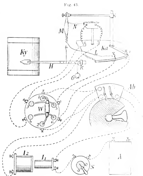
Versuchsordnung zur rhythmischen elektrischen Reizung des Nervenmuskelpräparates mit Öffnungs- oder Schließungsinduktionsschlägen
