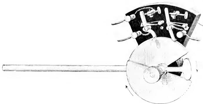
Rotierender Abblender nach O. Froel.
