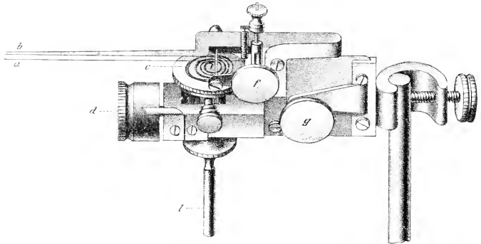
Elastisches Manometer, nach Härthle-God.
