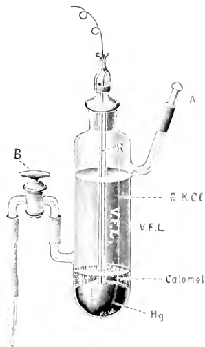
Kalomelektrode.
