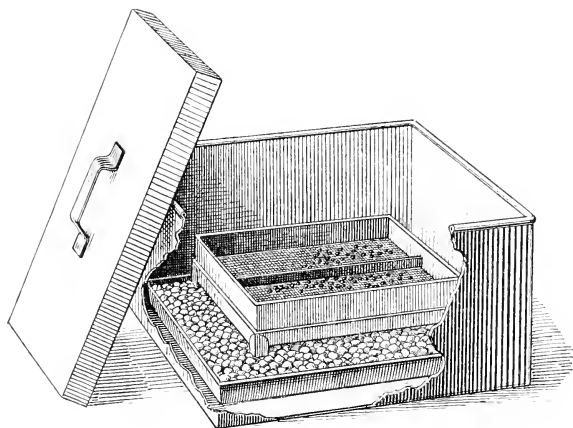
Trockenkasten von Krönig und Paul . (Nach Paul .)
