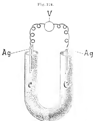
Schema einer Silber Konzentrationskette
