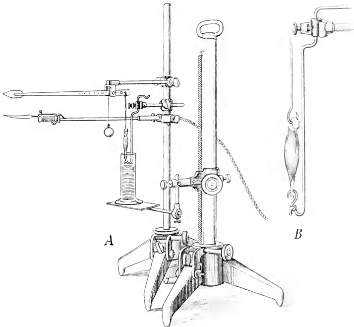
Versuchsordnung zum Einhängen des Muskels in Lösungen
