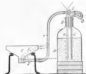
Wasserbad mit konstantem Niveau nach Schirm.
