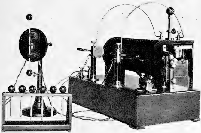
Induktor mit Ölkondensator und Funkenständer nach W. Gummelt .
