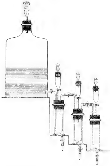
Apparat zum Sterilisieren lebender Wasserpflanzen. Nach Pollacci.
