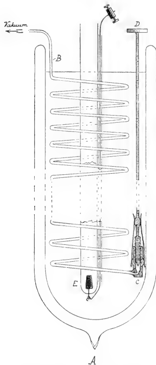
Apparat zum Kühlhalten flüssiger Luft nach Franz Fischer und Schröter.
