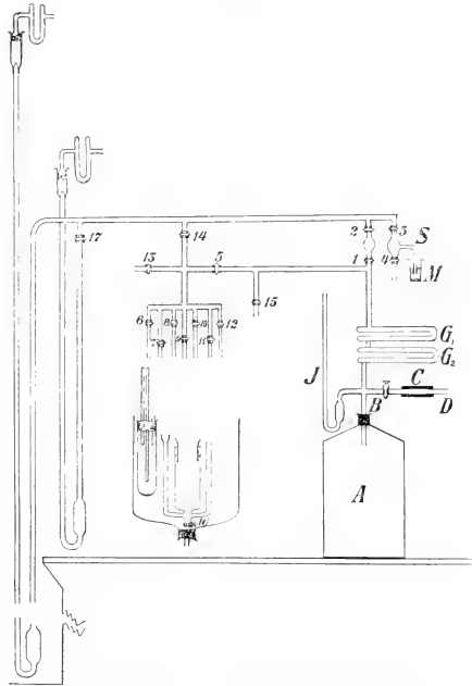
Whatmoughscher Apparat zur Bestimmung der Oberflächenspannung.
