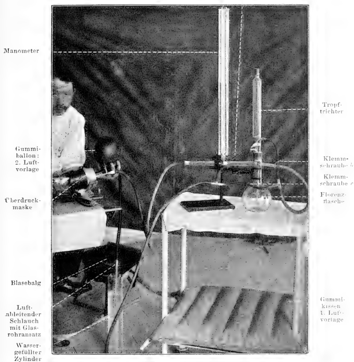
Modifizierter Volhard'scher Überdruck-Apparat mit einfacher Überdruckmaske im Gebrauch.
