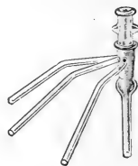
Fraktioniervorrichtung nach Hahn .
