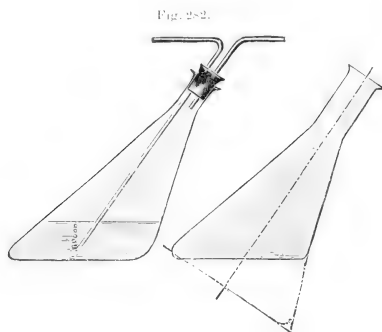
Fig. 282. Analysekolben nach Herzka .
