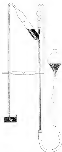
Töpler-Quecksilberluftpumpe nach Antropoff.
