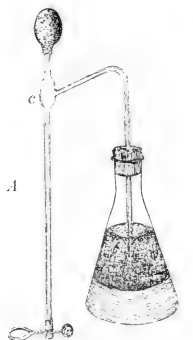
Heber nach Jacobson und Dinsmore .
