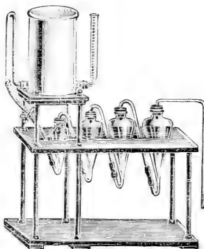
Schlammapparat nach Nöbel.
