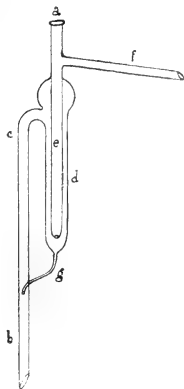
Fraktionieraufsatz nach Comanducci.
