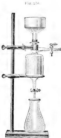
Saugapparat mit Ablasshahn nach Barthel.
