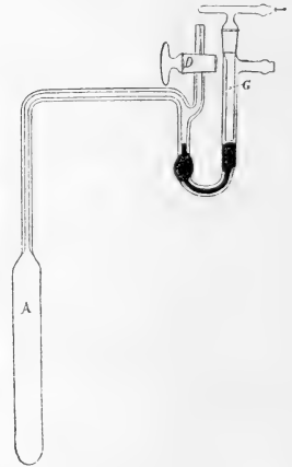
Thermoregulator für Gasheizung nach Poetschke.
