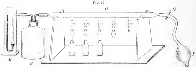
Absorbometer zur Entwicklung des Chromatogramms bei kleinen Flüssigkeitsmengen nach M. Tsvett.
