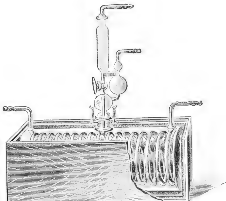
Schüttelgefäß mit Innentemperaturung und Gasableitung nach Kempf. (Neue Form.)
