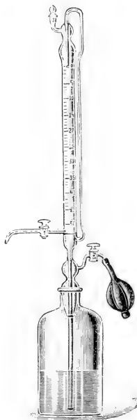
Titrierapparat mit automa- tischer Nullpunkteinstellung nach dem Heberprinzip.
