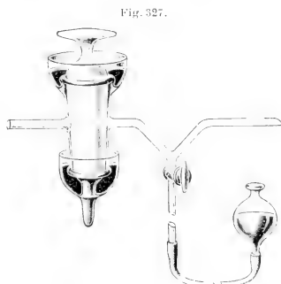
(Quecksilberdichtung eines senkrecht stehenden Hahnes.
