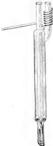
Fraktionieraufsatz für Glasperlenfüllung nach Golodetz.
