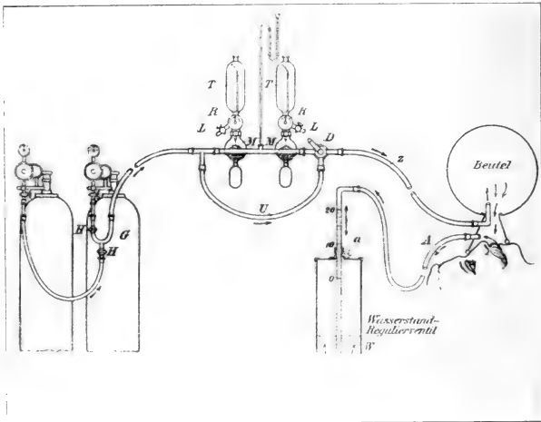
Tiegelsche Apparatur.
