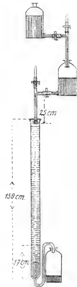
Reinigung von Quecksilber nach Moore.
