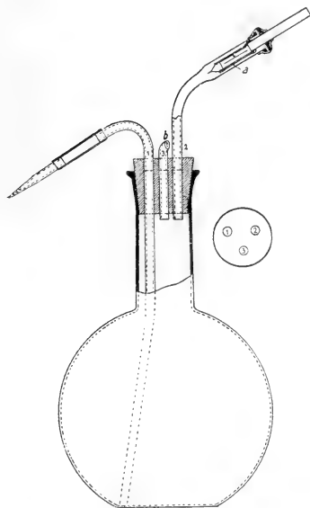
Spritzflasche mit Ventilen nach Schaaare .
