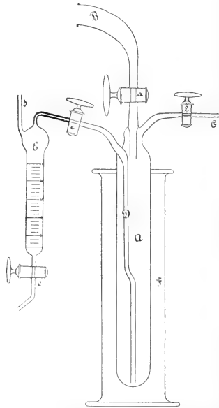
Apparate zum Aufbewahren und Abmessen giftiger, hygroskopischer oder tiefsiedender Flüssigkeiten nach Steinkopf.
