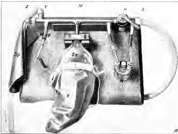
Überdruckapparat für Tieroperationen nach von den Velden.
