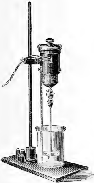
Rührer mit direktem elektrischen Antrieb nach Stähler.
