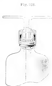
Quecksilberdichtung eines Flaschenstopfens.
