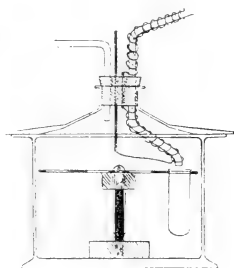
Apparat zur fraktionierten Vakuumdestillation leicht erstarrender Substanzen nach Brown.
