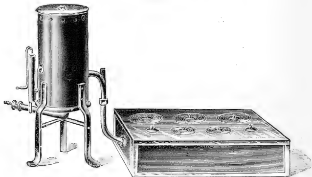
Wasserdampfbad nach Carliczek.
