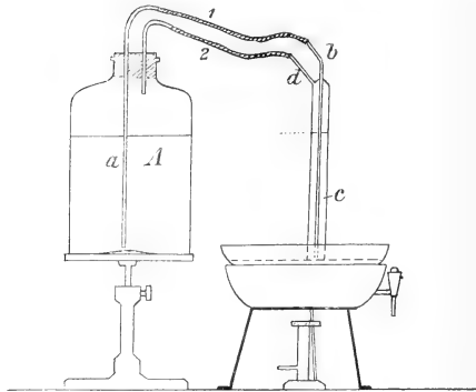
Niveaualter nach Noga.
