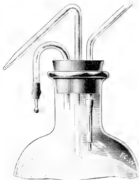
Spritzflasche mit Ventilen nach Gamber .
