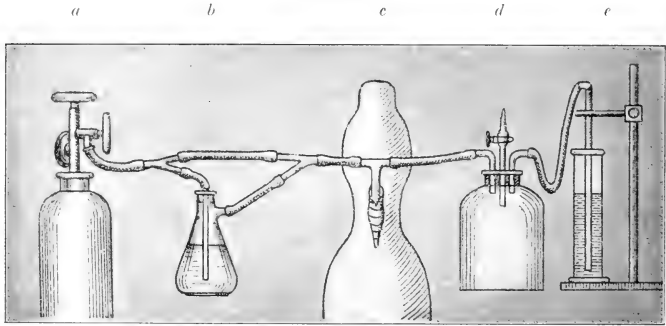
Versuchsanordnung nach Broder.
