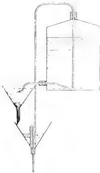
Selbsttätig arbeitende Waschvor- richtung nach Grégoire.
