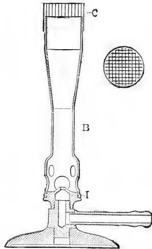
Meker-Brenner.
