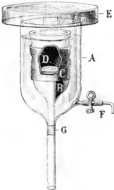
Eistrichter nach Serger.
