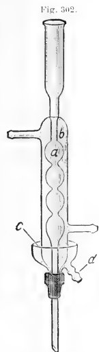
Vorrichtung zum Auffangen des Kondenswassers an Rückflüßkühlern nach Dede .
