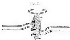
Schräg gebohrter Glashahn mit Quecksilberdichtung nach Göckel.
