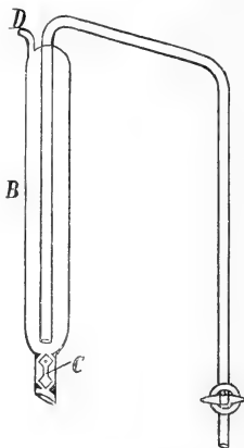
Fig. 283. Sichertheitsheber nach Niemann .
