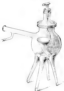
Fraktioniervorstoß nach Glaser .
