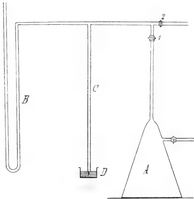
Schematisches Übersichtsbild des Whatmoughschen Apparates.
