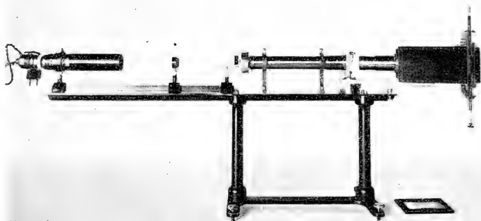
Gitterspektrograph mit vertikalem Spalt nach O. Schumm .
