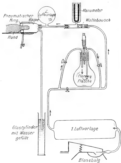
Überdruckapparat in schematischer Darstellung.
