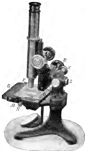
Meßmikroskop nach F. Löwe von Carl Zeiß.
