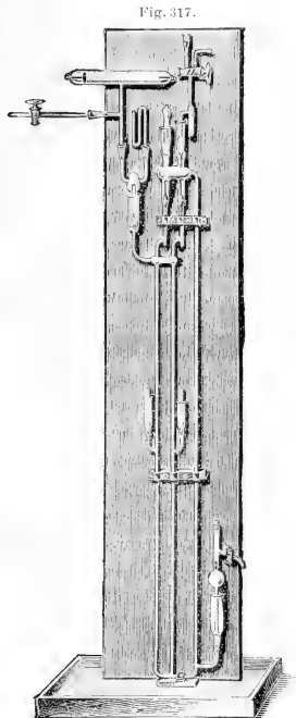
Sprengel-Quecksilberluftpumpe nach Beutell.
