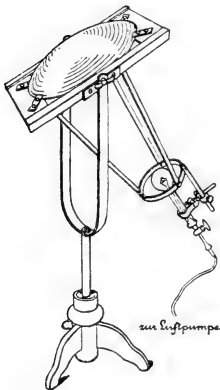
Sonnenvakuumofen nach Stock.
