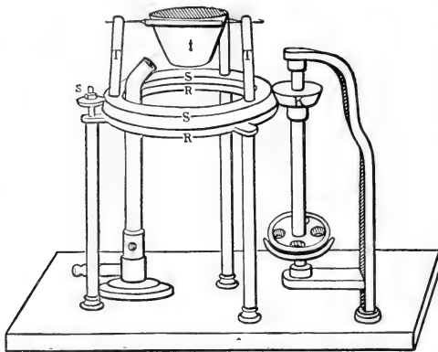
Apparat zur sicheren und gleichmäßigen Veraschung nach Hodes und Göbel.
