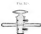
Hahn mit Quecksilberdichtung nach Göckel.
