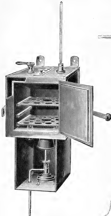
Intensiv-Trockenschrank nach Stähler.
