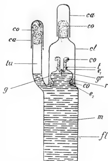
Apparat zur sterilen Pflanzenkultur. (Nach H. Combes.)
