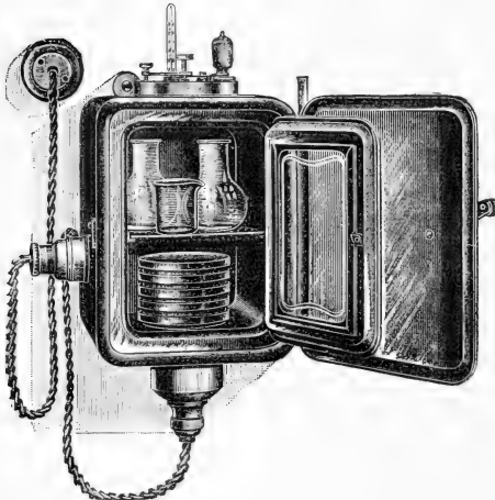
Thermostaten-Luftbad mit Glühlampenheizung nach Hanfland.
