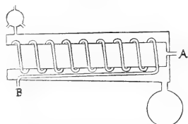
Thermostaten-Luftbad nach Simu.
