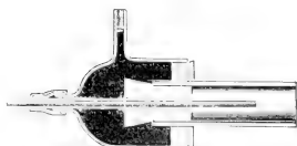
Quecksilberdichtung eines Kautschukstopfens.
