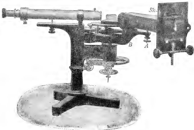
Prismenspektrograph nach F. Löwe .
