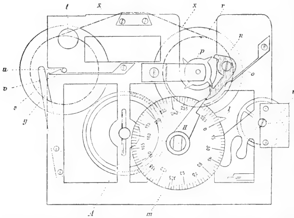
Die innere Konstruktion des selbstregistrierenden Photometers von Samec und Jenčić.
