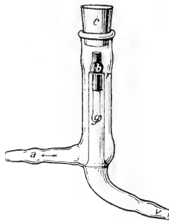
Rückschlagventil nach Kumm .
