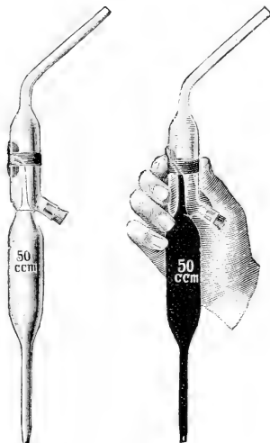
Sicherheitspipette mit automatischer Null- punkts-Einstellung.
