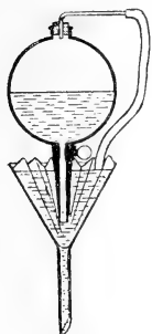
Automatisches Filtrieren nach Hamlin.
