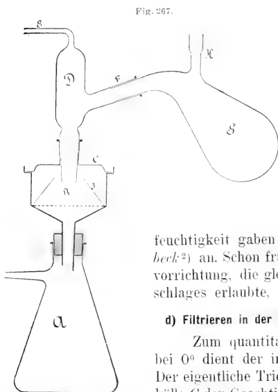
Filtrierapparat für hygroskopische und luftempfindliche Substanzen nach Steinkopf.
