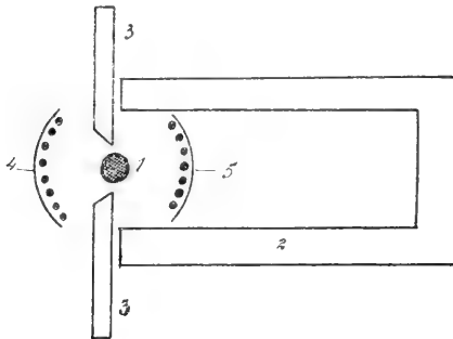
Congdonsche Versuchsanordnung. 1 = Radiumröhrchen, 2 = Bleirohr, 3 = Schirm, 4, 5 = Gestell mit Samen.
