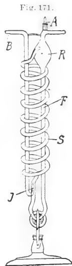
Absorptionsvorlage nach Berl.
