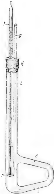
Schmelzpunktbestimmungsapparat nach Anthes.
