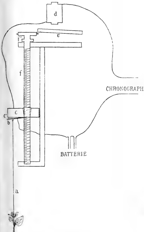
Die Skizze zum Präzisionselektroanemometer nach Borie.
