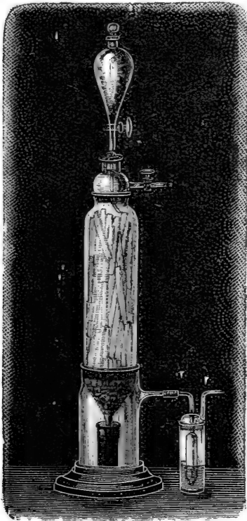
Gasentwicklungsapparat nach Griggnier.
