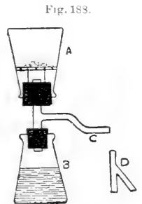
Gasentwicklungsapparat nach Hodges (Kipp-System).
