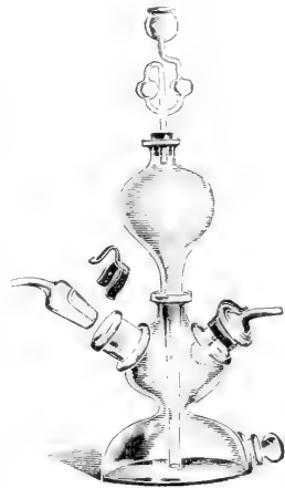
Gasentwicklungsapparat nach Kipp-Preuss.
