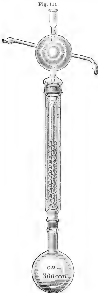
Apparat zur Extraktion von Lösungen nach Kempf (1. Modell).
