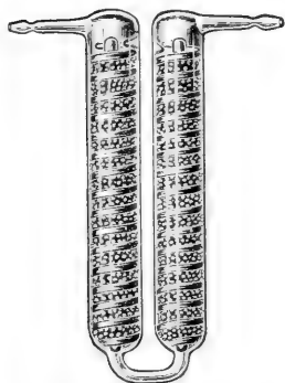
U-Rohr mit Flachglasspiralen nach Fleissner.
