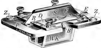
Ansicht einer Wasser- resp. Flüssigkeitskammer. Gegen Verdunstung ist die Flüssigkeit durch einen Glasdeckel D geschützt.
