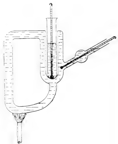
Schmelzpunktbestimmungsapparat nach Holleman, Hartogs und van der Linden.
