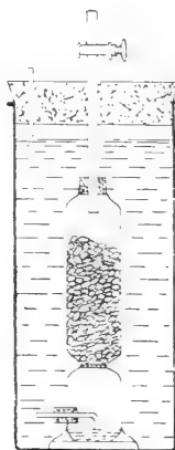
Gasentwicklungsapparat nach Vernon .
