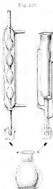
Apparat zur Extraktion fester Körper nach Klopstock .
