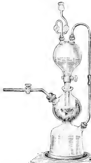
Gasentwicklungsapparat nach Wartha.
