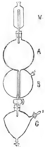
Gasentwicklungsapparat nach Sklepinski .
