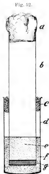
Apparat von Schmidt. a = Wattehausch. b = Reagenzrohr (Gasglühlichtzylinder). c = Wattering. d = Becherglas. e, f = Sandschichte. g = Zelloidinschicht.
