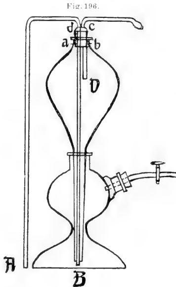
Entleerröhre für Kipp sche Apparate nach Friedmann .
