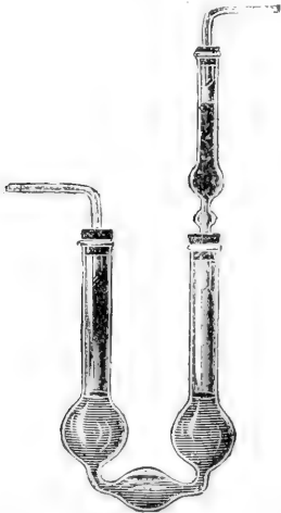
Absorptionsvorlage nach Péligot.
