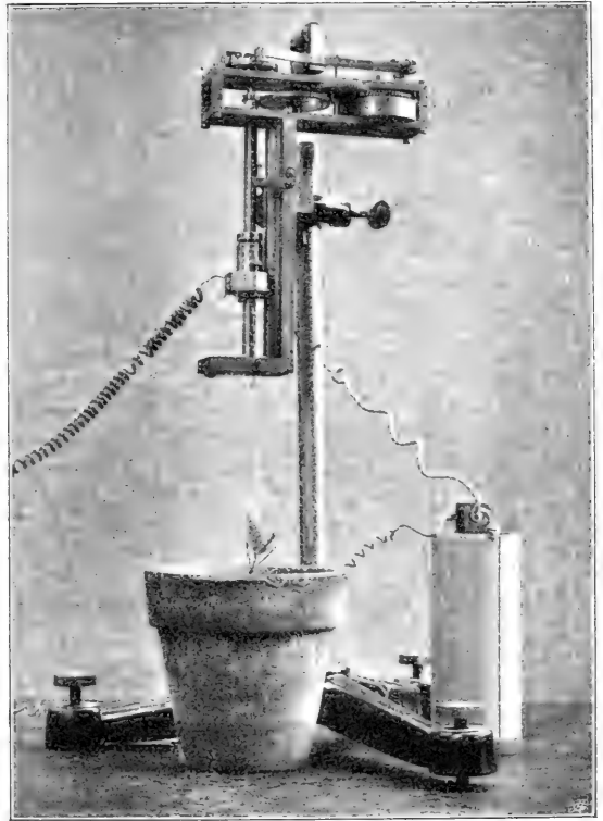
Anemometervorrichtung des elektrischen Präzisionsanemometers nach Borie. (Original-Photographie von Prof. Borie.)
