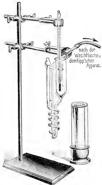
Erstarrungspunktbestimmungsapparat nach Stollzenberg.
