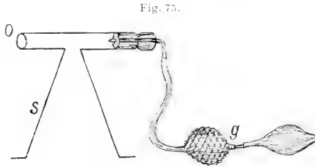
Fig. 75. Hürthles Rußzerstäuber (aus Langendorff, Physiolog. Graphik).
