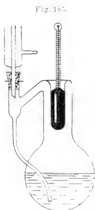
Siedepunktbestimmungsapparat nach Kablukow, Solomonow und Galine.
