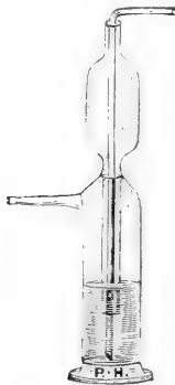
Sicherheitswaschflasche nach Mauthner.
