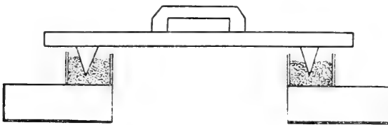
Sandverschluß des Ätherisierungskastens nach Aynard.
