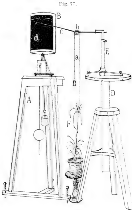
Fig. 77. Auxanometer nach Sachs (Vorles. über Pflanzenphysiologie, 2. Aufl.).
