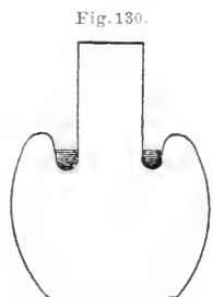
Stehkolben mit Quecksilberrinne nach Knorr .
