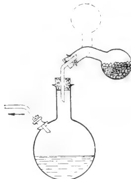
Apparat zur Entwicklung von Jodwasserstoffgas nach Étard (Gasentwicklungsapparat nach dem Einwurfsystem).
