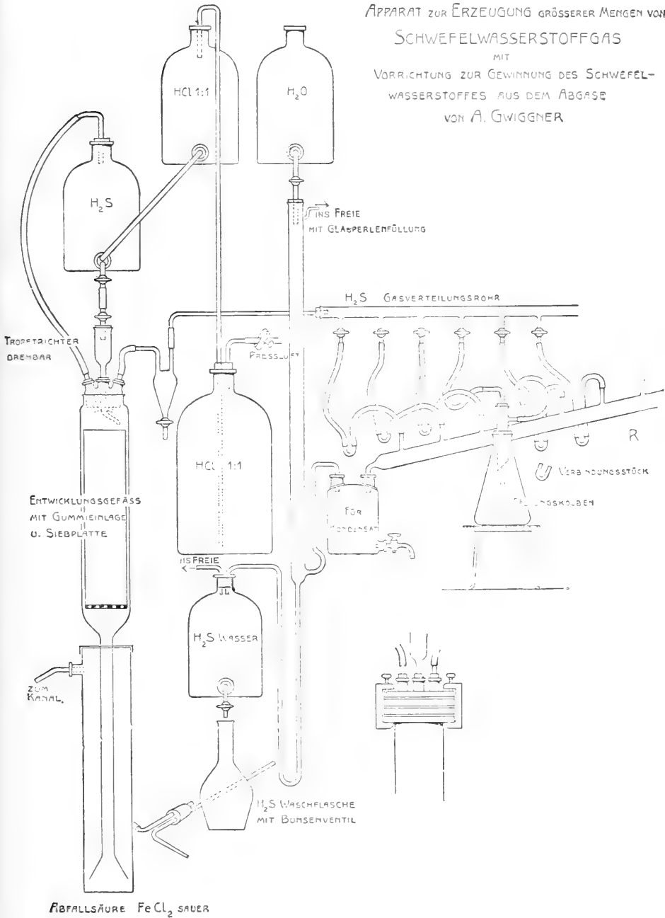
Gasentwicklungsapparat nach Gwignier.
