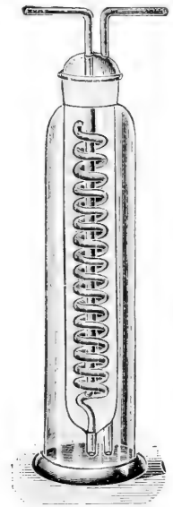
Waschflasche nach Hahn.
