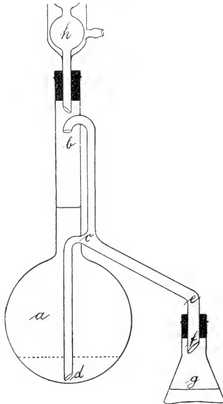
Apparat zur Extraktion von Flüssigkeiten nach Berlin .
