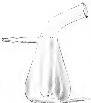
Absorptionsvorlage nach Stock .
