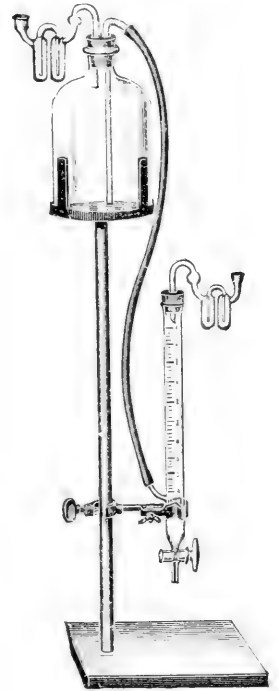
Luftwaschaufsatz nach Göckel in Verbindung mit einer Titrirvorrichtung.
