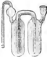
Luftwaschaufsatz nach Göckel.
