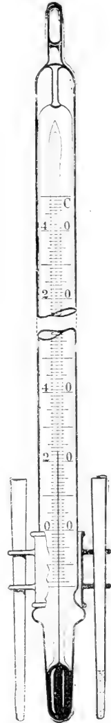
Schmelzpunktbestimmung nach Th. Weyl .
