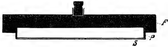
Baarsches Strahlenfilter für Lichtkeimungsversuche im Querschnitt. F = Filter (Farblösung), P = Petrischale, S = schwarzes Papier zum Abhalten des Lichtes.
