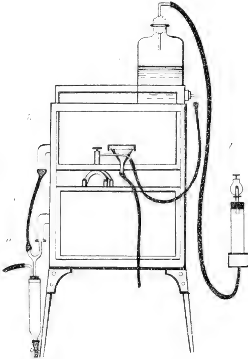
Waschapparat nach Archovskij. (Beschreibung im Text.)
