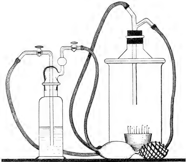
Apparatur von Molisch zur Behandlung von Keimpflanzen mit Radiumemanation.
