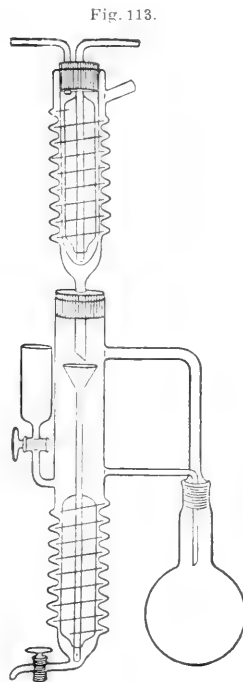
Apparate zur Extraktion von Lösungen nach Friedrichs .
