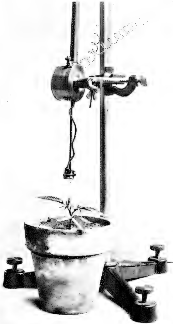
Die neue Form vom elektrischen Auxanometer nach Bovie . (Original von Prof. Bovie .)
