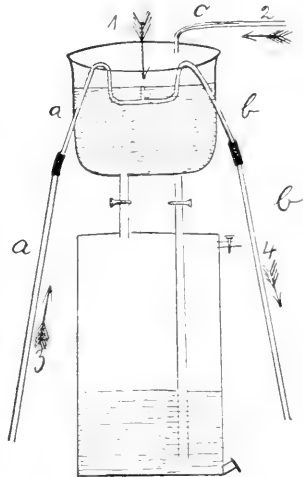
Überlaufverhinderung bei Gasometern nach Wästenfeld .
