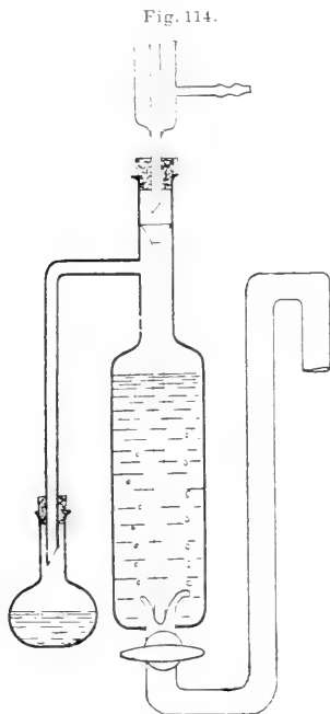
Apparat zur Extraktion von Lösungen nach Koolmann .
