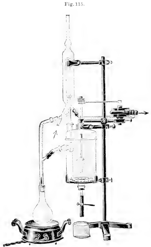
Apparat zur Extraktion von Lösungen nach Zelmanowitz , verbessert von Tolmacz .
