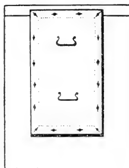
Abhebbarer Deckel des Johann schen Ätherisierungsgefäßes.
