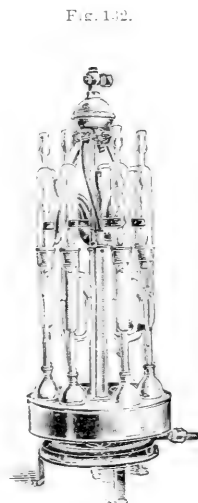
Praktische Anordnung von Soxhlet-Apparaten bei Reihensextraktionen nach Möllinger .
