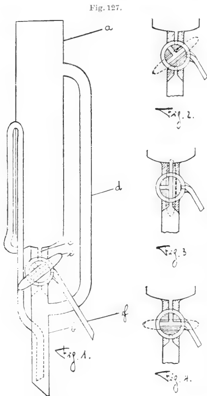
Apparat zur Extraktion fester Körper nach Schmid.
