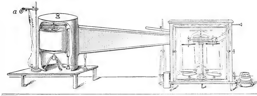
Vorderansicht der Gewichts- und -abnahmen automatisch registrierenden Wage.
