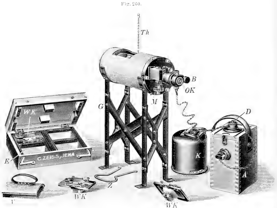
Gesamtansicht des Flüssigkeits-Interferometers in Gebrauchslage. A der Akkumulator. K Schutzkappe. I Verschlussdeckel. WK Wasser-(Flüssigkeits-)Kammer. Z Klammer zum Herausnehmen des Akkumulators aus dem Holzkasten.
