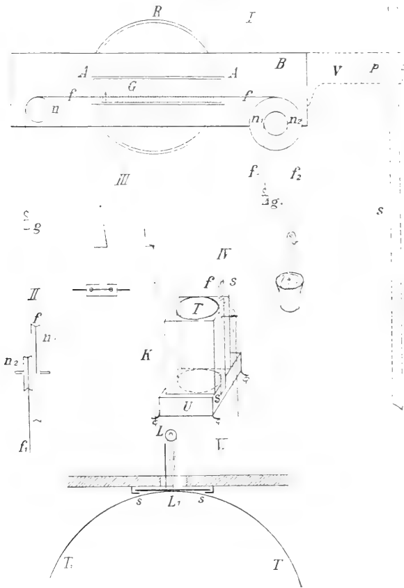
Projektionsauxanometer nach Kohl (I, II, III), photographische Registriermethode nach Kohl (IV, V).
