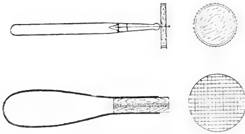
Markierer nach Ganong (Plant Physiology, 1908).
