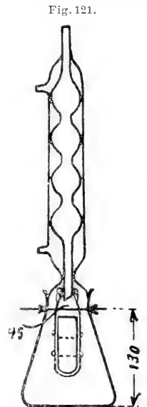
Apparat zur Extraktion fester Körper nach Gräfe-Holde-Meyerheim.
