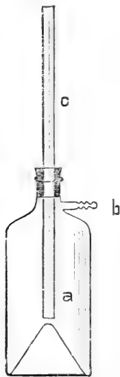
Gasentwicklungsapparat nach Küspert (Einwurfmethode).
