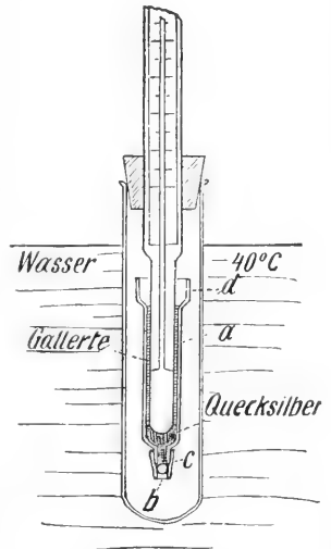
Schmelzpunktbestimmung von Gelatine nach Herold.
