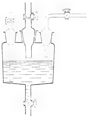
Gasentwicklungsapparat nach Köhlenz (Einwurfsystem).
