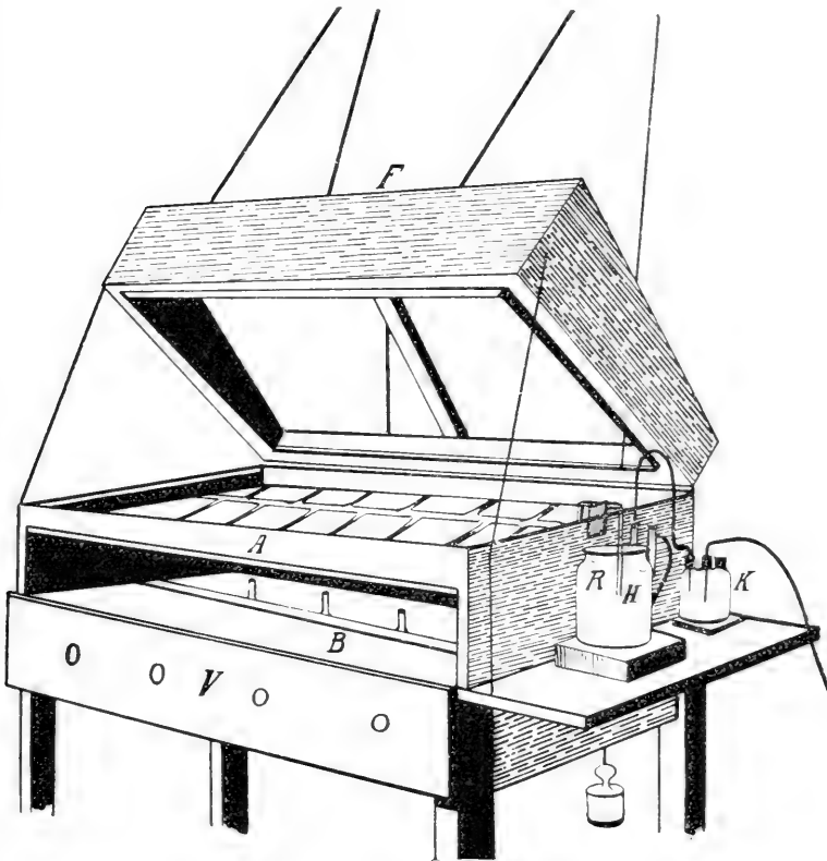
Keimapparat von Hoderwald. (Beschreibung im Text.)
