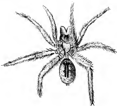
Fig. 922. Argyroneta antiqua Heyden. Oligocäne Braunkohle. Rott bei Bonn. 2/4. (Nach Heyden.)
