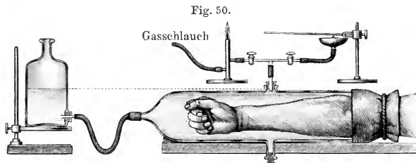
Plethysmograph nach Mosso.
