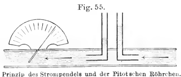
Prinzip des Strompendels und der Pitotschen Röhren.
