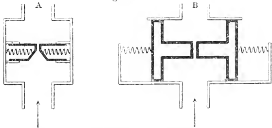
Zwei Polsterpfeifen (Gegenschlagpfeifen), nach Ewald.
