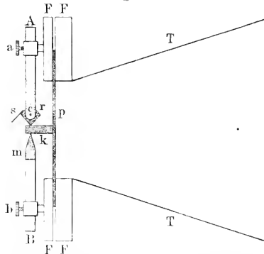
Apparat zur Projektion und Registrierung der Stimm- und Schwingungen, nach Samojloff.
