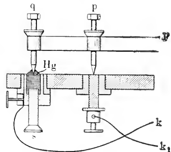
Helmholtz'scher Doppelkontakt mit Quecksilbertaden modifiziert von du Bois-Reymond.
