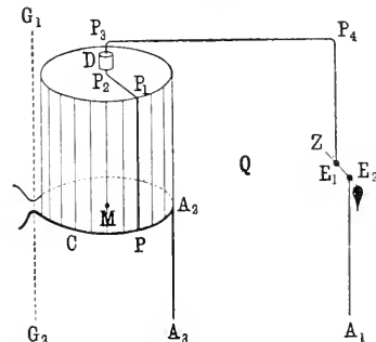
Detail zur Versuchsordnung Einthovens.
