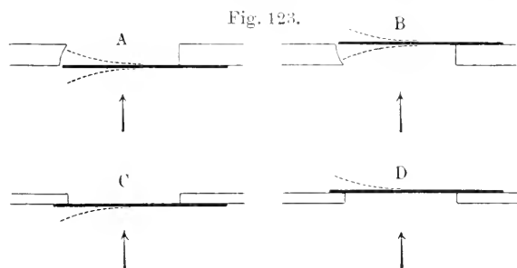
Schemata der vier Formen von Zungenpfeifen, nach Ewald. A durchschlagend einschlagend. B durchschlagend ausschlagend. C aufschlagend, einschlagend. D aufschlagend, ausschlagend.
