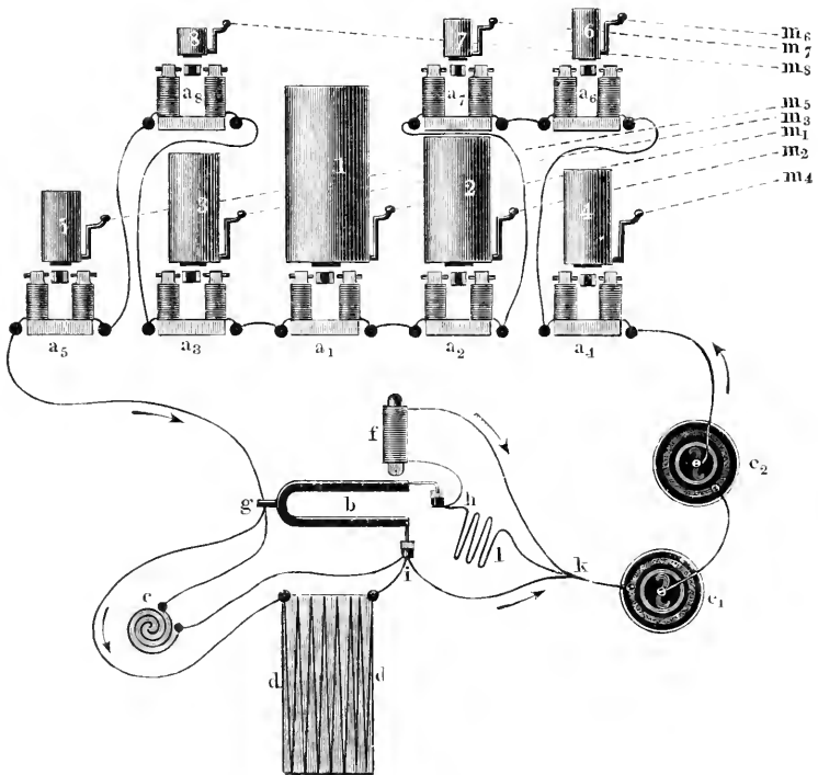
Helmholtz' Stimmabelapparat zur Vokalsynthese.
