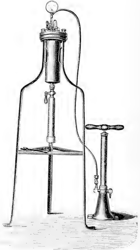
Fig. 76. Chamberland-Filter, mit Druckluftpumpe (rechts) montiert. — Ca. ein Zehntel der nat. Größe.
