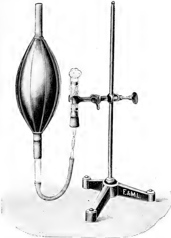
Fig. 75. Luftuntersuchungs-Apparat nach FICKER, bestehend aus der Ballonpumpe (links) und dem mit Glassand beschickten Filtrerröhrchen (rechts).
