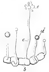
Fig. 54. Chlamydomucor racemosus BREFELD. Kette von fünf Chlamydosporen, welche je einen Sporangiumträger hervorgetrieben haben. Das Spora- ngium von d ist noch unreif. Das von c ist schon zerstört; nur die Columella c und acht Sporangiumsporen sind noch vorhanden. — Vergr. 120. Nach BREFELD.
