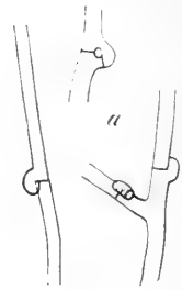
Fig. 34. Schnallenverbindung im Mycel von Hypochnus cen- trifugus . — Vergr. 390. Nach TULASSE.
