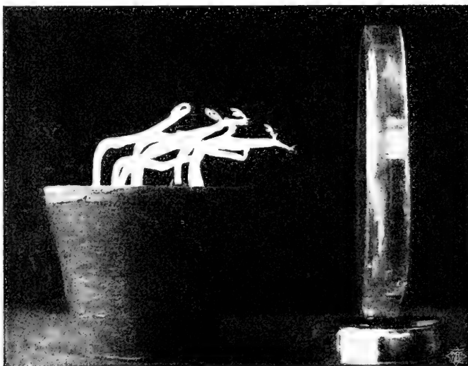
Fig. 95. Positiver Heliotropismus von Erbsenkeimlingen, hervorgerufen durch das Licht einer in der Petrischale (rechts) befindlichen Strickkultur von Bacterium phosphoreum (COHN) MOLISCH. Alle Keimlinge erscheinen zum Bakterienlicht hin positiv heliotropisch gekrümmt.
