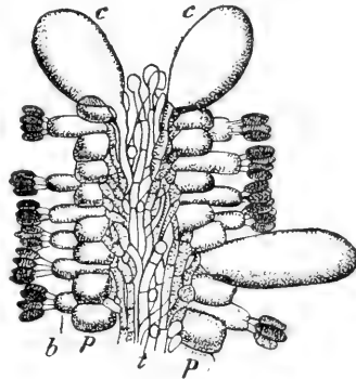
Fig. 36. Coprinus stercorarius . Stück eines Längsschnittes von einer Lamelle, t Trama, p die kleinen Paraphysen, c Cystiden, b Basidien mit ihren vier Basidiosporen. — Nach BREFELD.
