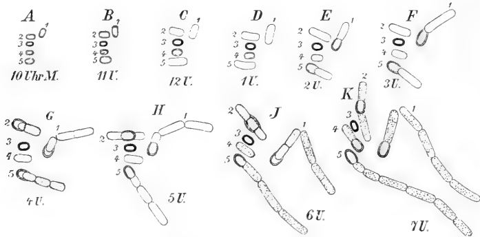
Fig. 18. Sporenkeimung bei Bacillus sessilis .
