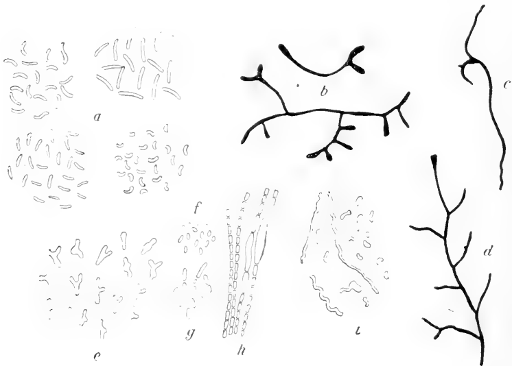
Fig. 5. Zellgestalten einiger Bakterienarten.
