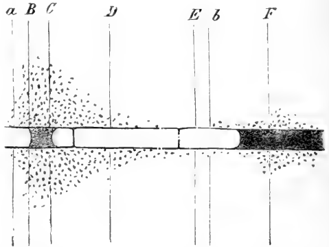
Fig. 68. Sauerstoffliebende Bakterien, einen Algenfaden umschwärmend, der in einem Mikrospektrum liegt. Die Chlorophyllkörner des Inhalts der Algenzellen sind nicht eingezeichnet, wohl aber die Spektrallinien, um die Lage des Spektrums zu bezeichnen. — Vergr. 200.
