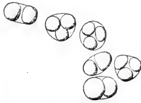
Fig. 45. Carlsberg Unterhefe Nr. 2. Einer Zucht auf Würzelgelatine entnommene Zellen, in denen je 2 oder 3 Ascosporen sich gebildet haben. — Vergr. 1000. Nach HANSEN.
