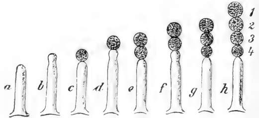
Fig. 47. Schema der Konidienbildung nach Typus I. Erklärung im Text. — Nach ZOPF.
