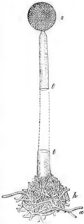
Fig. 56. Mortierella Rostafinskii BREFELD.
