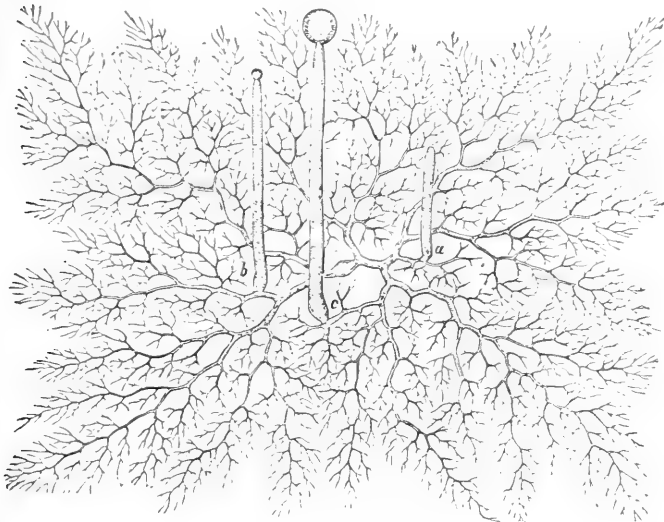
Fig. 28. Thallus von Mucor mucedo .
