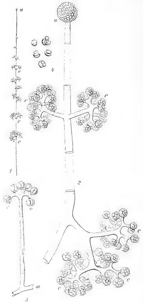
Fig. 44. Thamnidium elegans LINK.
