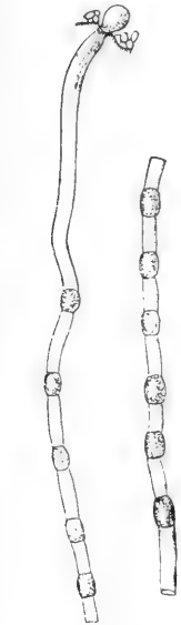
Fig. 51. Chlamydomucor racemosus BREFELD. Rechts ein Stück einer Mycelhypha mit sechs Chlamyosporen. Links ein Sporangiumträger mit fünf Chlamyosporen; am Scheitel die Columella, einige Sporangiumsporen und die Reste der durch Präparation zum größten Teile entfernten Sporangiummembran. — Vergr. 80. Nach BREFELD.
