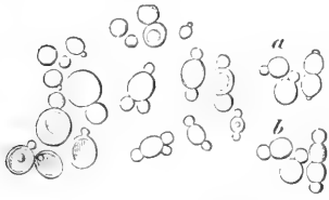
Fig. 32. Torula-Art in Bierwürze wachsend. In a eine Gruppe sprossender Zellen, deren Zustand nach Ablauf einer Stunde in b dargestellt ist. — Vergr. ca. 1000. Nach HANSEN.
