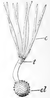
Fig. 60. Tilletia tritici (Stinkbrand des Weizens). Keimende Chlamydospore ( cl ) mit kurzem Keimschlauch ( t ) (Konidienträger), der nur an der Spitze Konidien trägt ( c ). — Vergr. 300. Nach BREFELD.
