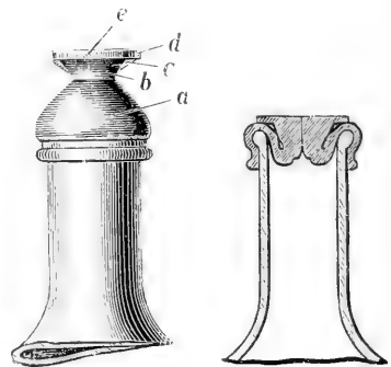
Fig. 73. Gummikappen-Verschluß nach A. SUTZER, links vor dem Sterilisieren, rechts eingezogen) nach dem Sterilisieren und Abkühlen. e der enge Schlitz. — Nat. Größe.
