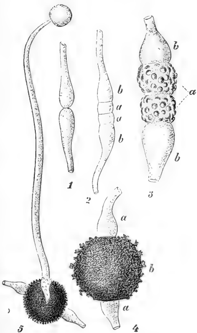
Fig. 39. Mucor mucedo . Bildung der Zygospore. 1 zwei Hyphenenden in Scheitelberührung. 2 Gliederung in Gamete a und Suspensor b . 3 Fusion der Gameten a ; Membran verdickt sich. 4 Reife Zygospore b von den Suspensoren ( a, a ) getragen. — Vergr. von (1—4) 225. 5 Auskeimung der Zygospore zu einem Sporangienträger. — Vergr. ca. 60. Nach BREFELD.
