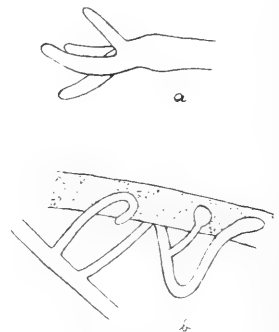
Fig. 71. a, Unregelmäßiges Auswachsen der Hyphenenenden von Sclerotinia trifoliorum auf Grund eines von benachbartem Mucor -Mycel ausgeübten Reizes. b, Anfangsstadium der knäuelartigen Umschlingung eines Mucor -Fadens seitens der Sclerotinia . In der Mucor -Hyphne ist der Zellinhalt angedeutet. — Nach REINHARDT.
