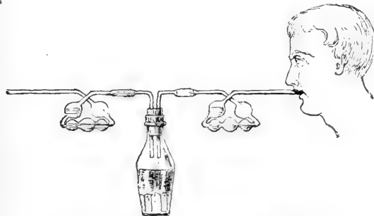
Fig. 2. Versuch von FRANZ SCHULZE.
