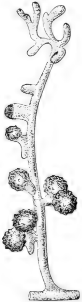
Fig. 41. Mucor tenuis BAINIER. Azygosporen in verschiedenen Stufen ihrer Ausbildung. — Nach BAINIER.
