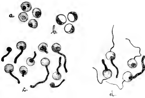
Fig. 62. Plasmoptyse der Cholera-Vibrien in einer 3—4 Tage alten Agarzucht (Peptonzuckeragar mit 0,5 Proz. Kochsalz) bei 30°. a Einzelne Plasmoptysekugeln mit stark färbaren Körnchen, mit Gentianaviolett gefärbt. b Lebende, noch sich bewegende Kugeln mit 2 Proz. Kochsalz plasmolysiert, der Inhalt halbmondformig kontrahiert (schwarz). c Verschiedene Stadien der Plasmoptyse, das Hervorquellen des Inhalts aus den Vibriolen zeigend; Färbung mit Gentianaviolett. d Geißelfärbung nach LOEFFLER, Geißeln an den Kugeln. — Vergr. 1500. Aus A. FISCHER, Vorlesungen, 2. Aufl.
