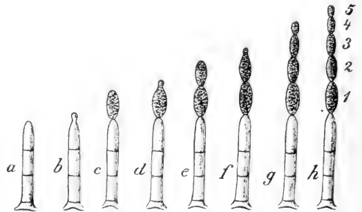
Fig. 48. Schema der Konidienbildung nach Typus II. Erklärung im Text. Nach ZOPF.
