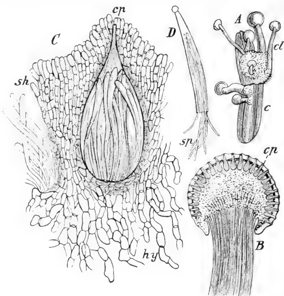
Fig. 58. Claviceps purpurea TUL. (Mutterkorn).
