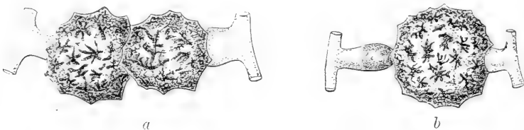
Fig. 40. Azygosporenbildung bei Mucor erectus . Nach BAINIER.
