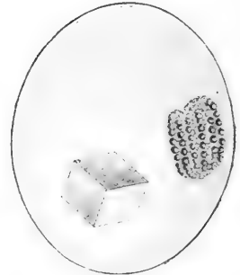
Fig. 19. Krystalloid in der Vakuole einer Preihefenzelle. Daneben befindet sich ein dichter Knäuel von Granulis. — Vergr. 4400. Nach HIERONYMUS .
