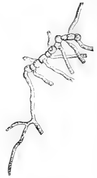
Fig. 53. Chlamydomucor racemosus BREFELD. Vegetative Keimung eines Verbandes von elf Oidien. Vergr. 80. Nach BREFELD.
