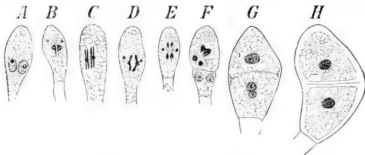
Fig. 22. Puccinia liliacearum . A Ende einer sporogenen Hyphle. B—E Kernteilungsstadien darin. F, G junge Teleutosporen mit Vereinigungsstadien der Kerne. H reife Teleutospore. — Nach POIRAULT und RACIBORSKI.
