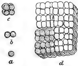
Fig. 8. Sarcina ventriculi . Aus dem Mageninhalt eines Magenkranken. a—d verschiedene Entwicklungsstufen. — Nach ZOPF.
