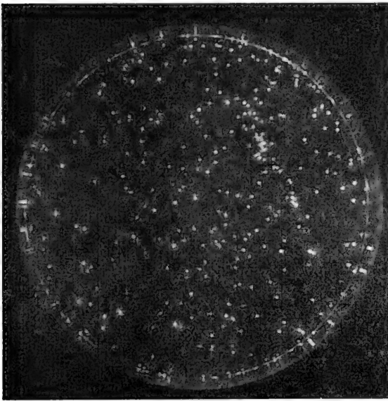
Fig. 93. Photographie leuchtender Kolonien von Bacterium phosphoreum (COHN) MOLISCH in ihrem eigenen Lichte. Die Kolonien waren sechs Tage alt und befanden sich in einer Petrischale, deren Umgrenzung in der Photographie auch zu sehen ist. Expositionszeit 15 Stunden.
