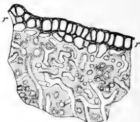
Fig. 38. Sclerotinia Fuckeliana . Stück eines dünnen Querschnittes durch ein Sklerotium. r das Rindengewebe, nach innen Prosoplectenchym. — Vergr. 390. Nach DE BARY.
