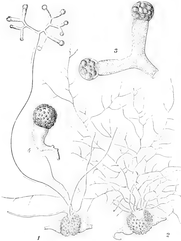
Fig. 52. Sporodinia aspergillus SCHRANK. 1 Fructifikativ keimende Zygospore. — Vergr. 40. Nach BREFELD. 2 Vegetativ keimende Zygospore. — Desgl. 3 Zwei Sporangien dieses Fruchtkörpers in reifem Zustande. — Vergr. 150. Nach DE BARY. 4 Azygospore. — Vergr. 90. Nach v. TAVEL.
