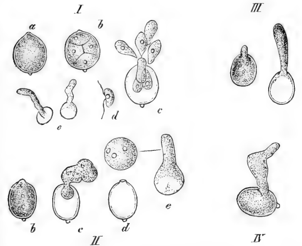
Fig. 55. Keimung der ungeschlechtlichen Sporangien von Peronosporaceen. I Plasmopara nivea UNG.; in a das abgefallene Sporangium, in b Teilung seines Inhaltes, c Austritt der Schwärmsporen d, in e deren Auswachsen. II Plasmopara densa RABH.; in b beginnende Teilung des Inhaltes, c und d Austritt desselben, in e sein Auswachsen zum Keimschlauch. III Bremia lactucae UNG.; das Sporangium ist zur Konidie geworden, die nur am Scheitel auskeimt. IV Peronospora radii DE BY.; die Konidie keimt auch seitlich aus. Vergr. 400. Nach DE BARY.
