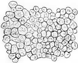
Fig. 35. Boletus edulis . Längsschnitt (oben) und Querschnitt (unten) durch den Stiel des Fruchtkörpers (Hutes) des Steinpilzes ( Boletus edulis ). — Vergr. 300. Nach STRASBURGER.
