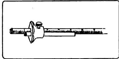
Fig. 217. Roller Mortise-Gage.
