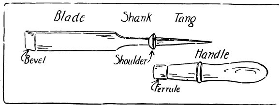
Fig. 65. Firmer-Chisel.
