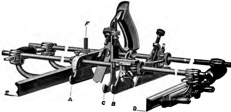
Fig. 117. Universal Plane.
