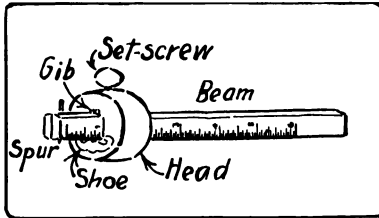
Fig. 211. Marking-Gage.
