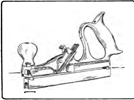
Fig. 115. Tonguing-and-Grooving-Plane.
