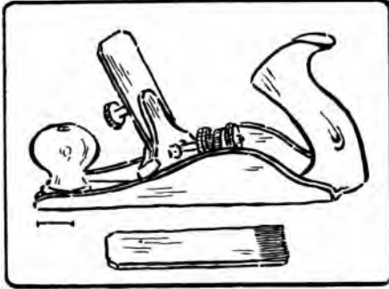
Fig. 111. Scratch-Plane and Scaper-Plane.
