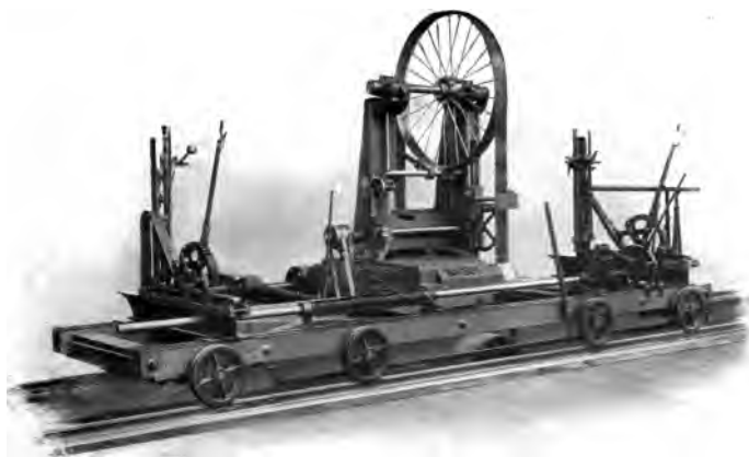
Fig. 34. Band-Saw.
