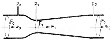
Fig. 63. Venturirohr.
