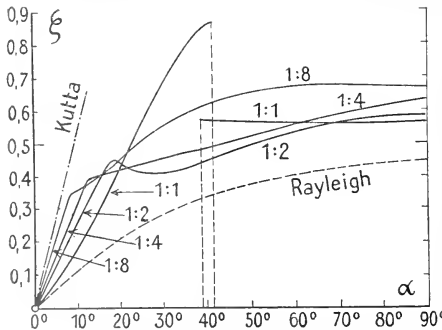
Fig. 78. Gesamtwiderstand von ebenen Flächen.
