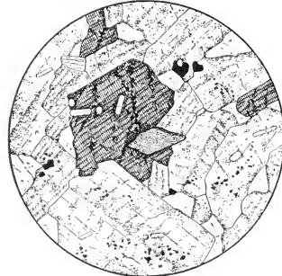
Fig. 2. Hornblendesyenit. Meißen. Feldspat trübe, Hornblende dunkel, in der Mitte Titanit. Vergrößerung 15.
