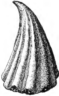
Fig. 13. † Orthonychia elegans Barr. Ober-Silur. Lochkow, Böhmen. Nach Zittel.
