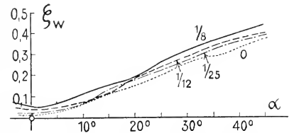
Fig. 80. Widerstand von gewölbten Flächen.
