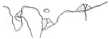
Ozeanische Deltas.
