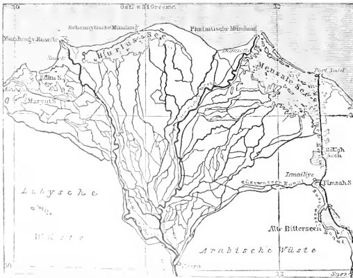
Fig. 36. Nildelta. Aus Supan, Grundzüge der physischen Erdkunde.
