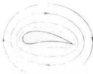
Fig. 20. Zirkulante Strömung.
