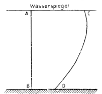
Fig. 1b. Linien gleicher Geschwindigkeit i. Längsprofil. v. Z. nach Brückner.
