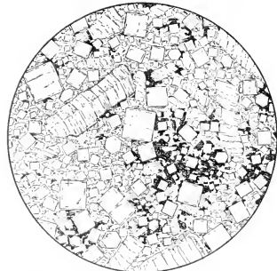
Fig. 7. Nephelin-Phonolith. Brüx, Böhmen. Rechtecke von Nephelin, lange Schnitte von Sanidin, Aegirin dunkel. Vergrößerung 35.
