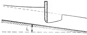
Fig. 69. Fluß.
