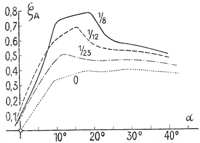
Fig. 79. Auftrieb von gewölbten Flächen.
