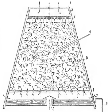
Fig. 5. Gefäß für die Alkoholoxydation nach der deutschen Methode. 1 Deckel. 2 Alkoholische Flüssigkeit. 3 Fehlboden. 4 Thermometer. 5 Sägespäne. 6 Fehlboden. 7 Lüftungssofen. 8 Siphon zum Abzapfen des gewonnenen Essigs. 9 Lüftungsöffnung.
