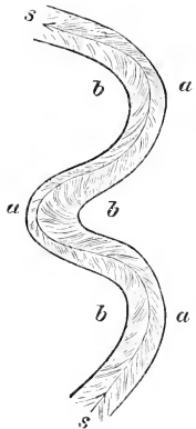
Fig. 2. Lage des Stromstrichs in Krümmungen. Aus Supan, Grundzüge der physischen Erdkunde.
