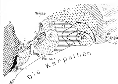
Fig. 12. Das Vorland der Westkarpathen unter Weglassung der transgredierenden Schollen. Ueberdeckung des variszischen Bogens durch die Decken der Karpathen. Arch Archäikum, d Devon, Cu Unter-, Ca Oberkarbon, p Rotliegendes, tr Trias, j Jura, cr mittlere und obere Kreide, sy Syenit. Nach E. Sueß
