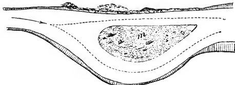
Fig. 10. Ablagerung in einer Flussweitung. Aus v. Neumayr; Anleitung zu wissenschaftlichen Beobachtungen auf Reisen.
