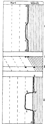
Fig. 21. Seitenverschiebung eines Flusses. v. Zahn. Nach v. Richthofen.
