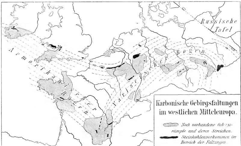
Fig. 23. Der armorikanische und der variszische Gebirgsbogen. Ihre Scharung im französischen Zentralplateau. Nach E. Kayser.
