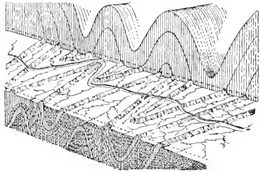
Fig. 26. Schematische Ansicht, welche darstellt, wie aus einem Faltengebirge (im Hintergrunde) durch Abtragung ein Rumpfigebirge (im Vordergrunde) entsteht. Seine Rumpffläche, deren Niveau durch die gestrichelten Linien angedeutet ist, ist durch Flußläufe zerschnitten. Nur die Züge von hartem Gestein ragen empor, wobei der Faltenbau noch zum Ausdruck kommt. (Motiv: Alleghanies.) Nach W. M. Davis und G. Braun.
