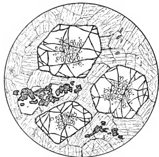
Fig. 11. Eklogit. Fattigau, Fichtelgebirge. Große, einschlußreiche Granate, Omphacit (reich an Spaltrissen), Rutil (dunkel). Vergrößerung 15.
