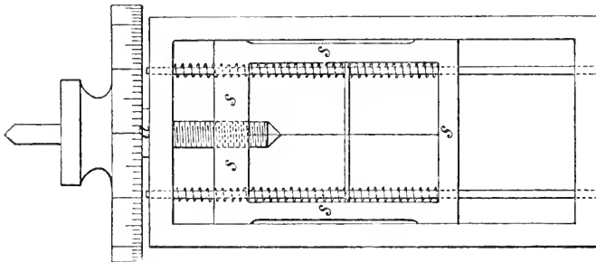
Mikroskopmikrometer nach C. BAMBERG. (A. 301.)
