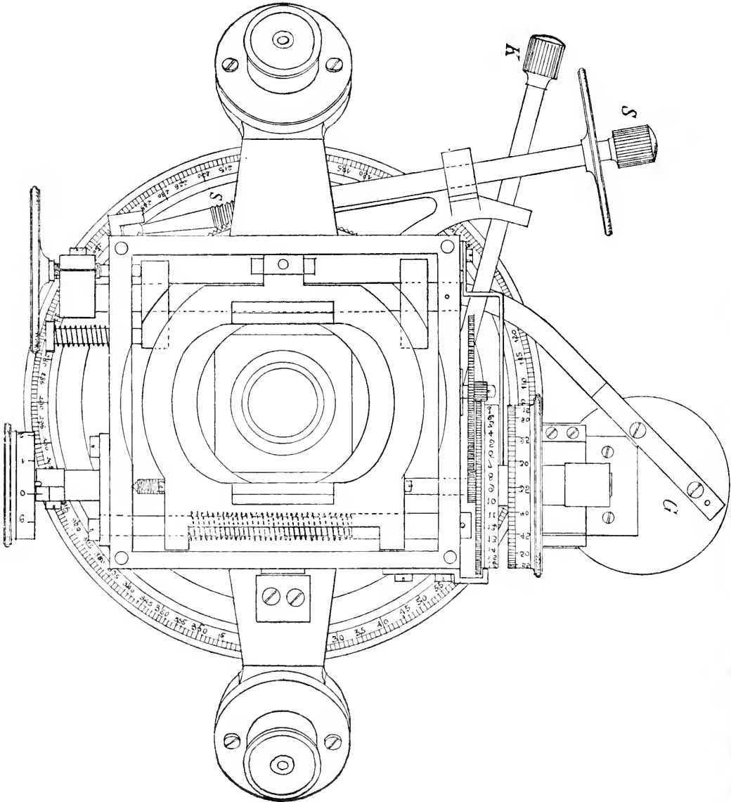
Positionsmikrometer von A. REPSOLD &amp; Söhne (Sternwarte Strassburg). Bem. Die Theilung des Kreises geht in Wirklichkeit von 10 zu 10 Minuten und jede zweite Gradzahl ist numerirt.
