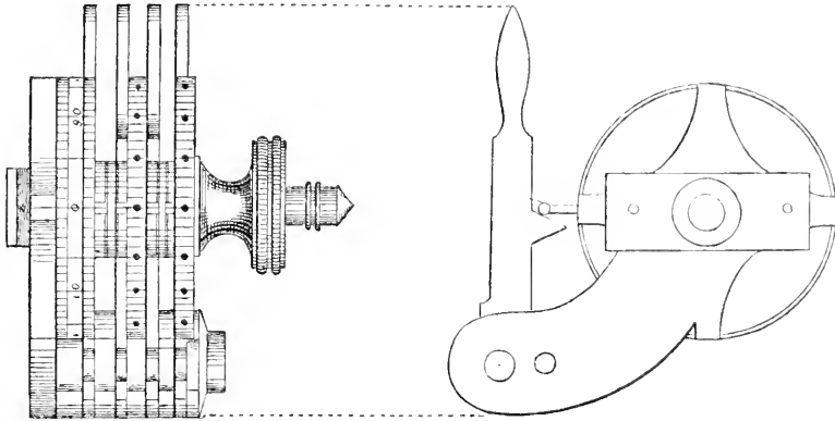
Registrirvorrichtung nach J. A. ROGERS.
