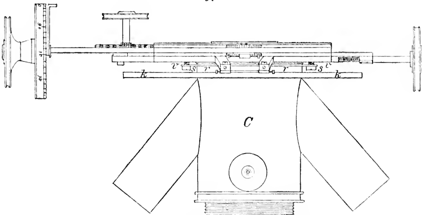
Positionsmikrometer von FRAUNHOFER.
