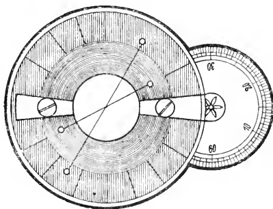
Cross-hair-Mikrometer von W. HERSCHEL.
