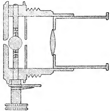
(A. 345.) Doppelbildmikrometer von G. DOLLOND.
