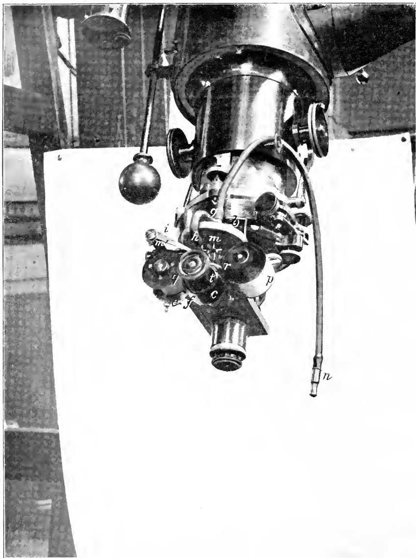
Declinograph nach V. KNORRE, construirt von R. FUESS (Sternwarte Berlin) (A. 312)
