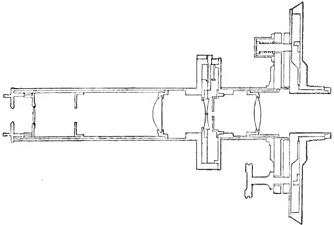
AIRY's Doppelbildmikrometer
