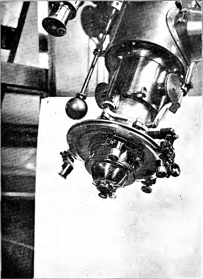
Doppelbildmikrometer nach V. WELLMANN
