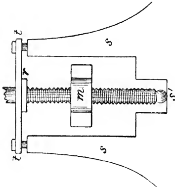
Lagerung der Schraube nach FRAUNHOFER. (A. 300.)
