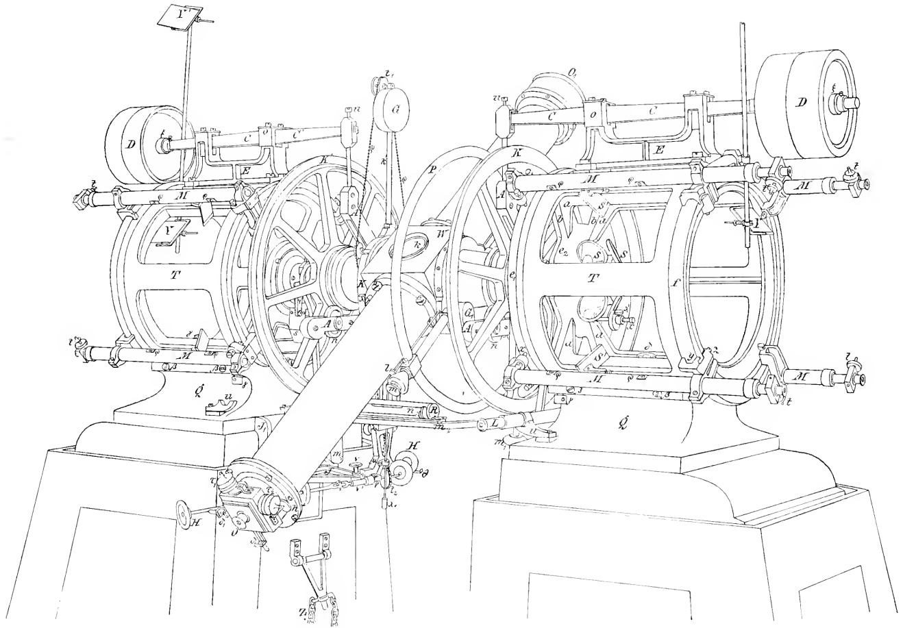
Repsold'scher Meridiankreis
