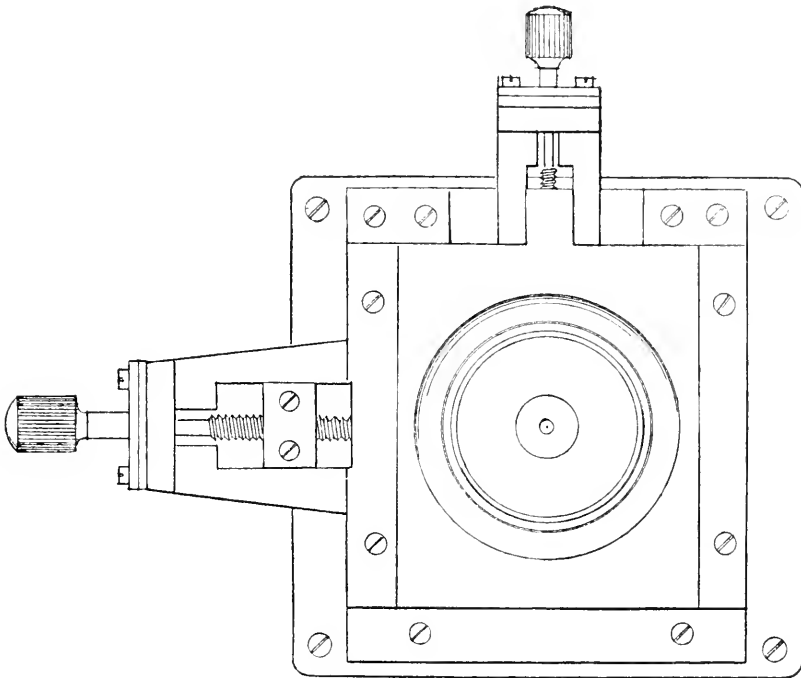
Ocularschiebplatte.
