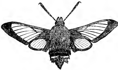
Fig. 116.— Sphinx fuciformis .
