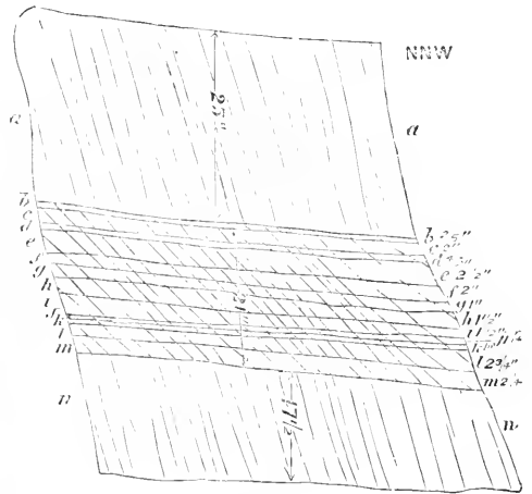
Fig. 144.
