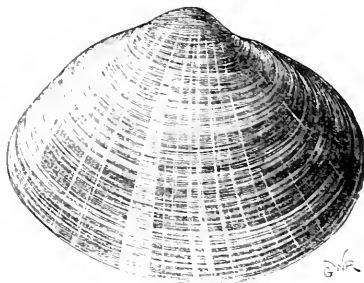
Fig. 5.— Macra stultorum .
