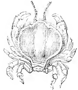
Fig. 132.— Thia polita .
