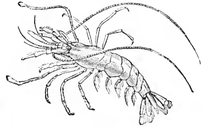
Fig. 131.— Nika edulis .
