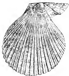
Fig. 4.— Pecten varius .
