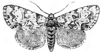
Fig. 113.— Diphthera Orion.
