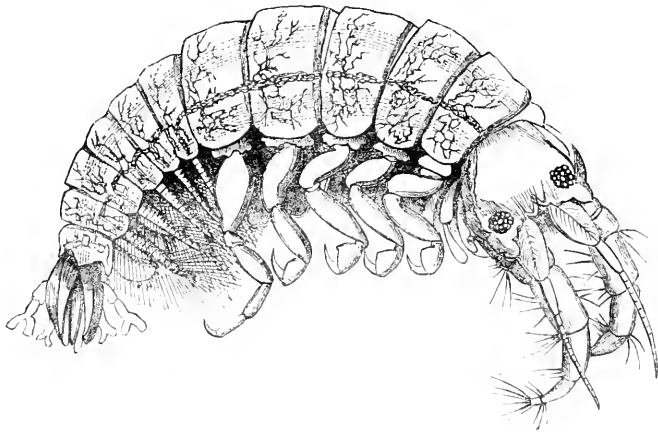
Fig. 89.— Corophium crassicornes × 25.
