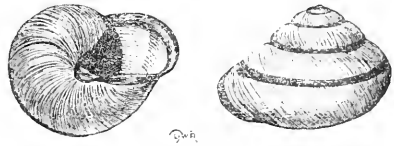
Fig. 118.— Helix nemoralis .
