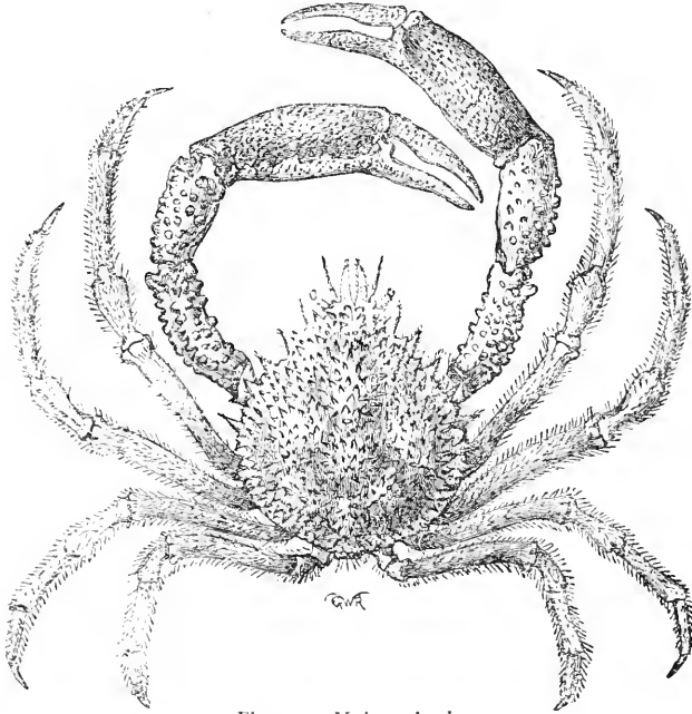
Fig. 129.— Misi squinado .
