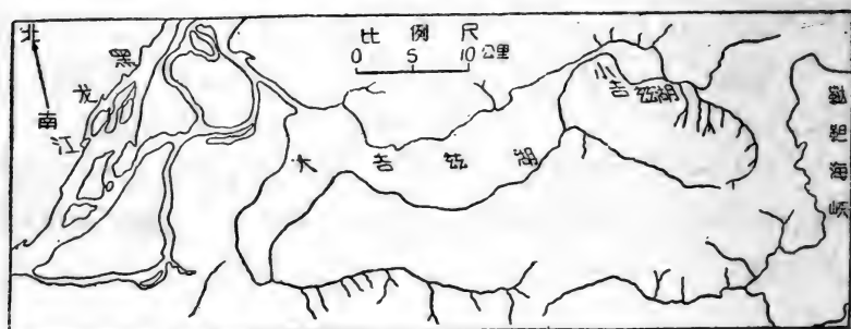
25. 大吉兹湖—鞑靼海峡运河平面图
