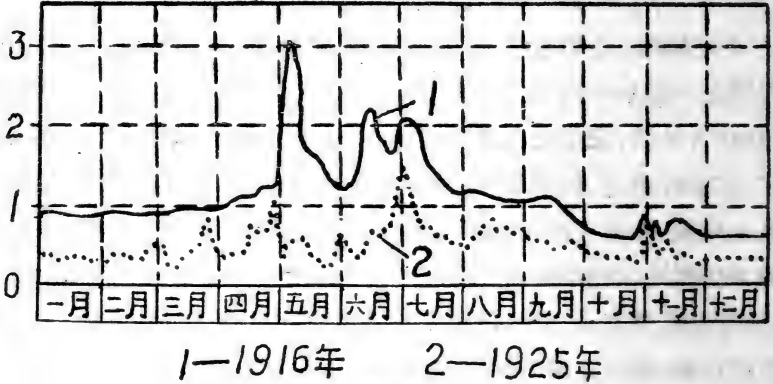
13. 額尔古納河鄂洛赤站水位过程綫图
