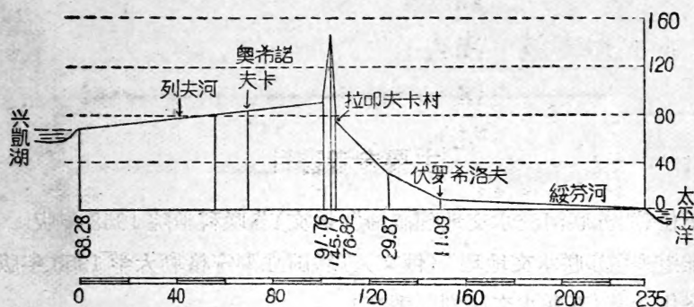
28. 兴凯湖—大彼得灣运河縱剖面图。
