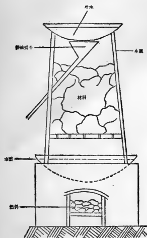
木質蒸餾器裝置示意圖
