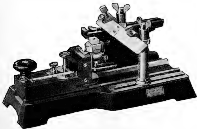
FIG. 36.—Base Sledge Microtome
