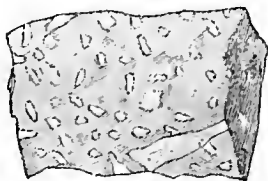
Fig. 7. Pórfido.
