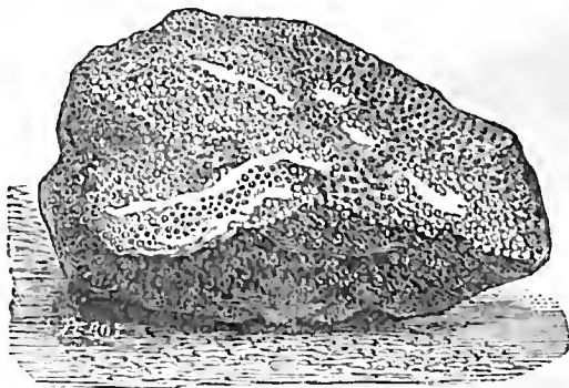
Fig. 2. Caliza oolítica .
