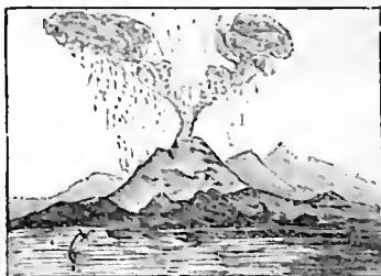
Fig. 18. Volcán.
