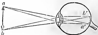
Fig. 139. — Curso de los rayos luminosos en el ojo.
