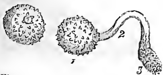
Fig. 126. — Granos de polen vistos con el microscopio.
