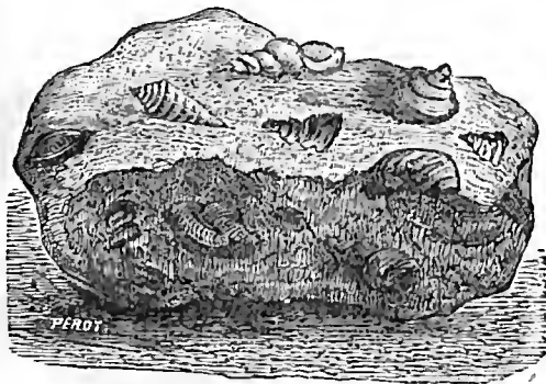
Fig. 1. — Caliza común.
