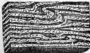
Fig. 10. Gneis .
