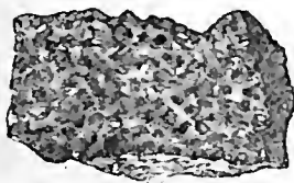
Fig. 6. Granito.
