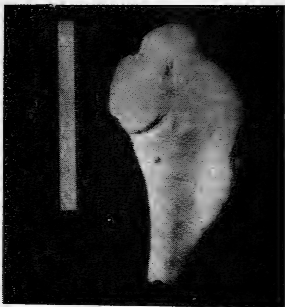
Фиг. 2. Проксимален фрагмент от дясна раменна кост на дропла ( Oreotyx variegatus ) (сн. В. Назан)
