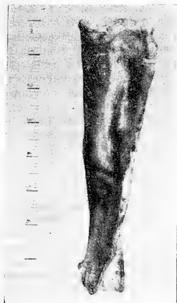
Фиг. 5. Aquila chrysaetos — tarsometatarsus sinistra (сн. Виктор Хазан)
