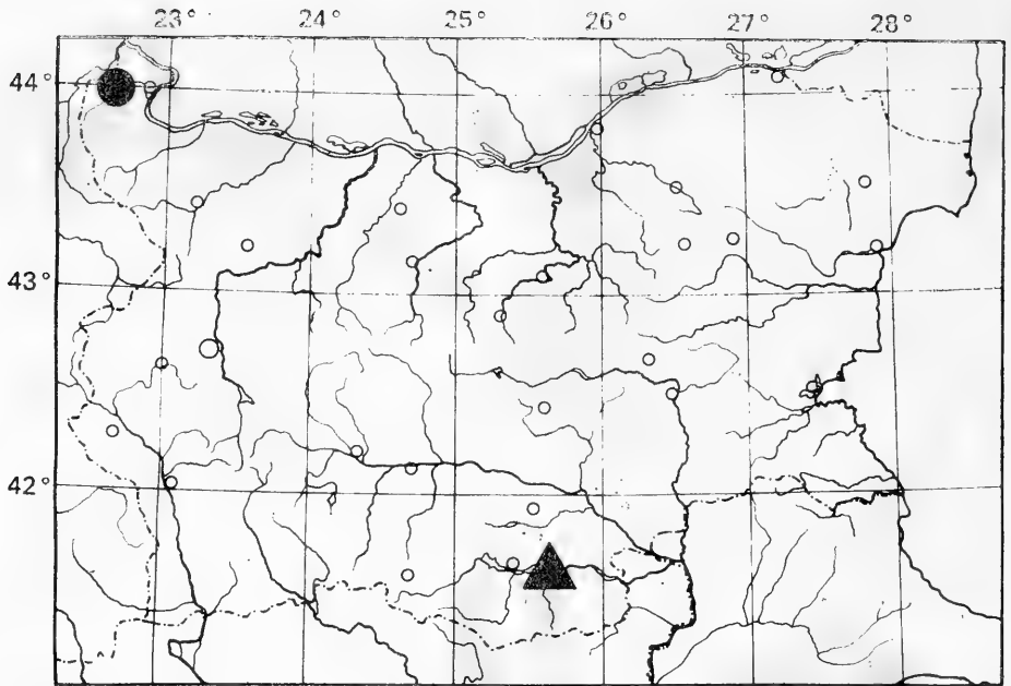
Фиг. 3. Разпространение в България на Potamophylax rotundipennis (Вгац.) (●) и Micropterna hatatilla М а l. (▲) (ориг.)
