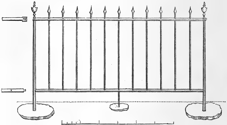
Fig. 333. Cast-iron Espalier-rail.
