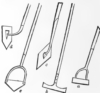
Fig. 23. Thrust-hoes.
