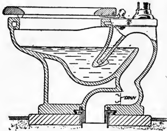
FIG. 20.—Flush closet.
