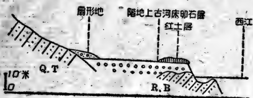
图10 西江谷地高要广利附近西江北岸20米卵石階地。
