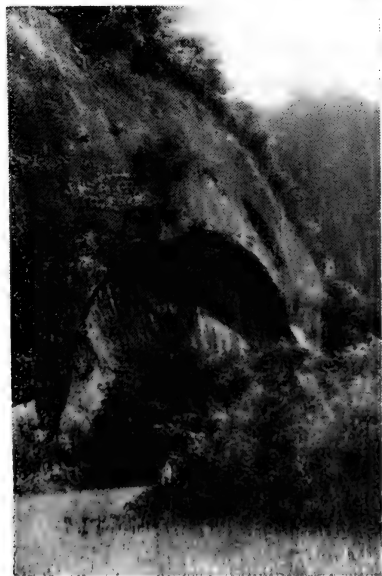
14 片狀剝落作用。
