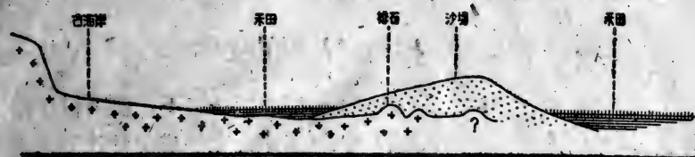
图4 銀沙乡沙堤基部有花崗岩排石，沙堤就在排石上堆积起来。
