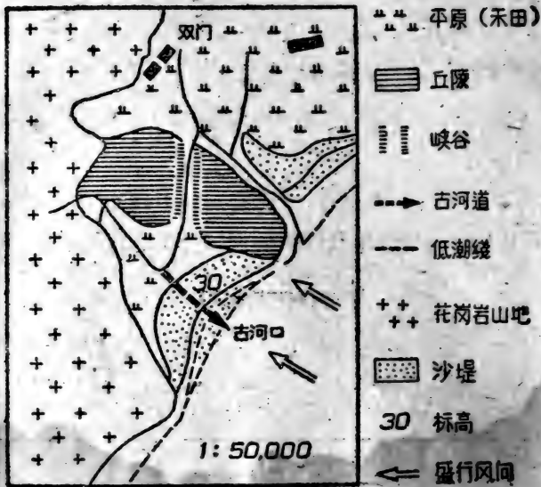
图23 广东广海海岸沙堤发育, 迫小河改流, 切过丘陵, 流入双门南方的小河。
