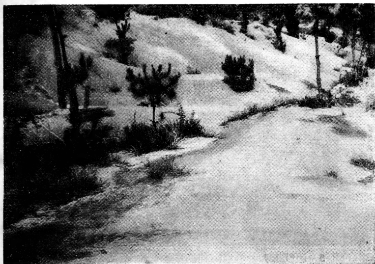
1 紅土瀉溜地形（注意圓滑形狀）。
