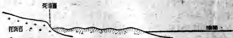
图17 沙堤堆叠成沙地,保护了海崖的状态。
