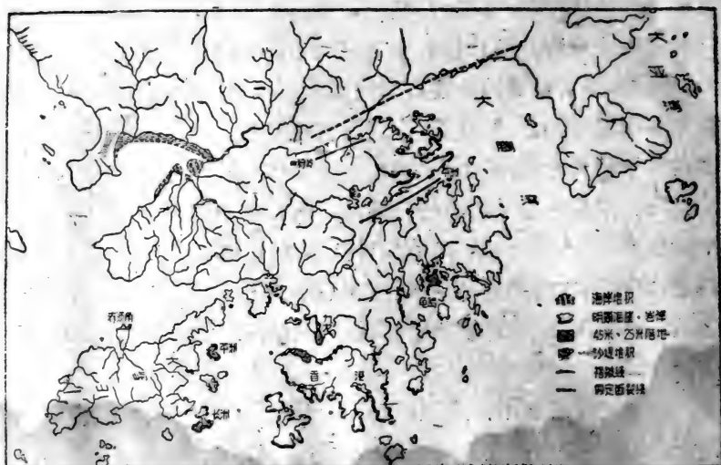
图19 香港、九龙深水山地海岸略图。
