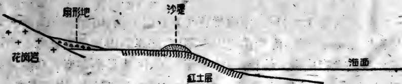
图16 沙堤移到扇形地的情形。
