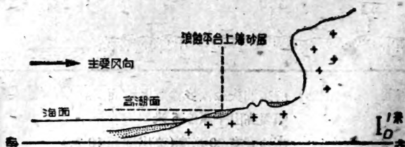
图27 广东广海附近花岗岩上海穴。
