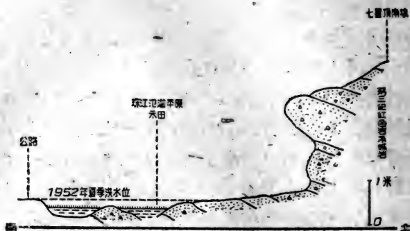
图12 广州东南郊七星顶山脚浪蚀平台。
