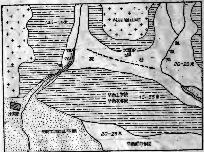
图11 广州市东北郊沙河切过45-55米階地掠夺長滙水。
