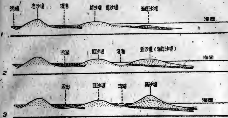
图7 低沙堤生成图。
