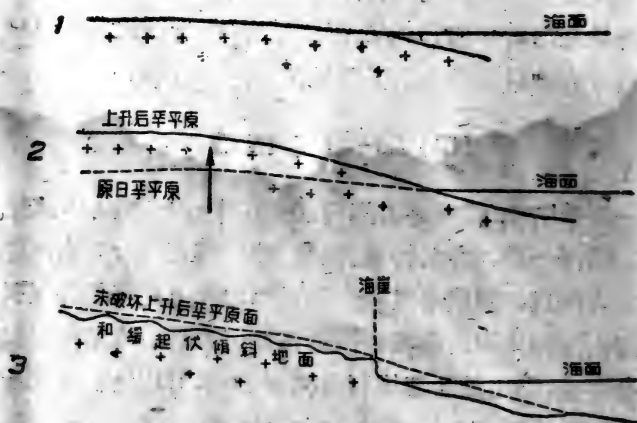
圖21 廈門附近傾斜准平原面的假說。
