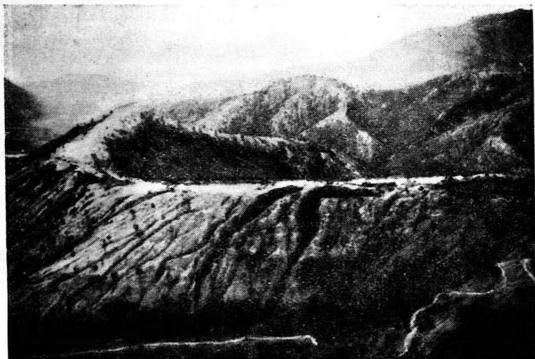
2 紅土溝地形（切溝）。
