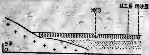
图9 广东番禺北郊太和市20米古平原(与20米階地同級)。
