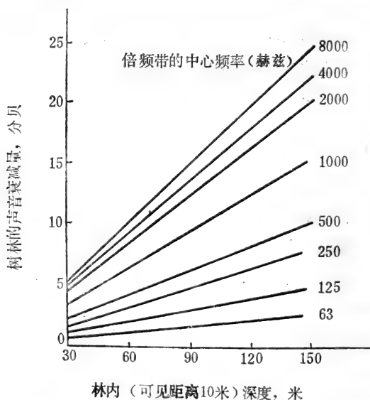
图6-8 树林内(可见距离10米)不同频率声音衰减量值变化
