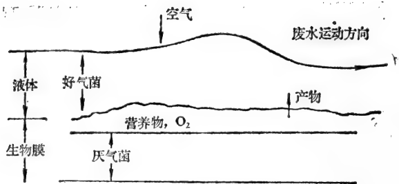
图6-5 生物滤池中的生物过程示意图
