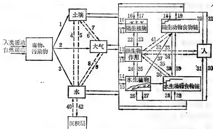
图5-1 毒物、污染物在生态系统中迁移、循环。1.废渣、风化。2.废气、挥发、蒸发、火山爆发、风暴等。3.废水、岩溶、灌溉、溶解、迁移。7,8挥发、蒸发、6,9沉降、冷凝。5.渗漏, 渗溶。4.灌溉。滴漏、排放。11,15,16,26,吸收、吸附。13.微生物吸附作用。18,19.吸收、食用、捕食。21,31,33,吸收、捕食、食用。22,25,32,35吸收。38,39捕食、食用。10,14,17,19,21,23,24,27,28,30,34,36,41分解、尸解。40.风化、岩溶等。42.沉积成岩。
