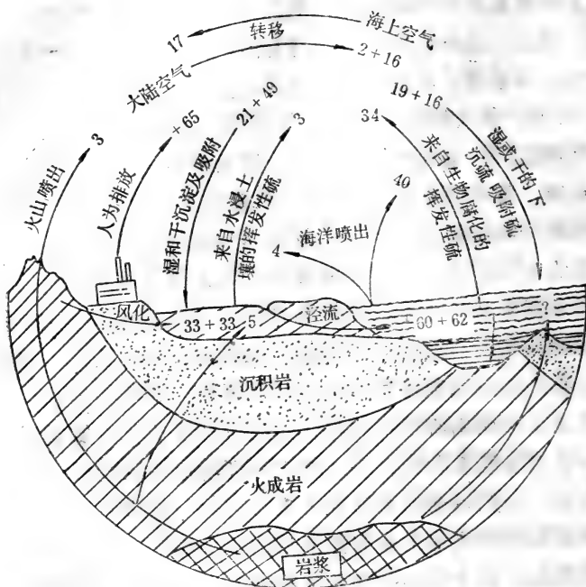
图2-6 全球的硫循环 (图中数字单位为 10^6 吨)
