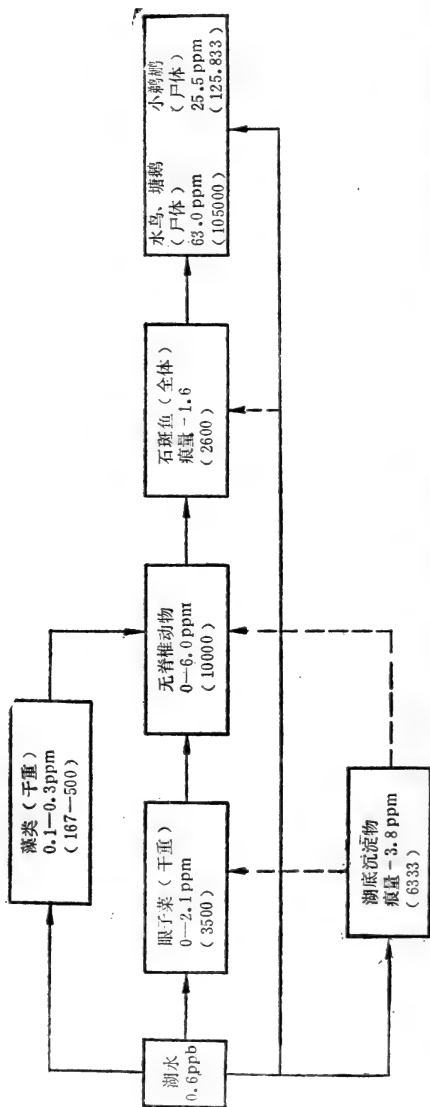
图5-11 美国加利福尼亚东北部明湖 (Tule) 和下克拉马斯 (Lower Klamath) 保护区中, DDT 依食物链富集传递情况。(图中括号内为浓缩系数, 痕量指含量为0.1ppm以下, 图中生物在湖里尸解后的 DDT 还可返回湖中与沉淀在湖底中。)
