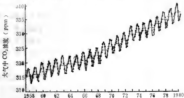
图7-1 夏威夷蒙娜罗亚大气中二氧化碳浓度的平均值
