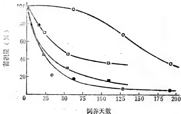
图5-10 喂金鱼DDT、狄氏剂，喂银大麻哈鱼多氯联苯后，它们在鱼体内的降解情况。○：DDT，●：狄氏剂，□：六氯联苯，■：四氯联苯(DItri1974)
