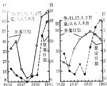
图7-4 日本大阪、东京的烟雾历年变化(宿稔等, 1972) 左: 大阪(大管浓烟雾); 右: 东京(东管浓烟雾)
