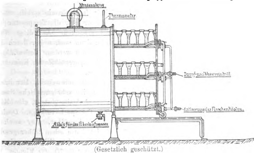
Milch-Pasteurisierungs- und Sterilisierungsapparat mit Rückkühlung.
