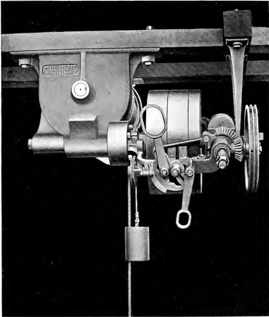
2000-LB. WORM HOISTING MACHINE.
