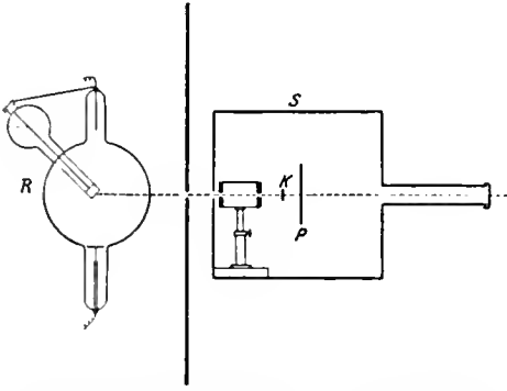
Durchleuchten eines Kristalls (K) mit Röntgenstrahlen.
