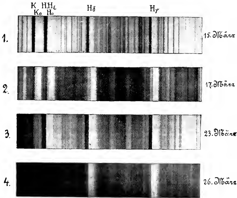
Spektra des neuen Sterns Nova Geminorum Nr. 2.
