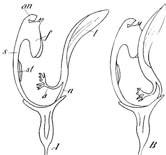
Pterostylis-Blüten nach dem Typus der Pt. curta . Helm und Unterlippe sind weggelassen. A mit ungereiztem, B mit gereiztem Labellum (l), s Säule, an Anthere, f flügelartige Anhängel der Säule, st Stigma, l Lippenplatte, n Nagel (Bewegungsorgan), a Anhängel des Labellums (Sinnesorgan). Nach Haberlandt.
