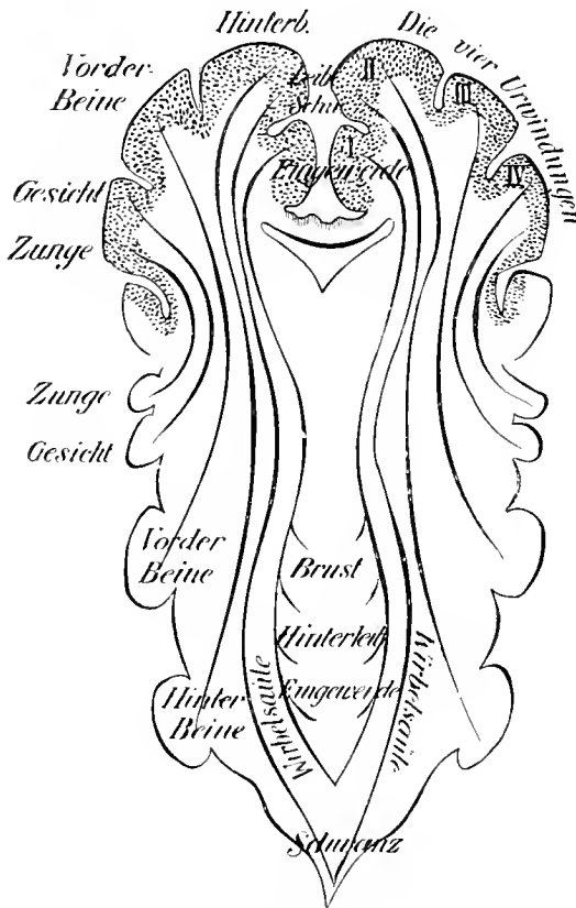
Projektion der Kumpfoberfläche auf die Hirnrinde. Schematisch, die Hirnrinde punktiert.
