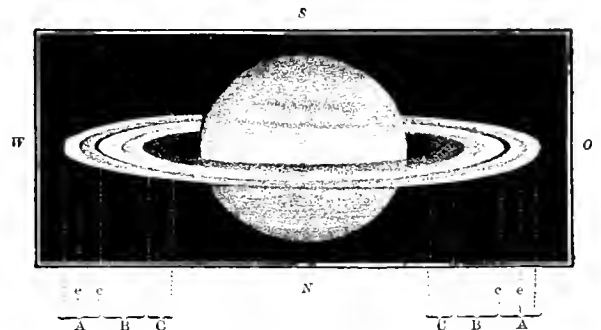
Bezeichnung der Saturnringe und der Trennungen.
