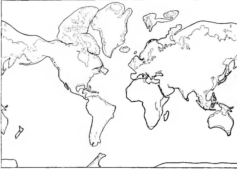
Skizze der einstigen Kontinental-schollen (fette Umrandung) bei Entstehung der Kontinente.
