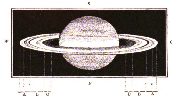
Bezeichnung der Saturnringe und der Trennungen. A = äußerer heller Ring, B = innerer heller Ring, C = dunkler oder Schleier-Ring. e = Endeische Trennung, e = Cassinische Trennung.
