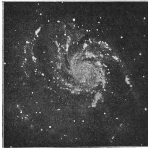
Photographie eines Spiralnebels im Großen Bären.
