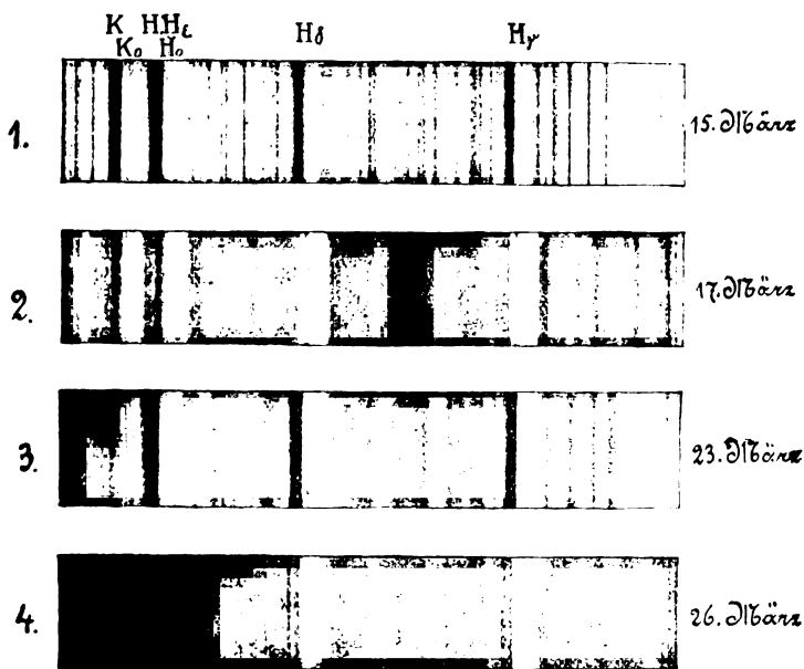
Spektra des neuen Sterns Nova Geminorum Nr. 2.
