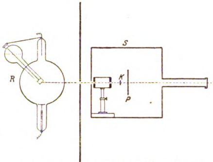
Durchleuchten eines Kristalls (K) mit Röntgenstrahlen.
