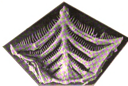
Coregonus fera Kiemenreue. (Nach Originalphotographien von Dr. A. Thienemann.)
