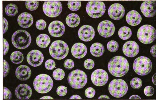
Flüssige Kristalle (Paraazoryanisol), welche mit Tusche vermischt waren, sondern sich von den Rußpartikelchen und drängen diese in die Zwischenräume.
