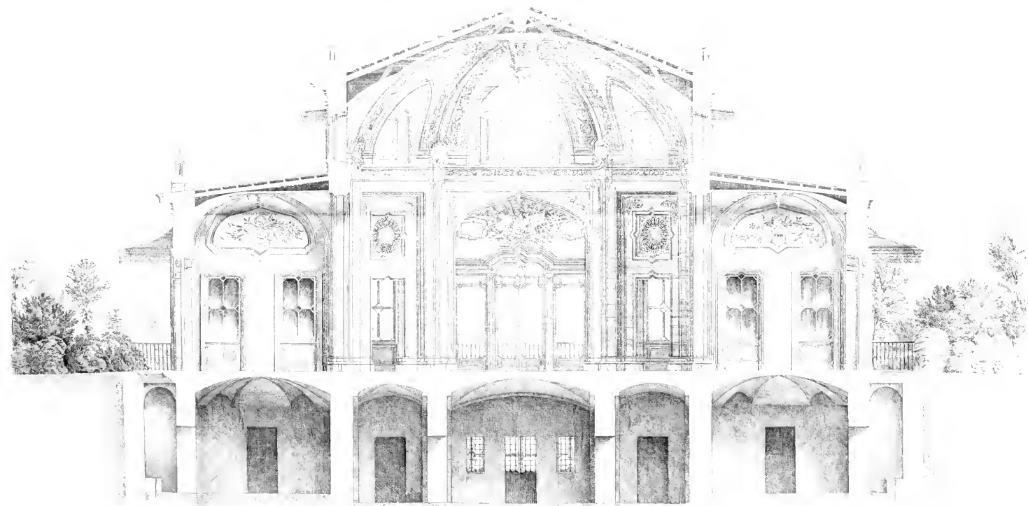
SEZIONE SULL'ASSE DI LEVANTE A PONENTE DEL SALONE ED ANNESSI DEL CAFFÈ COI SOTTOPOSTI LOCALI DI SERVIZIO
