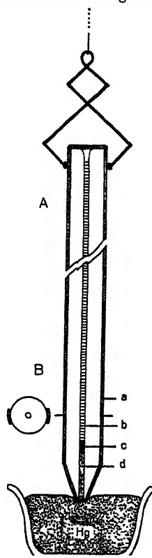
Abb. 1. A. Dosierröhrchen im Längsschnitt: a Gummiband, b Suspensionsflüssigkeit, c Mikroorganismensediment, d Eugenol. B. Dosierröhrchen im Querschnitt.
