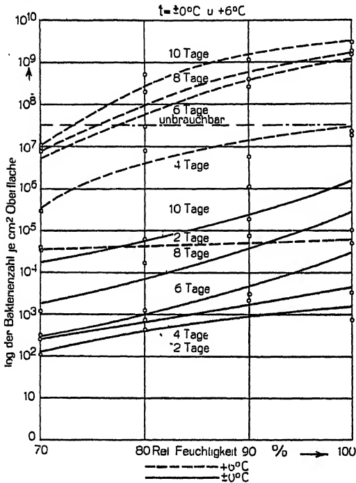
Abb. 2. Einfluß der Luftfeuchtigkeit auf das Bakterienwachstum bei verschiedenen Lagertemperaturen. F/G = 0,28; t = + 6 und ± 0° C.
