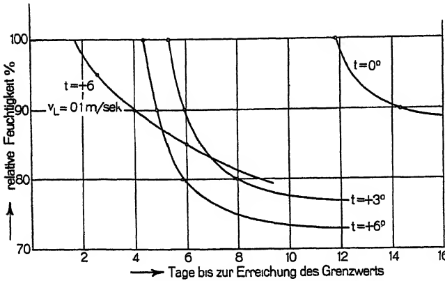
Abb. 7. Maximale Lagerdauer bei verschiedenen relativen Feuchtigkeiten und bei ruhender und bei bewegter Luft (Luftgeschwindigkeit: 0,1 m/sek.).
