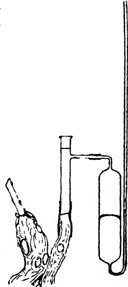
Fig. 27. Einrichtung zur Messung des Blutungsdruckes im Freien.
