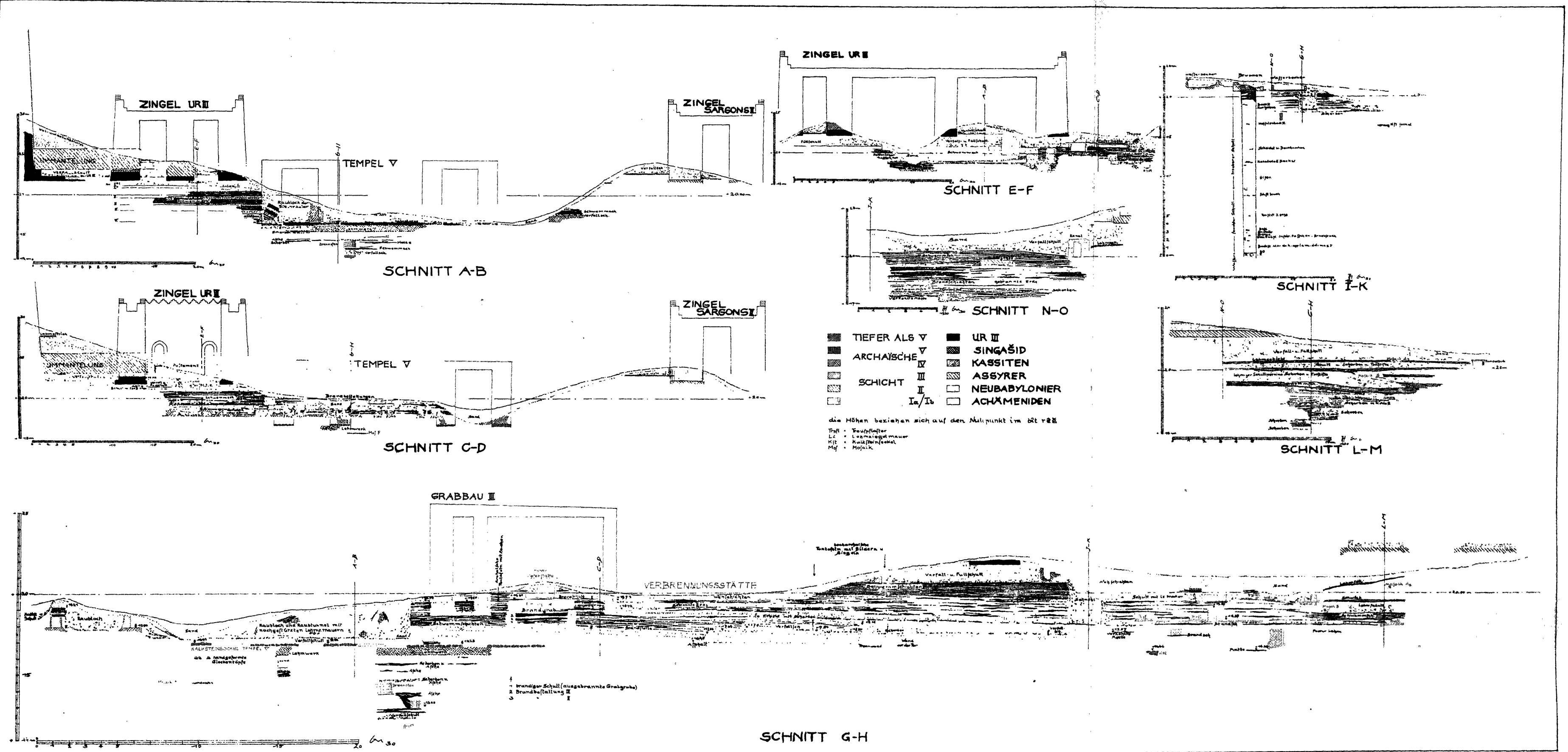
Eanna südöstlich der Zikurrat, Schnitte. J. JORDAN: Ausgrabungen in Uruk 1929/30. — Taf. 5.
