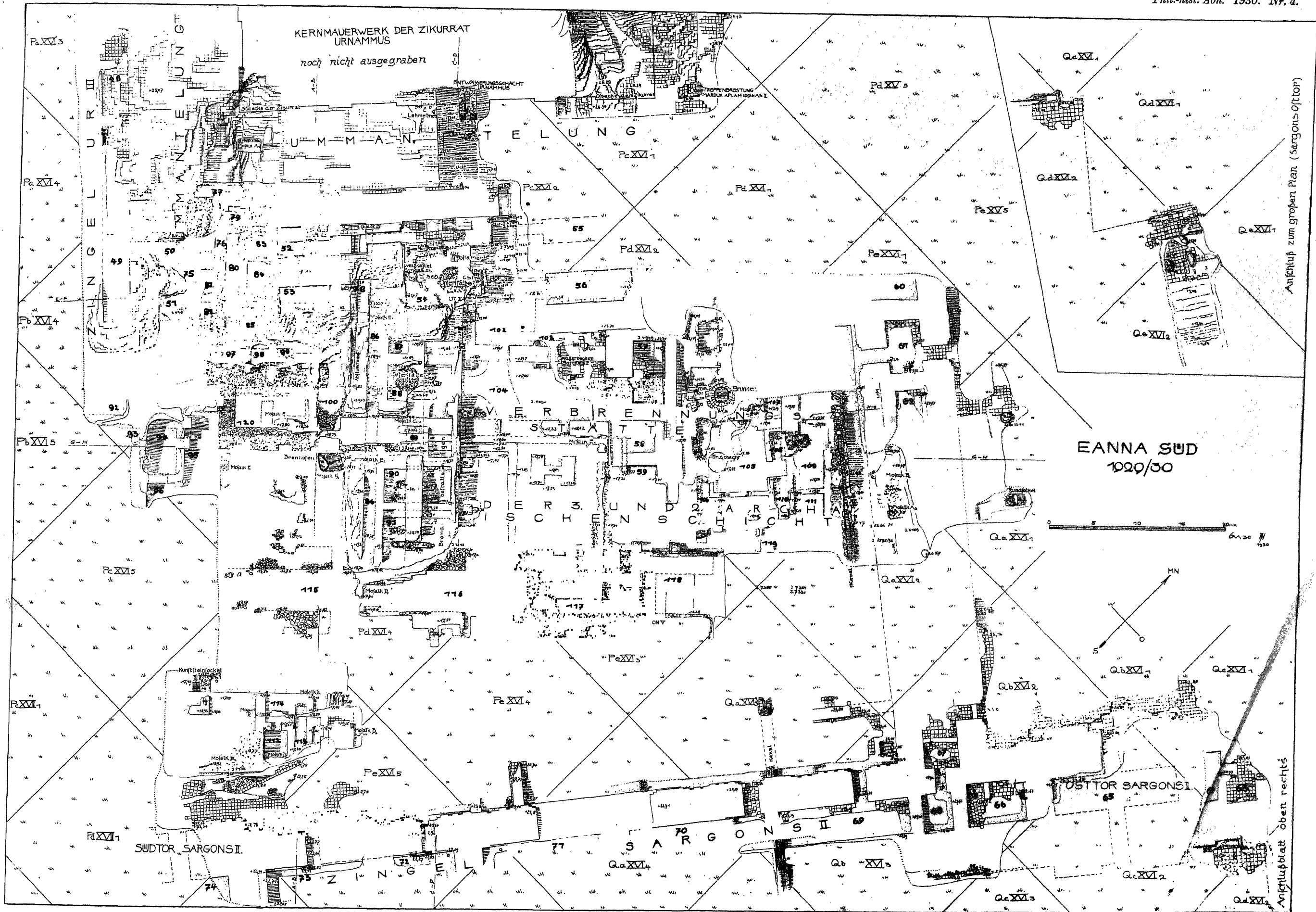
Eanna südöstlich der Zikkurat.
