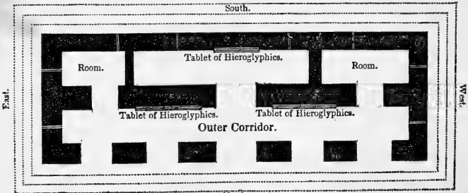
Plan of No. 1, Casas de Piedras, Palenque.
