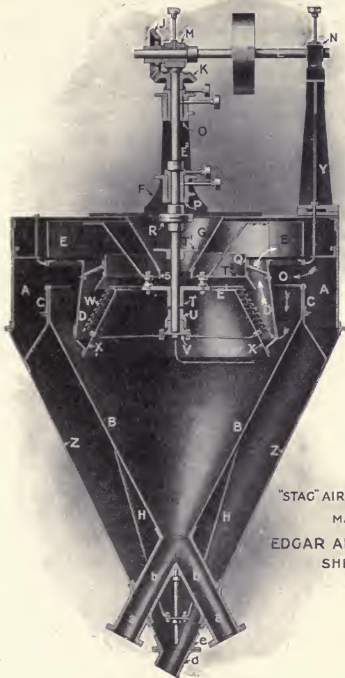
FIG. 34.—" STAG " AIR SEPARATOR.
