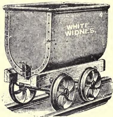
FIG. 146.—END-TIPPING WAGGON.
