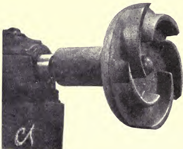
FIG. 168.—CERATHERM IMPELLER.
