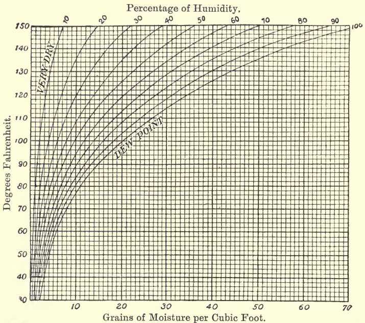
FIG. 80.—HYGROMETRIC CHART.
