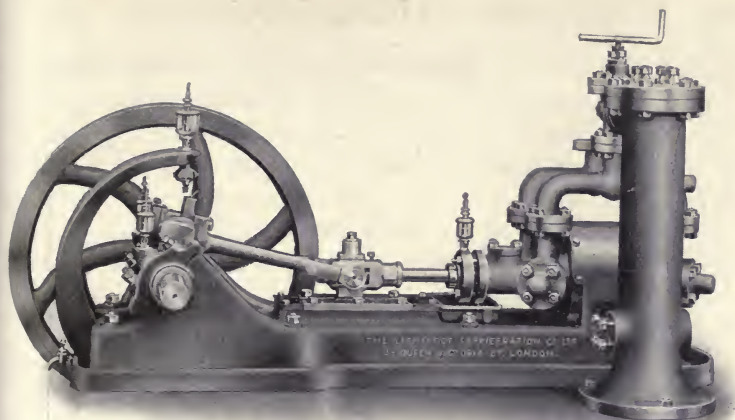
FIG. 143.—HORIZONTAL AMMONIA COMPRESSOR.
