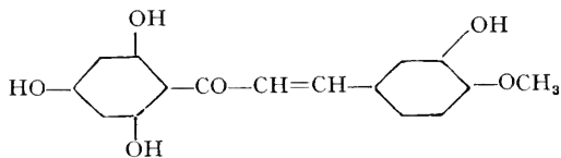
Hesperetin
