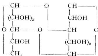
Amylose [(C_6H_{10}O_5)_2]_n
