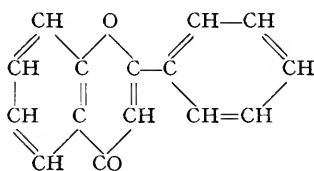
Flavone
