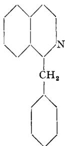
Papaverine
