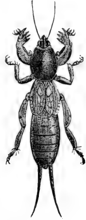
FIG. 108. — Gryllotalpa borealis .
