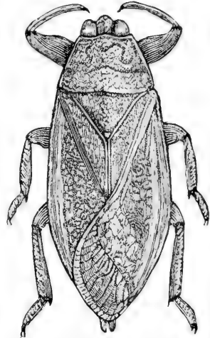
FIG. 159.— Belostoma americanum .
