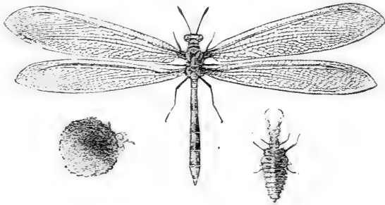
FIG. 193.— Myrmelcon .
