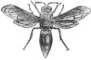
FIG. 2.— Monobia .
