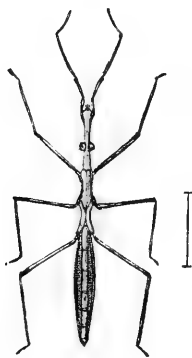
FIG. 165.— Limnobates lineata .
