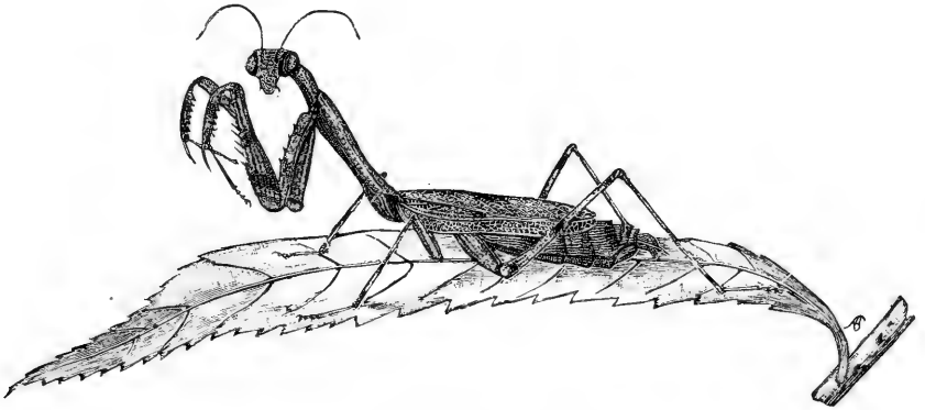
FIG. 89.— Phasmomantis carolina.
