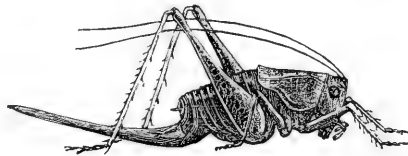
FIG. 106.— Thyreonotus .
