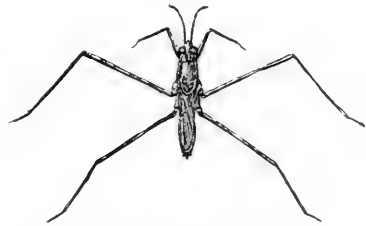
FIG. 164.— Hygrotrechus conformis .
