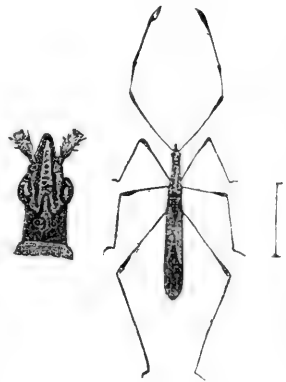
FIG. 181.— Jällysus spinösus .
