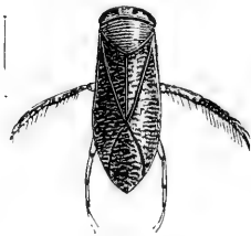
FIG. 156.— Corisa undulata .
