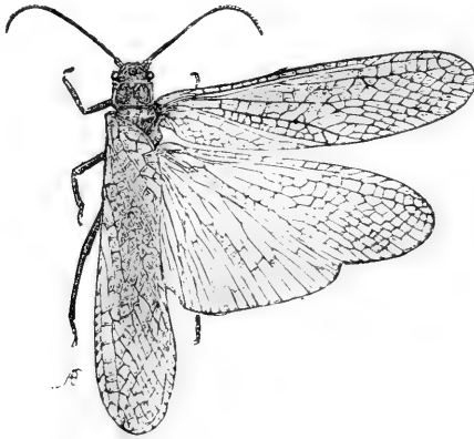
FIG. 72.— Pteronarcys regalis .
