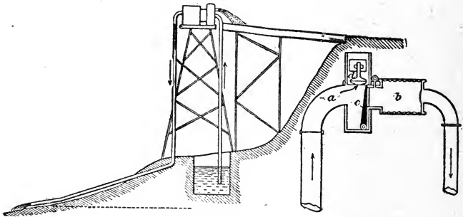
Fig. 70. Siphon elevator. (Wilson, U. S. Geol. Survey.)
