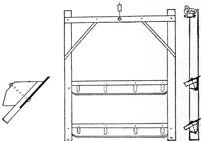
Fig. 91. Simple land grader.
