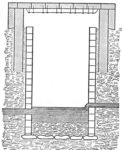
Fig. 140. Silt basin.
