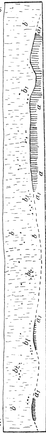
Fig. 1. Profil an der Nordwand der Ziegelei-grube von Kilian & Cie. am Südaabhäng des Gräselberges in 110-115 m über N. N. Maßstab 1:250.
