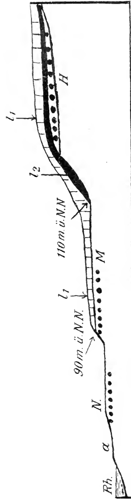
Fig. 3. Idealschema für die Beziehungen von älterem und jüngerem Löss am Südrand des Taunus zu den drei jüngsten Diluvialterrasse.
