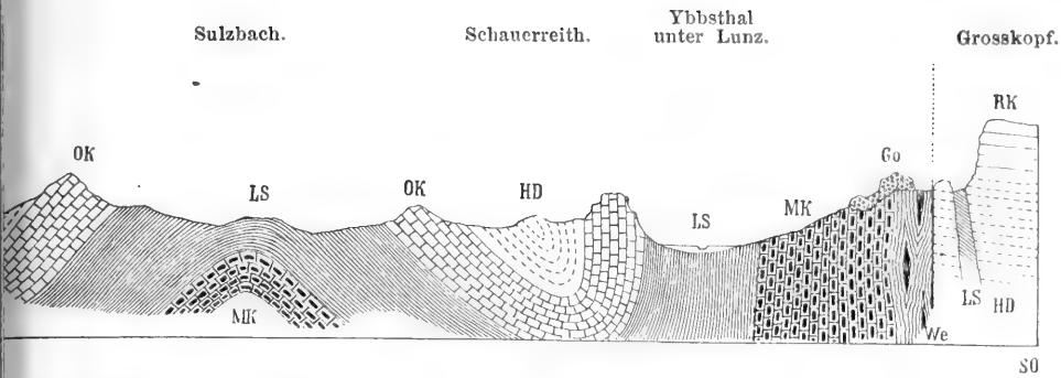
1. Profil durch die Gegend von Lunz nach den Aufnahmen von A. Bittner.
