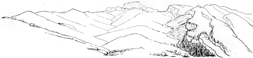
Grenze des Flyschgebietes nördlich von Sarajevo gegen das Triasgebirge. Vom Narodno brdo aus.
