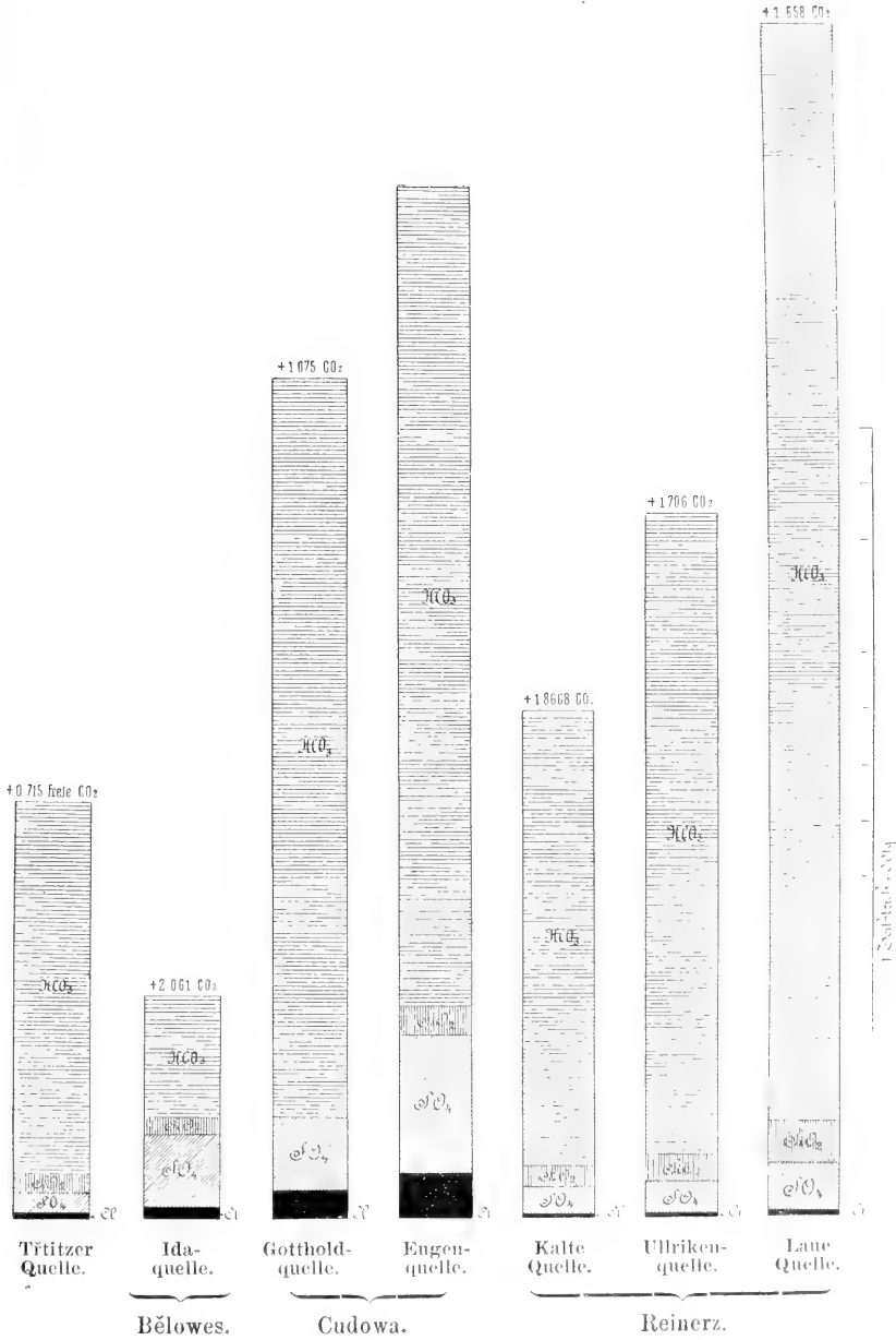
Fig. 2. Säure Jonen.
