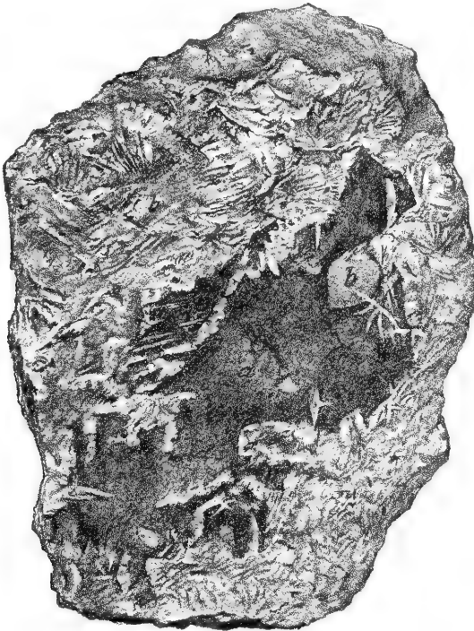
a = Dolomit. — b = Magnesit.
