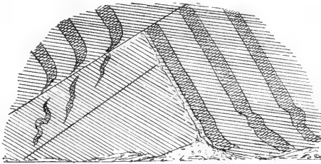
Falsche Schieferung und Verwürfe der Karbouschiefer bei Lugovi.
